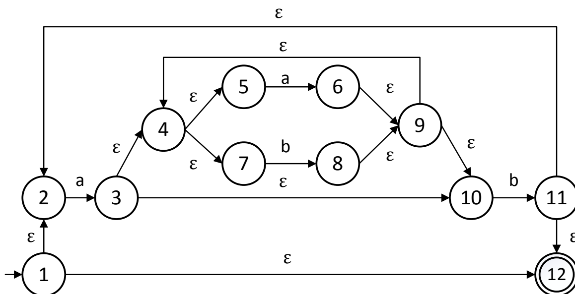
Рис. 3.10 НКА с \epsilon -переходами для регулярного выражения (a(a|b)^*b)^*
