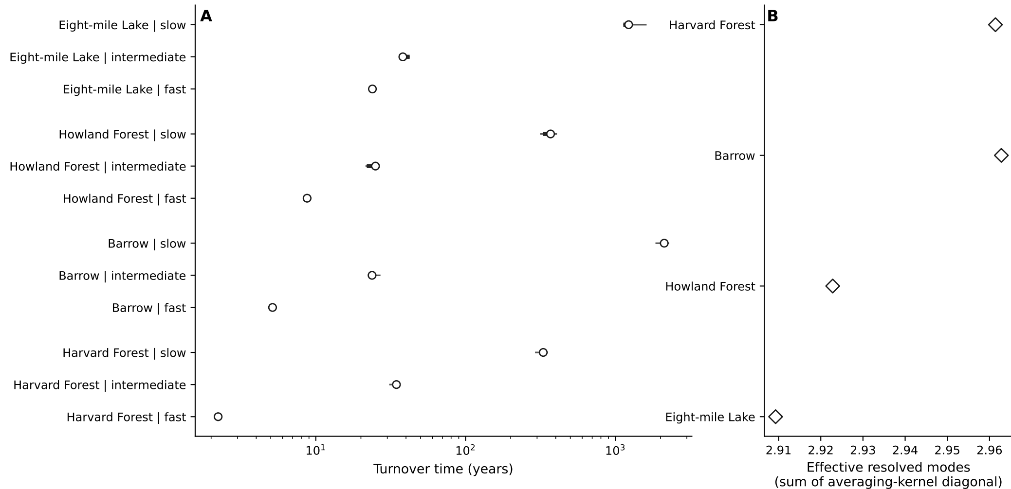
Posterior Turnover-Time Distributions
