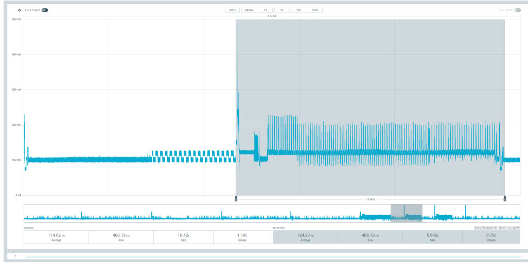
Abbildung 10: Stromverlauf – BLE-Phase gesamt (Ausgangslage)
