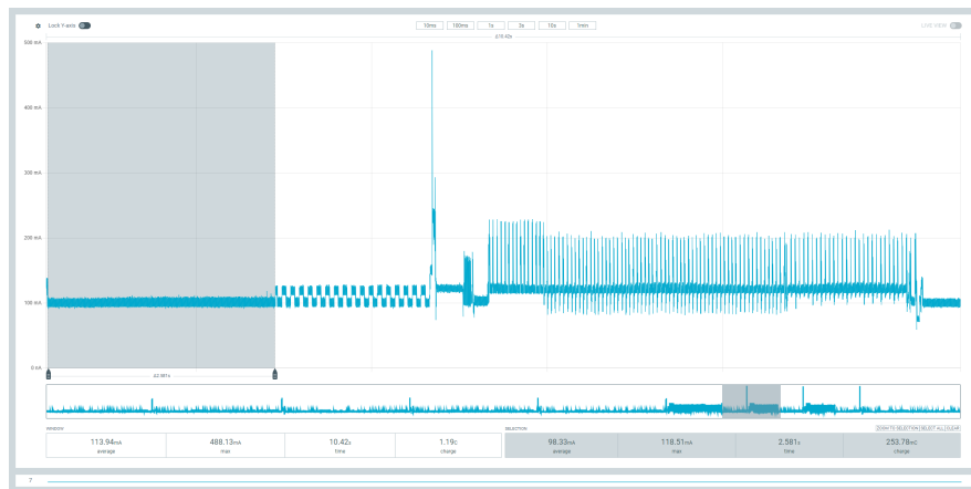
Abbildung 3: Stromverlauf – Boot & Initialisierung (Ausgangslage)
