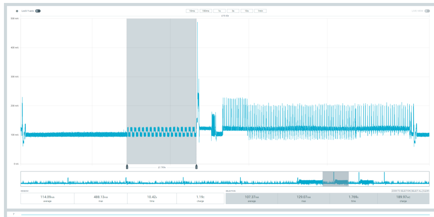
Abbildung 4: Stromverlauf – ADC-Messung (Ausgangslage)
