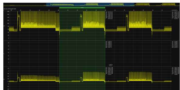
Abbildung 31: Nach LDO (3V3-Pin) – Ausgangslage; 2220 mJ
