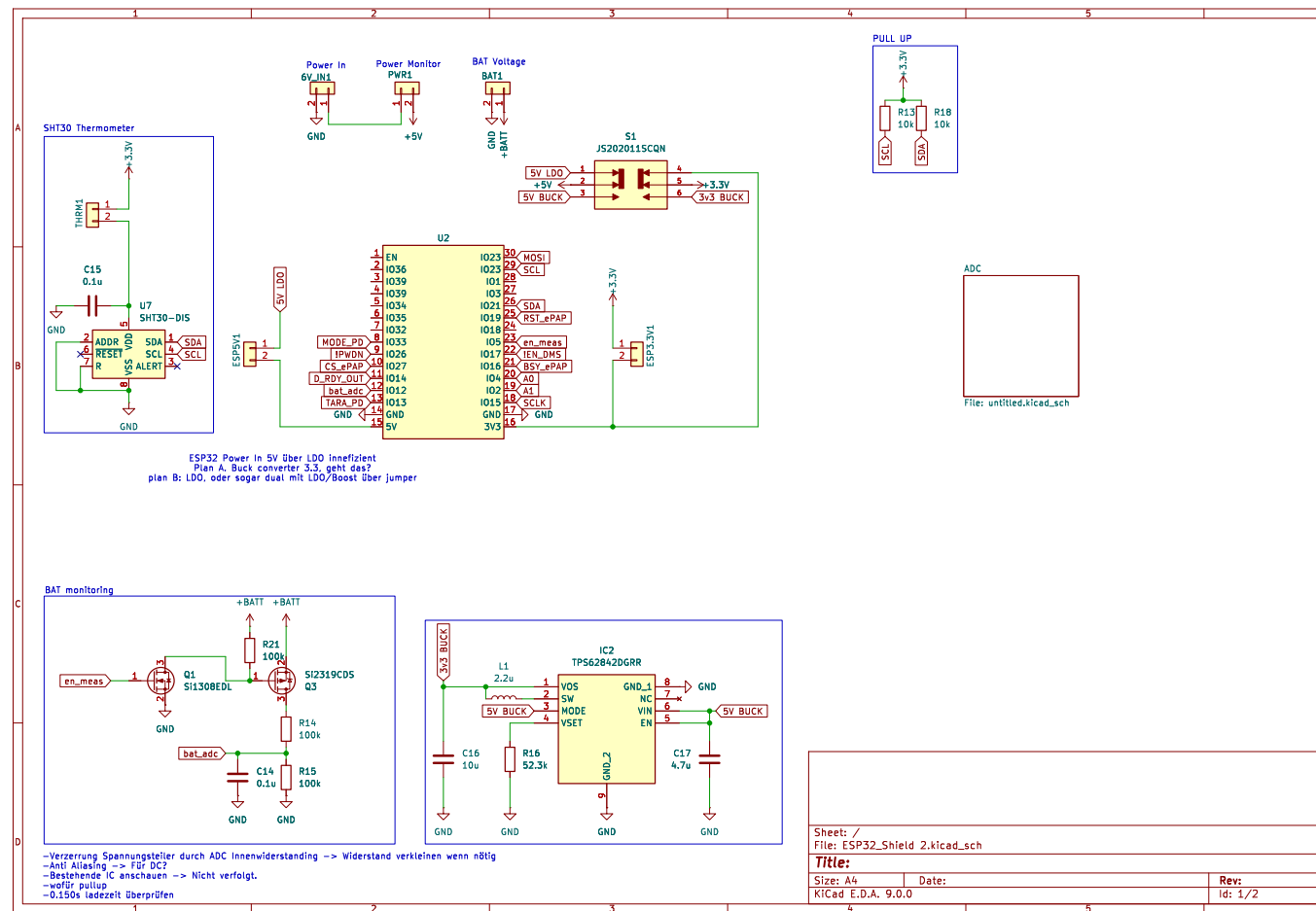
Abbildung 33: PCB Schaltplan – Seite 1
