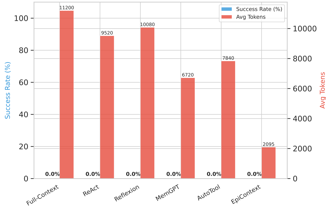
WEBARENA
