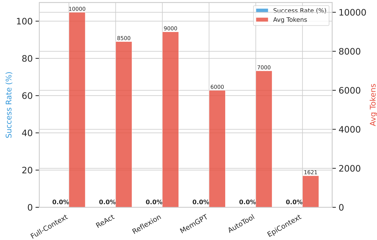
ALFWORLD
