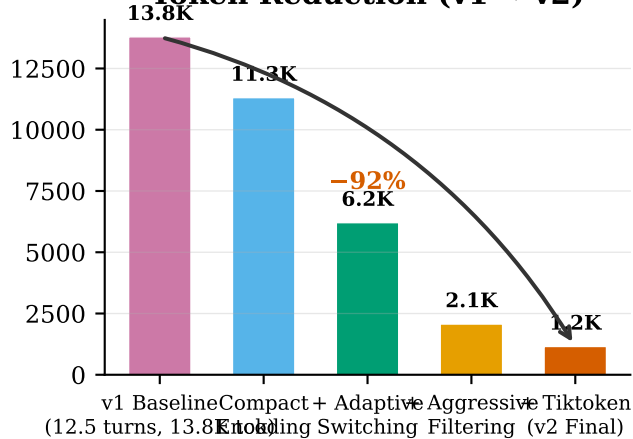
Token Reduction (v1 → v2)
