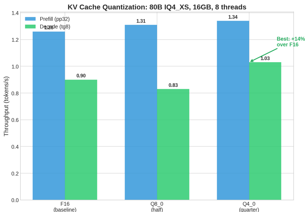
图 4: KV Cache 量化类型对比 (F16 vs Q8_0 vs Q4_0)
