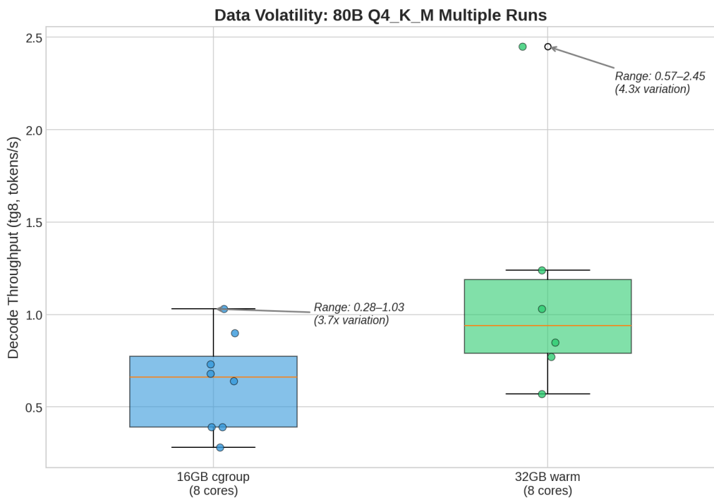
图 3: 80B 模型多次测量的数据波动分布（箱线图 + 散点）
