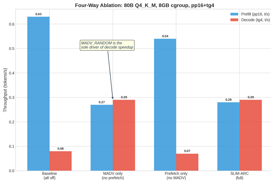
图 2: 四组单点消融实验结果对比
