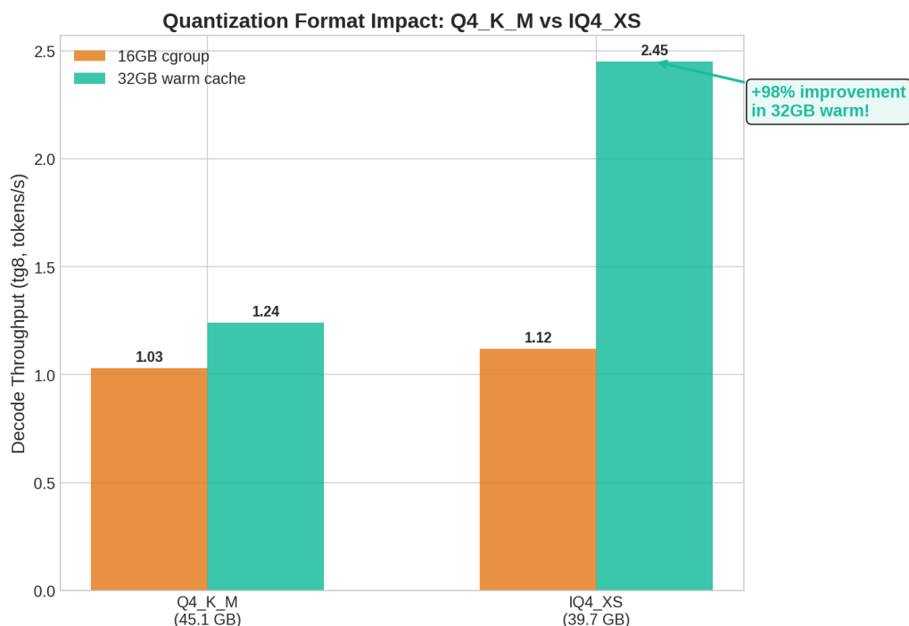
图 7: Q4_K_M vs IQ4_XS 量化格式性能对比
