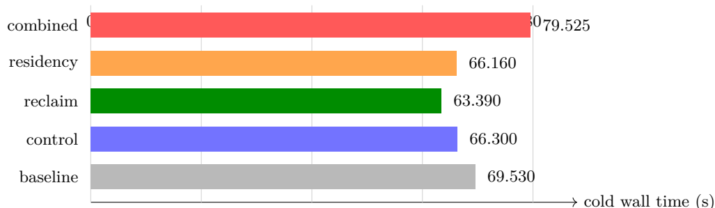
图 2: 固定 2 GiB 协议下的 cold wall time。数值由 hash 绑定的正式 JSON 宏生成；该图用于展示配置排序和组合回退，不表示跨设备加速比。
