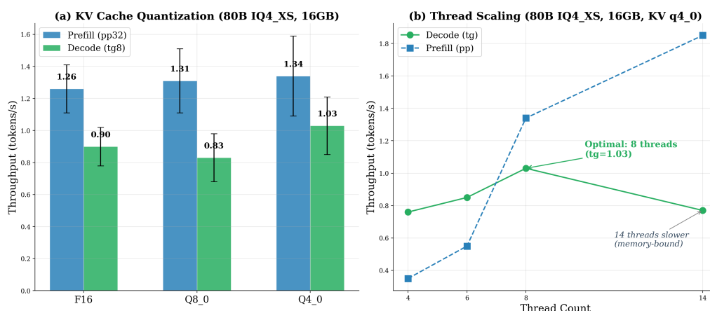
图 8: (a) KV Cache 量化类型对比 (带误差棒)。Q4_0 在 decode 阶段显著优于 F16 和 Q8_0，因为 0.5× 内存占用为权重缓存腾出更多空间。(b) 线程数扩展性分析。8 线程最优，超过 8 线程后由于 memory-bound 特性无额外收益。
