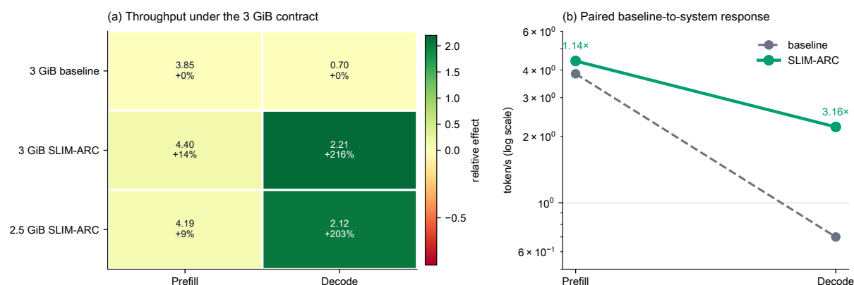
图 9: RK3588 3 GiB cgroup 的归一化性能温度图与配对响应图。左图同时编码绝对吞吐和同档增益, 右图在对数轴上显示 baseline 到 SLIM-ARC 的 Prefill/Decode 迁移。
