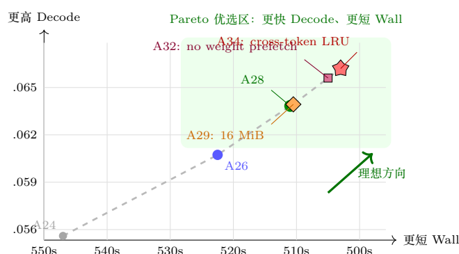
图 12: Raspberry Pi 5 的 Decode-Wall 多目标 Pareto 图。预算收缩、关闭无收益预取和跨 token LRU 依次把运行点推向右上角。
