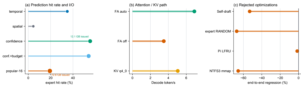
图 14: 消融实验多指标总览。左: 专家预测命中与投机 I/O 的联合代价; 中: FlashAttention 与 KV 量化对 ARM Decode 的影响; 右: 由端到端指标否决的优化。图中只连接同一实验合同内可比较的数据。
