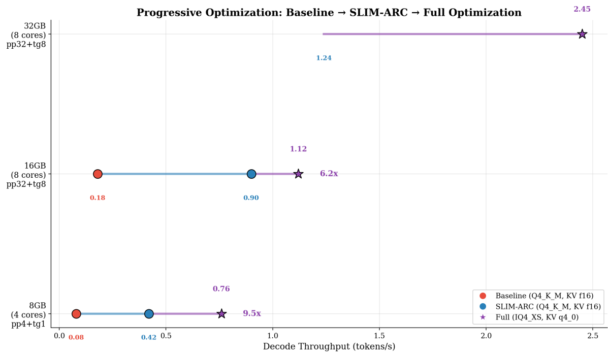
图 4: 优化技术渐进提升：从 baseline 到 IQ4_XS + KV q4_0 + eviction 的完整优化链
