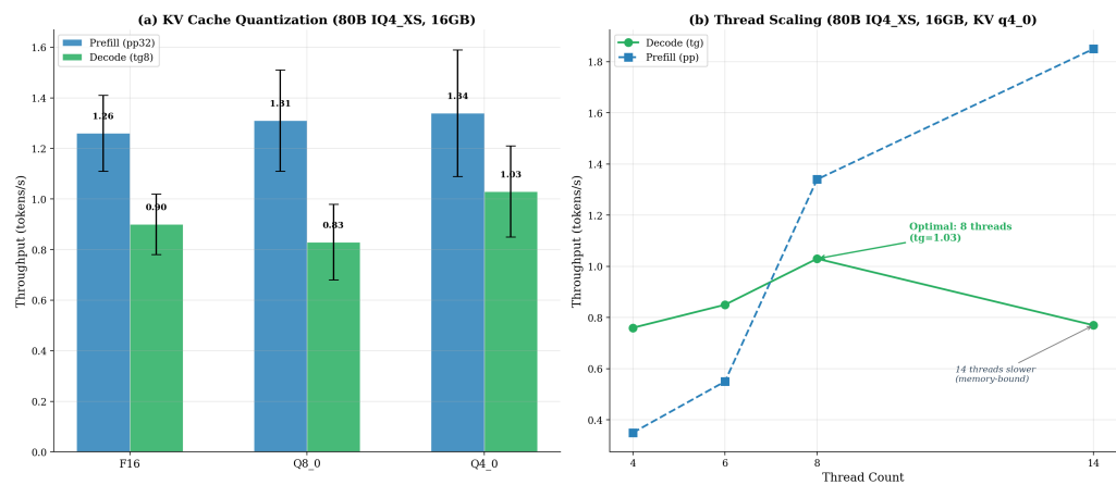
图 5: (a) KV Cache 量化类型对比 (带误差棒) (b) 线程数扩展性分析
