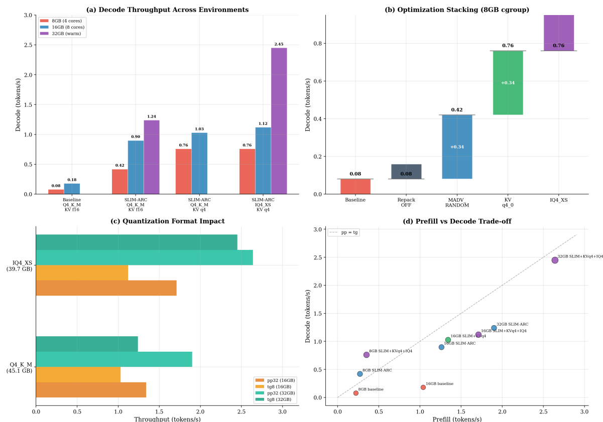
图 1: SLIM-ARC 性能全景: (a) 三档环境 decode 对比, (b) 优化堆叠瀑布图, (c) 量化格式对比, (d) prefill vs decode 权衡
