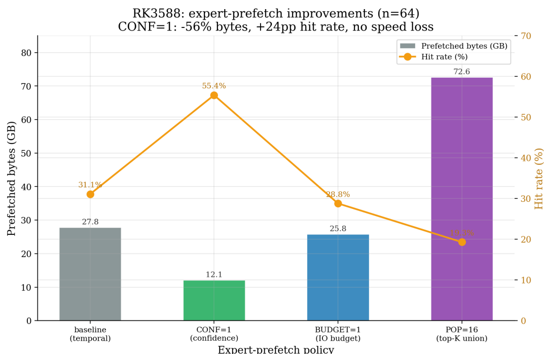
图 16: RK3588 专家预取改进对比。置信度门控 (CONF=1) 将预取字节从 27.8 GB 降至 12.1 GB (-56%)、命中率从 31.1% 提升至 55.4%(+24 个百分点)且解码速度无损;统一 I/O 预算(BUDGET=1)机制正确但端侧非 I/O 受限、收益有限;热门专家并集 (POP=16) 为诚实负结果 (默认关闭)。
