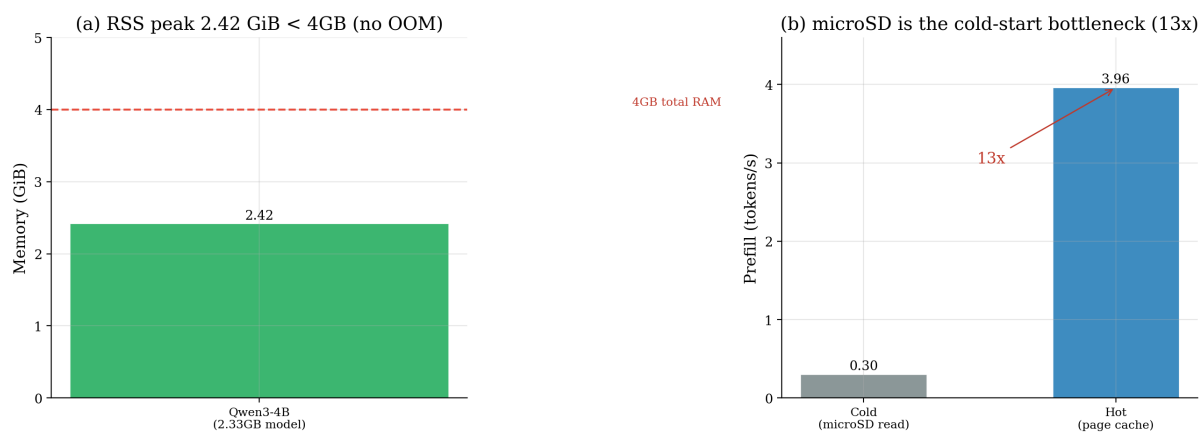
图 19: Pi5 (4GB) 内存占用与存储瓶颈。(a) Qwen3-4B 推理 RSS 峰值 2.42 GiB (小于 4 GB, 未 OOM); (b) 冷启动 prefill 0.3 t/s vs 热缓存 3.96 t/s (约 13 \times ), microSD 是冷启动最大瓶颈。
