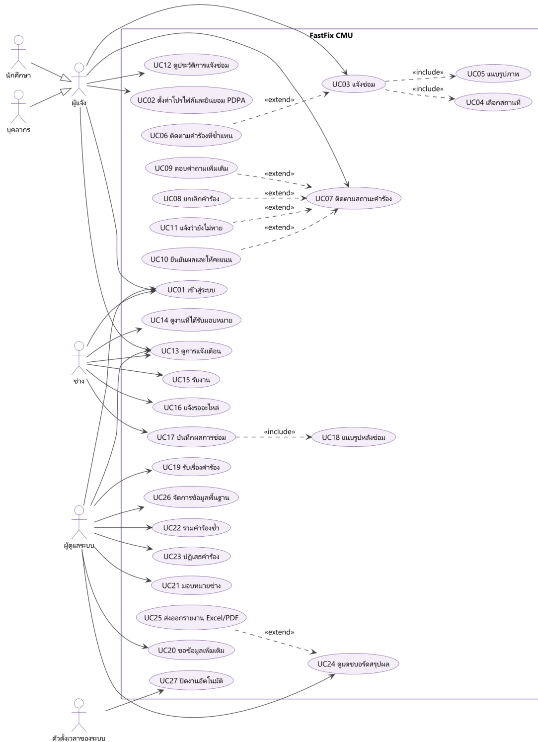
ภาพที่ 4.1 แผนภาพยูสเคสของระบบ FastFix CMU
