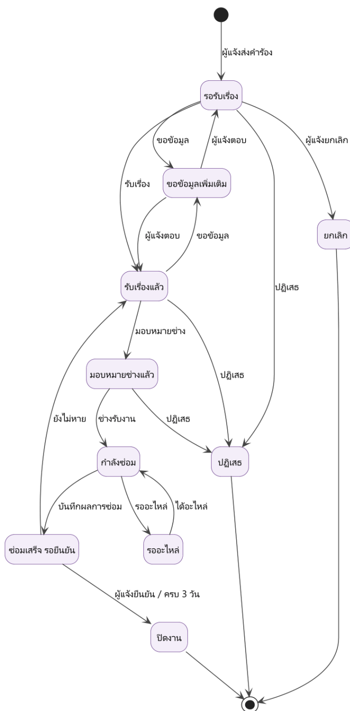
ภาพที่ 5.6 แผนภาพสถานะของคำร้องแจ้งซ่อม
