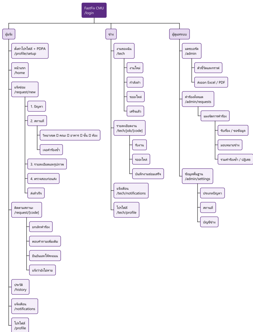
ภาพที่ 6.1 แผนผังเว็บไซต์ของระบบ FastFix CMU
