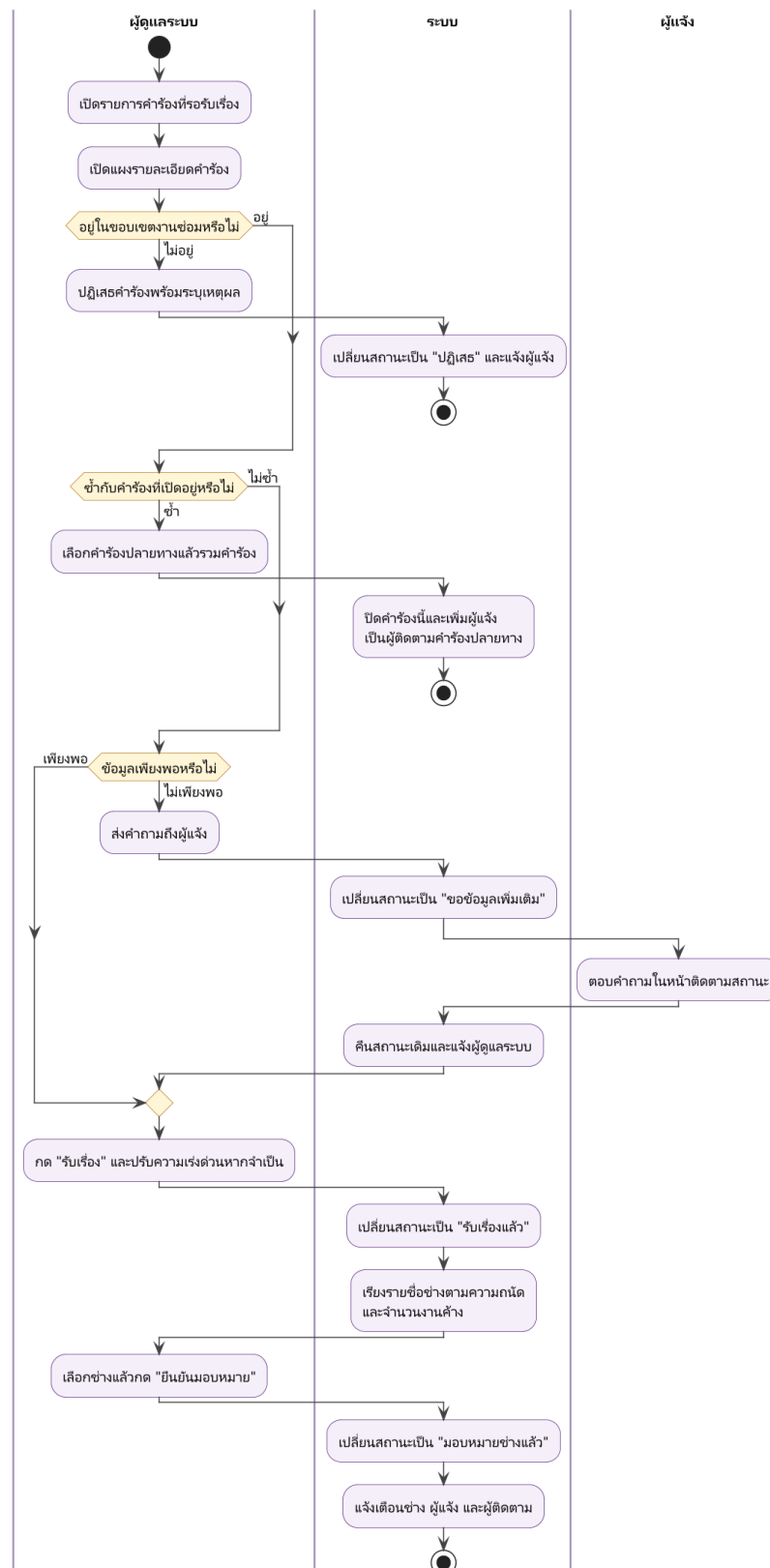
ภาพที่ 5.5 แผนภาพกิจกรรมการคัดกรองคำร้องและมอบหมายข้าง
