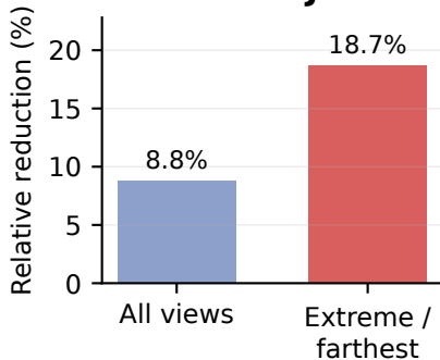
WA-MPJPE
