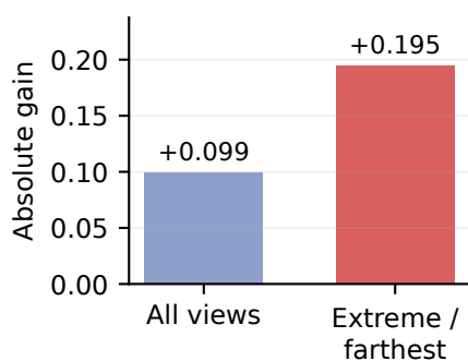
IDF1
