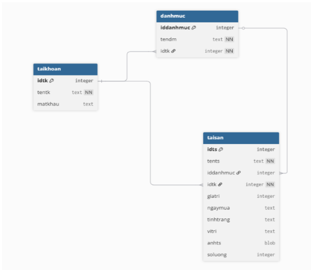
Hình 3. Thiết kế cơ sở dữ liệu mức vật lý
