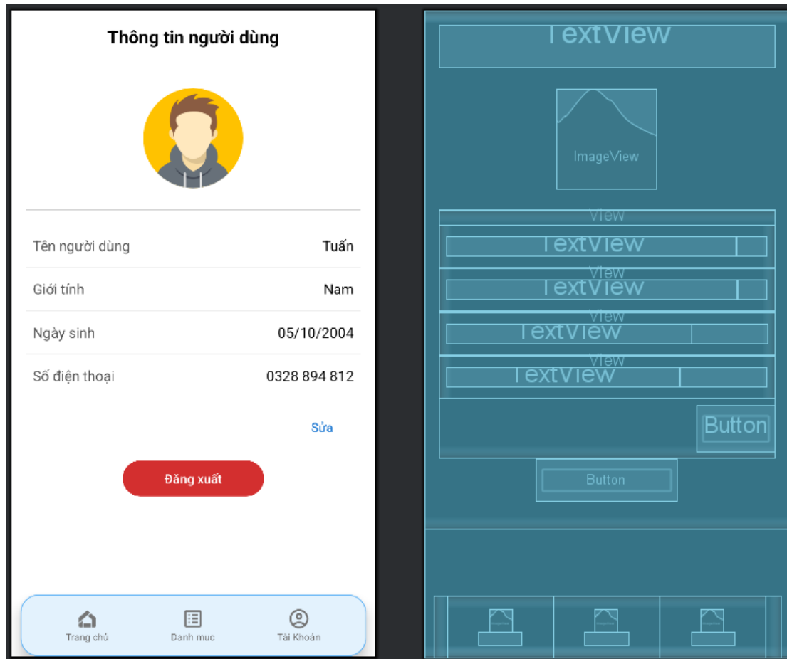
Hình 11. Màn hình android thông tin người dùng
