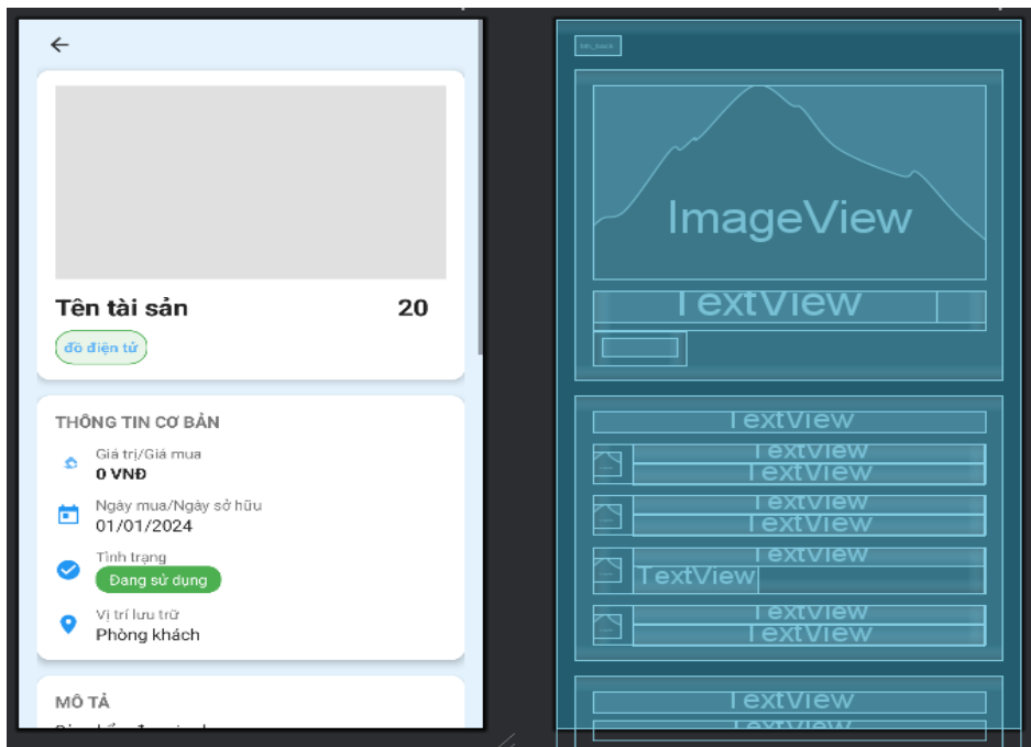
Hình 25. Màn hình android xem chi tiết tài sản
