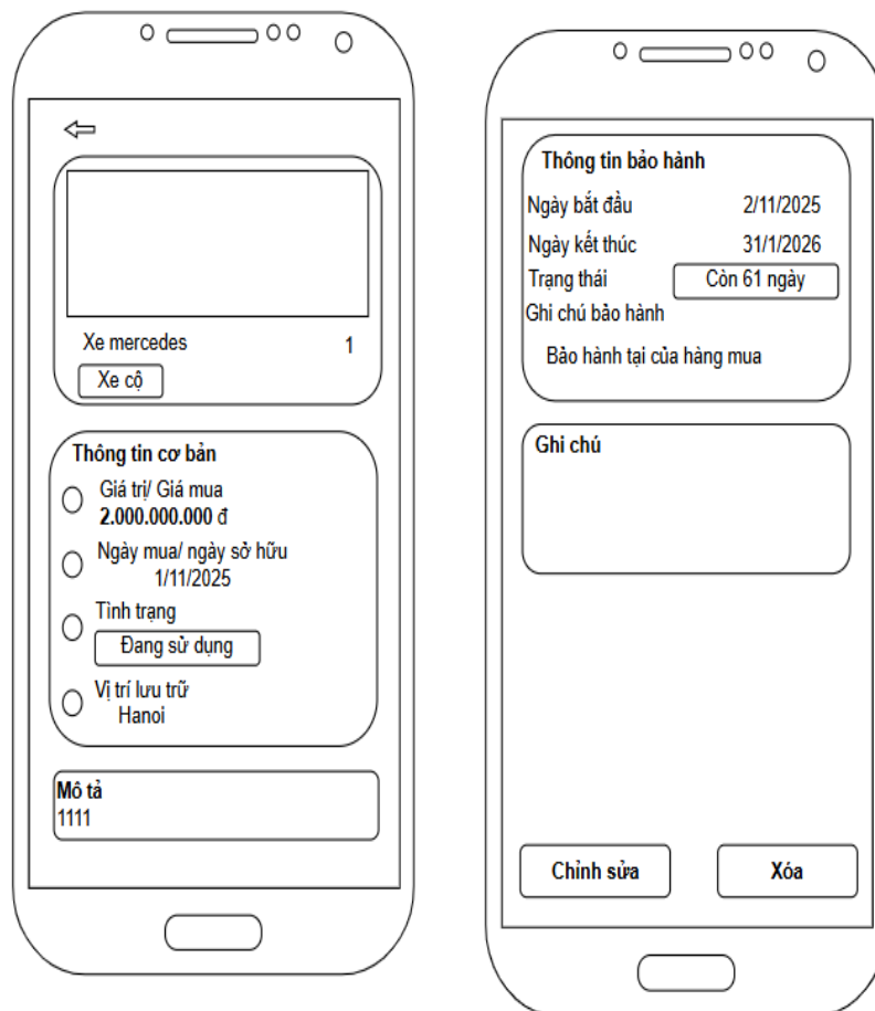
Hình 24. Hình dung màn hình xem chi tiết tài sản
