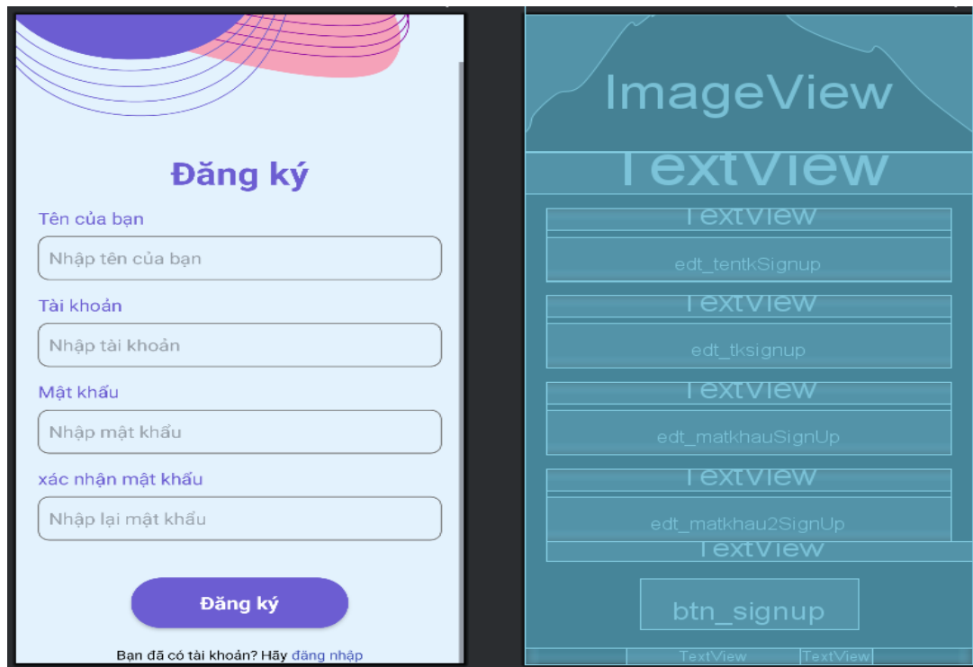
Hình 8. Màn hình android đăng ký
