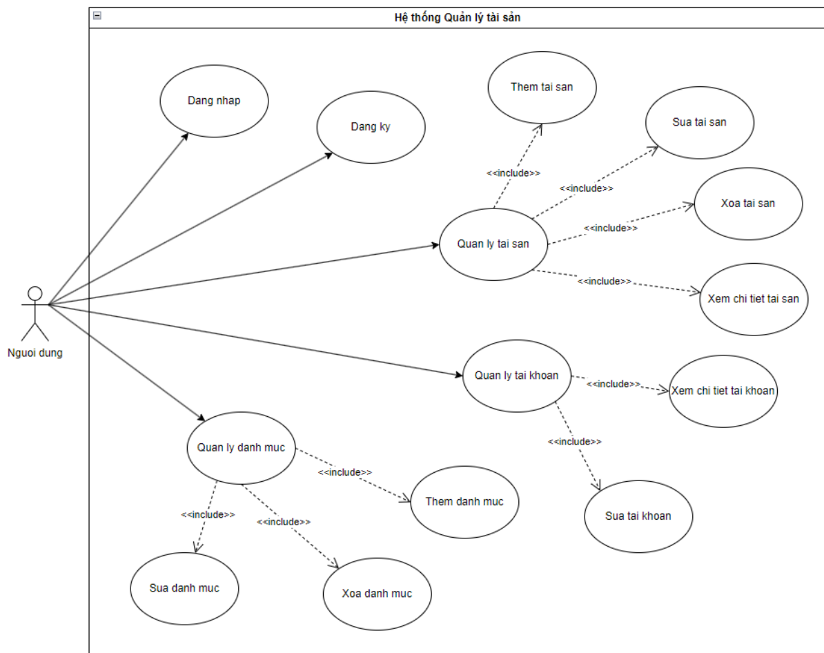
Hình 2. Biểu đồ quan hệ giữa các use case
