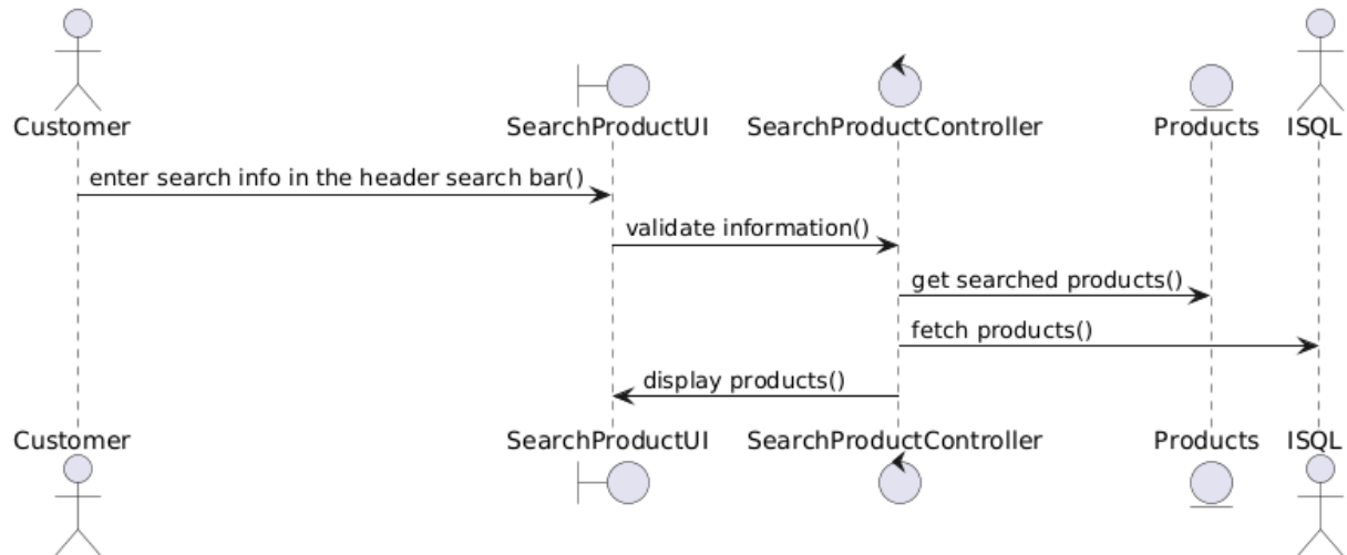
Hình 2.24: Biểu đồ trình tự chức năng tìm kiếm
