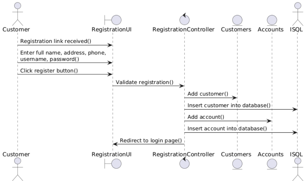
Hình 2.8: Biểu đồ trình tự chức năng đăng ký
