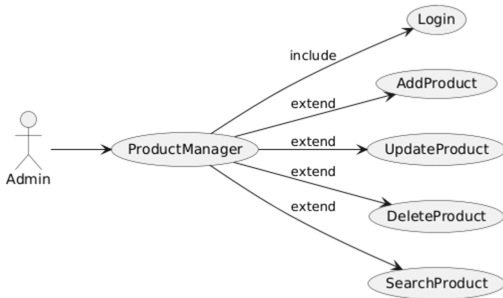
Hình 2.5: Use case quản lý sản phẩm
