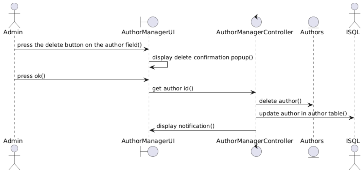
Hình 2.14: Biểu đồ trình tự chức năng xoá tác giả
