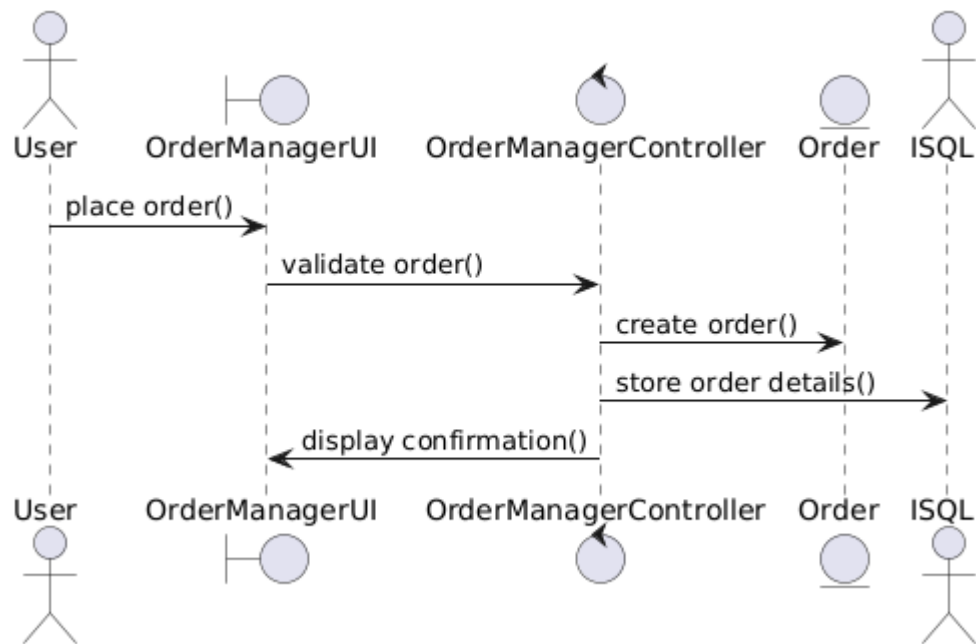
Hình 2.21: Biểu đồ trình tự chức năng quản lý đơn hàng
