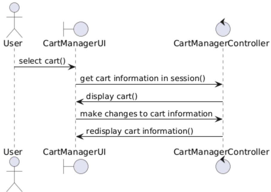
Hình 2.22: Biểu đồ trình tự chức năng quản lý giỏ hàng
