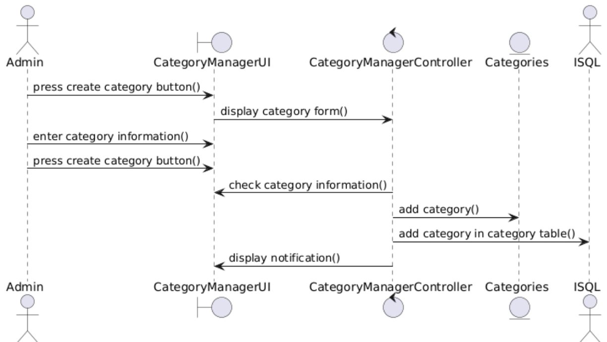
Hình 2.10: Biểu đồ trình tự chức năng thêm mới danh mục
