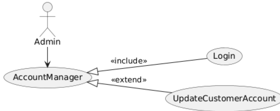
Hình 2.7: Use case quản lý khách hàng
