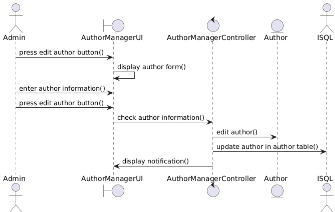
Hình 2.13: Biểu đồ trình tự chức năng cập nhật tác giả
