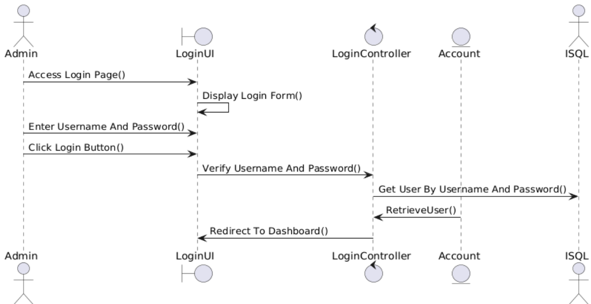
Hình 2.9: Biểu đồ trình tự chức năng đăng nhập
