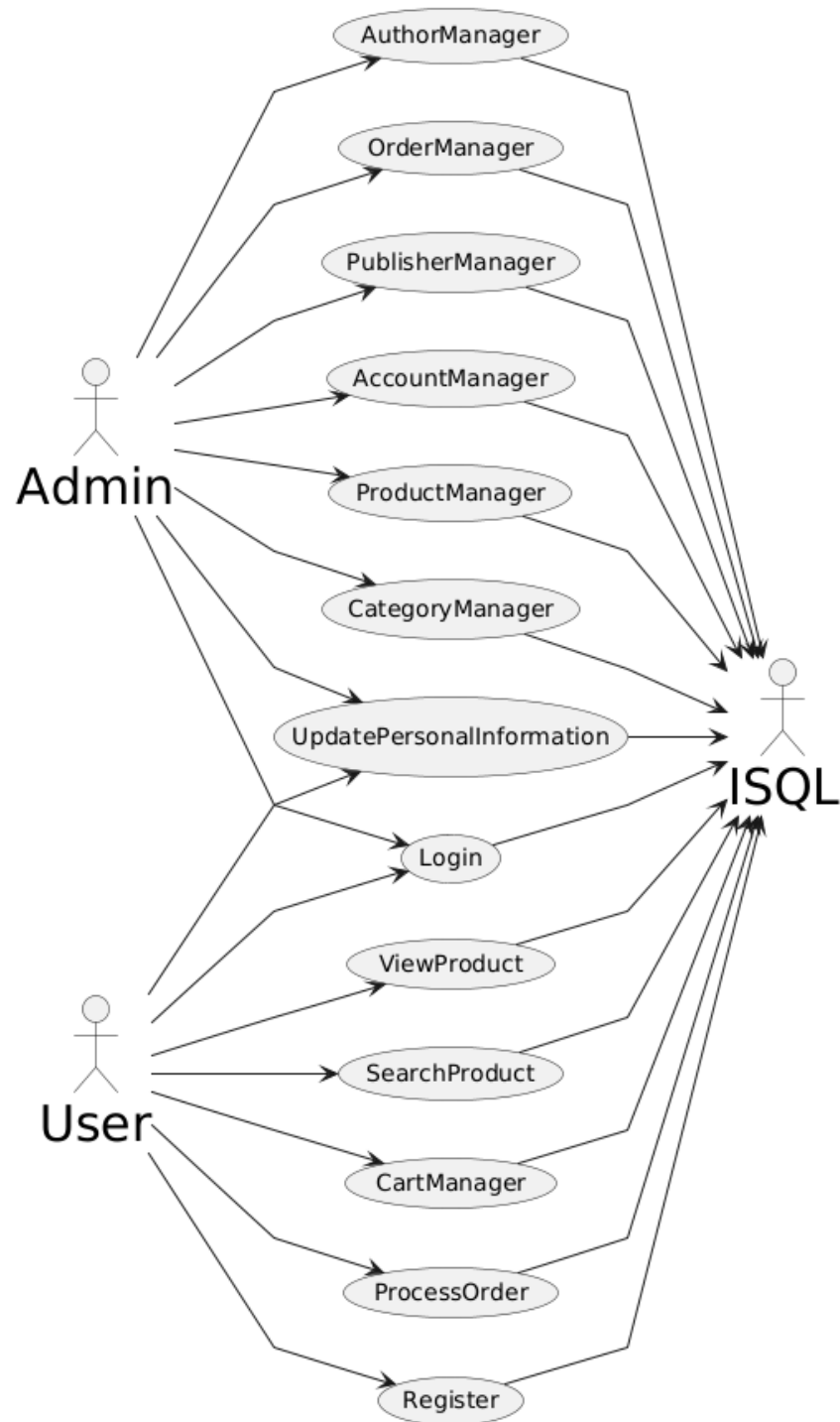
Hình 2.1: Biểu đồ Use case
