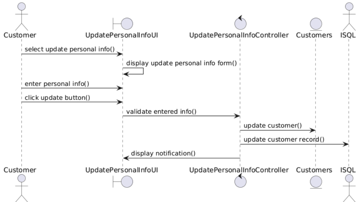
Hình 2.10: Biểu đồ trình tự chức năng cập nhật thông tin cá nhân
