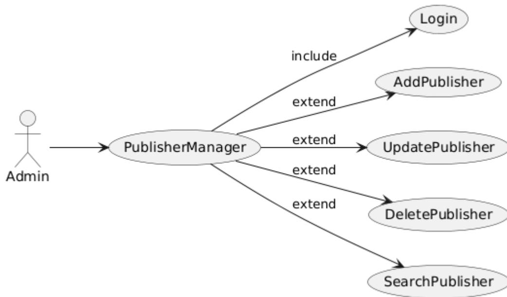
Hình 2.4: Use case quản lý nhà phân phối
