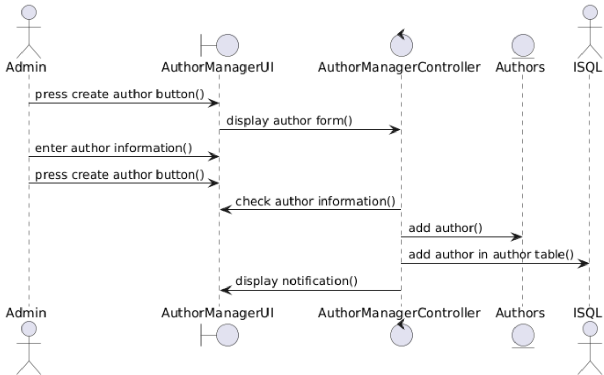
Hình 2.12: Biểu đồ trình tự chức năng thêm mới tác giả
