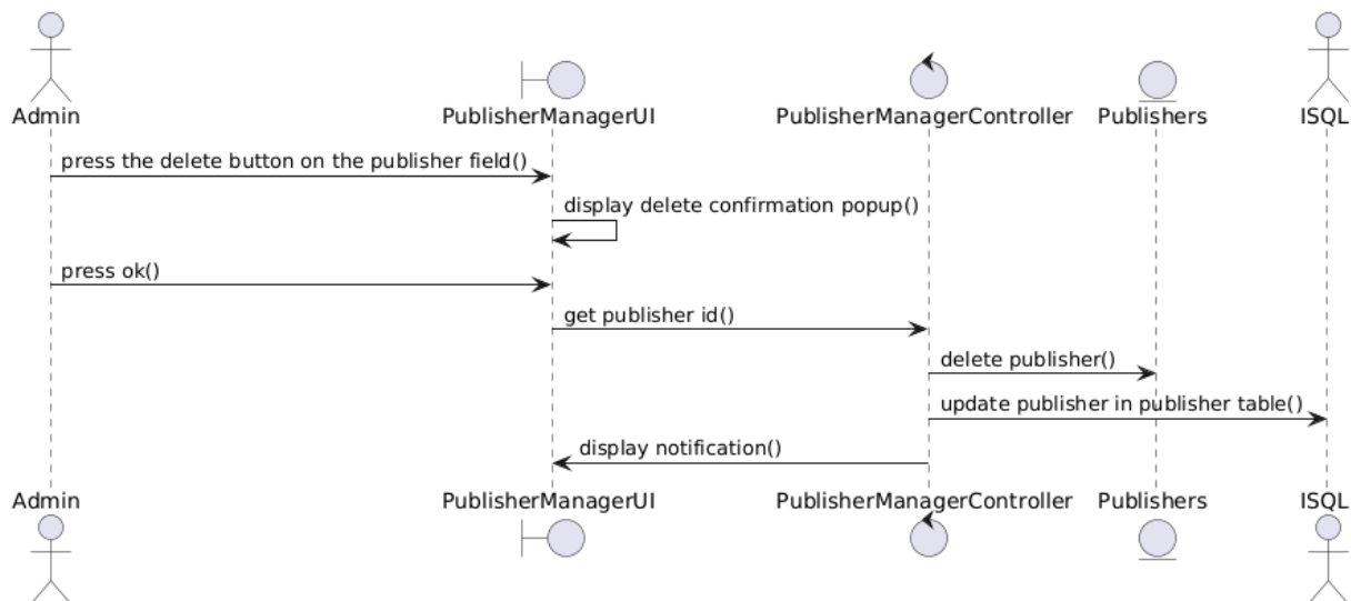
Hình 2.17: Biểu đồ trình tự chức năng xóa nhà phân phối
