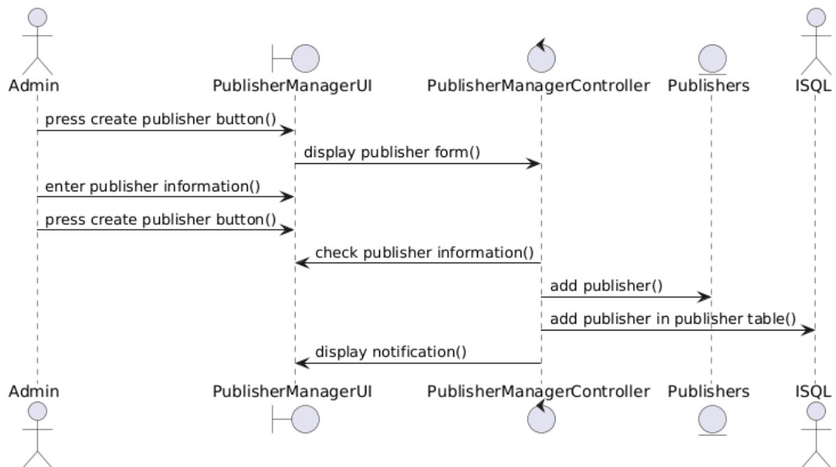
Hình 2.15: Biểu đồ trình tự chức năng thêm mới nhà phân phối
