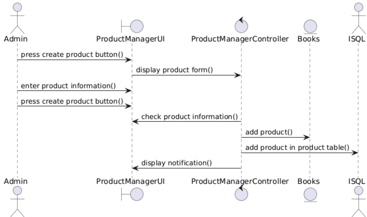
Hình 2.18: Biểu đồ trình tự chức năng thêm mới sản phẩm
