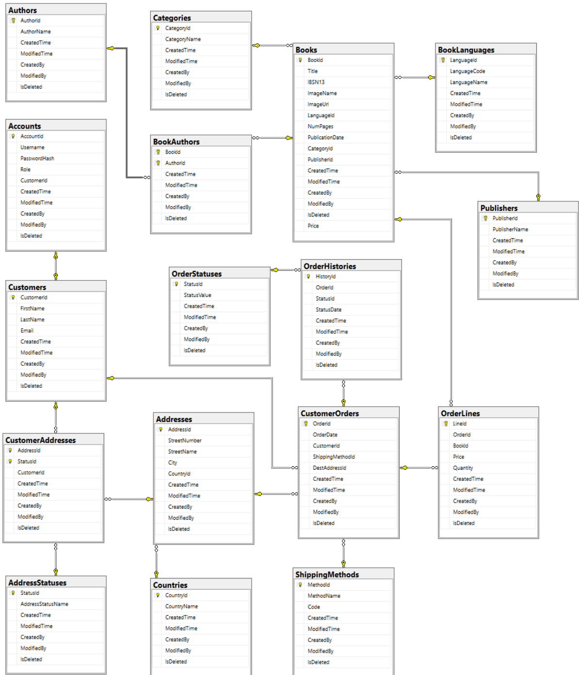
Hình 2.26: Sơ đồ quan hệ giữa các bảng
