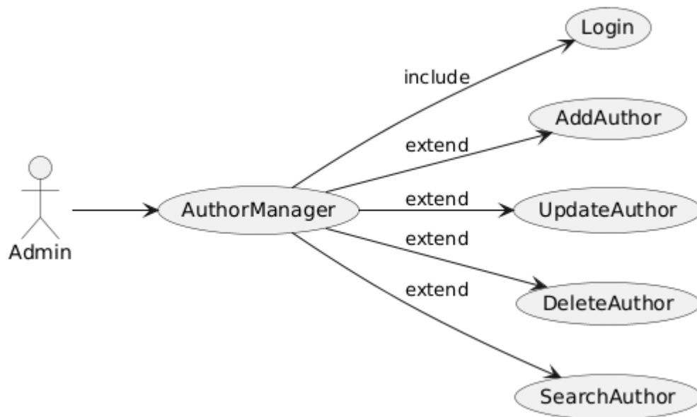
Hình 2.3: Use case quản lý tác giả
