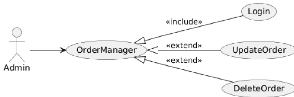
Hình 2.6: Use case quản lý đơn hàng
