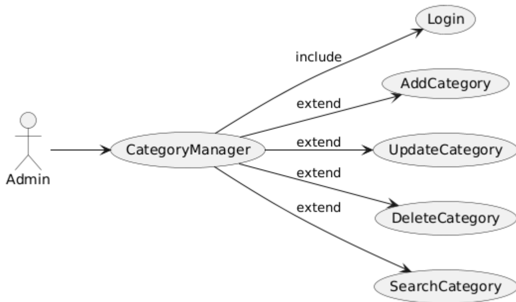
Hình 2.2: Use case quản lý danh mục
