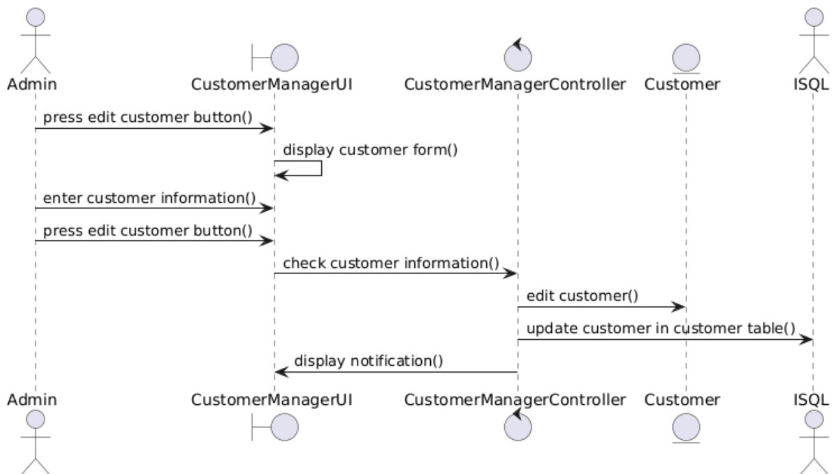
Hình 2.23: Biểu đồ trình tự chức năng quản lý tài khoản khách hàng
