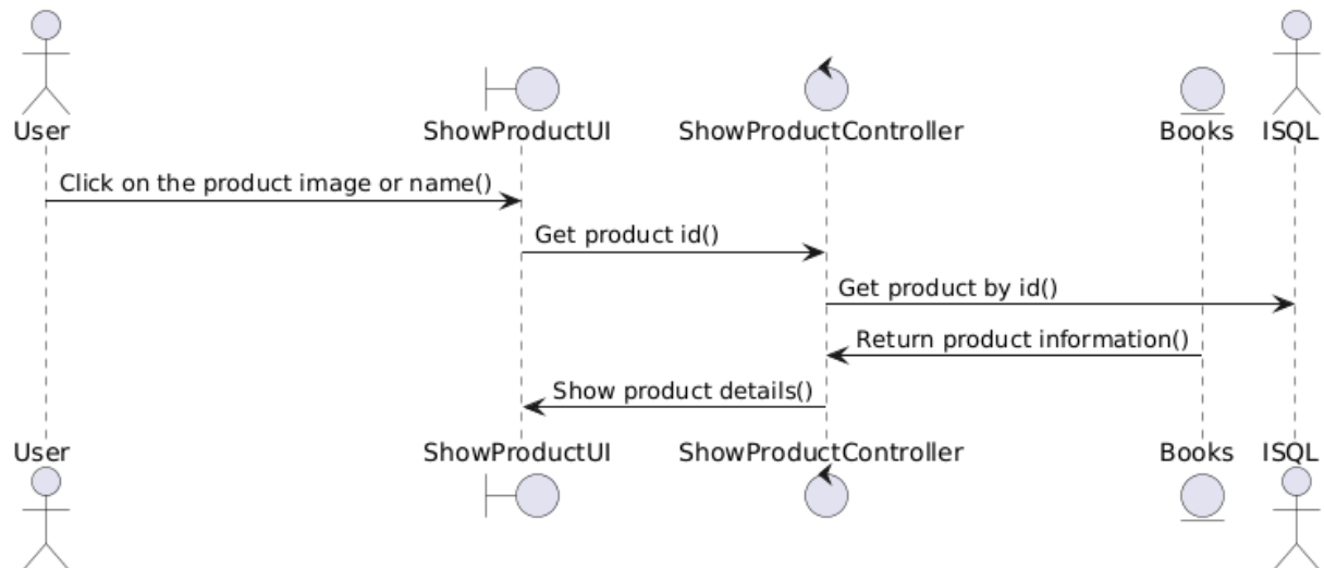
Hình 2.25: Biểu đồ trình tự chức năng xem sản phẩm
