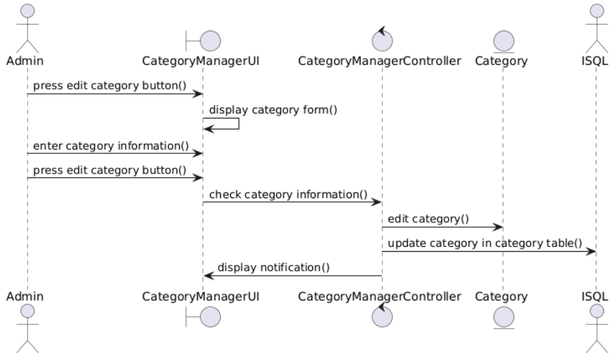
Hình 2.11: Biểu đồ trình tự chức năng cập nhật danh mục
