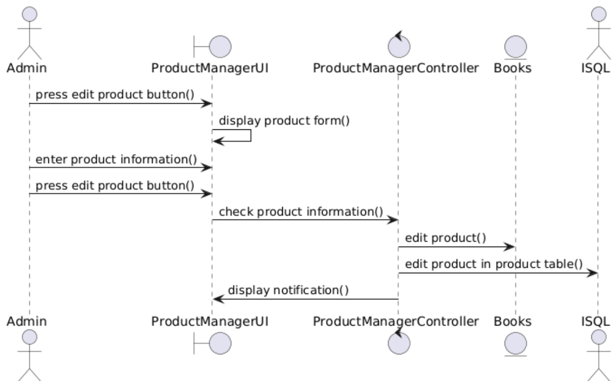
Hình 2.19: Biểu đồ trình tự chức năng cập nhật sản phẩm
