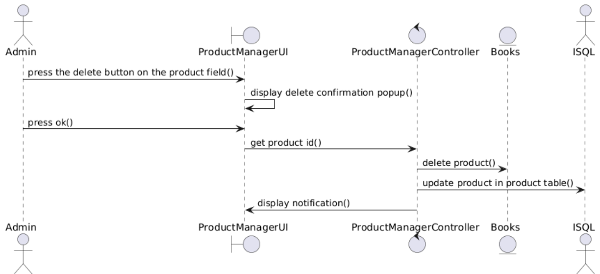
Hình 2.20: Biểu đồ trình tự chức năng xoá sản phẩm
