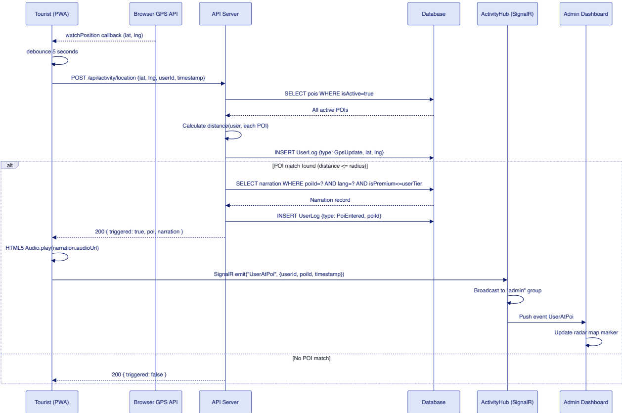
Hình 6.1 — Luồng chính của hệ thống: GPS → API → Narration trigger → Admin realtime update.
