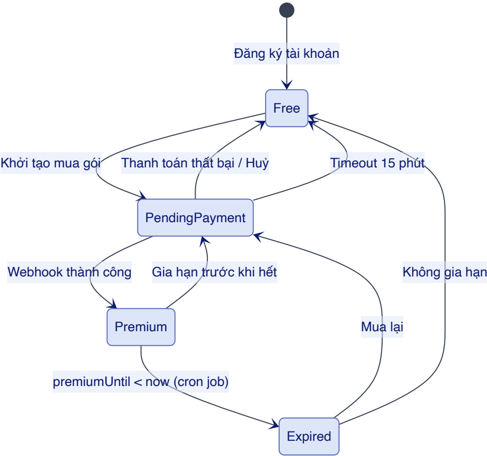
Hình 8.1 — State machine subscription. Cron job chạy hàng giờ để check expiry.
