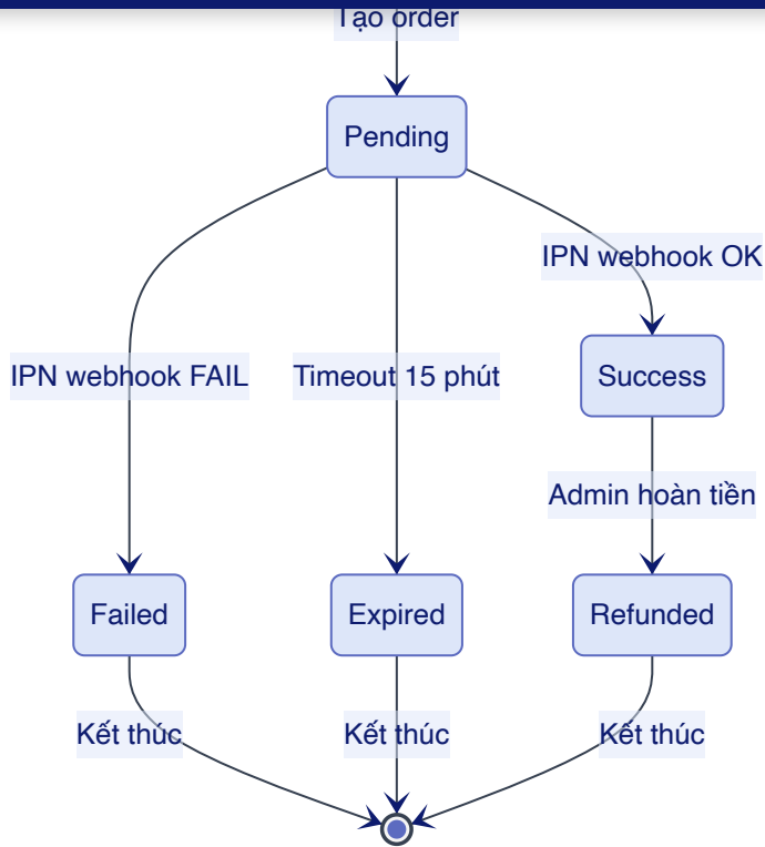
Hình 8.2 — State machine giao dịch thanh toán. Timeout là 15 phút theo quy định VNPay.
