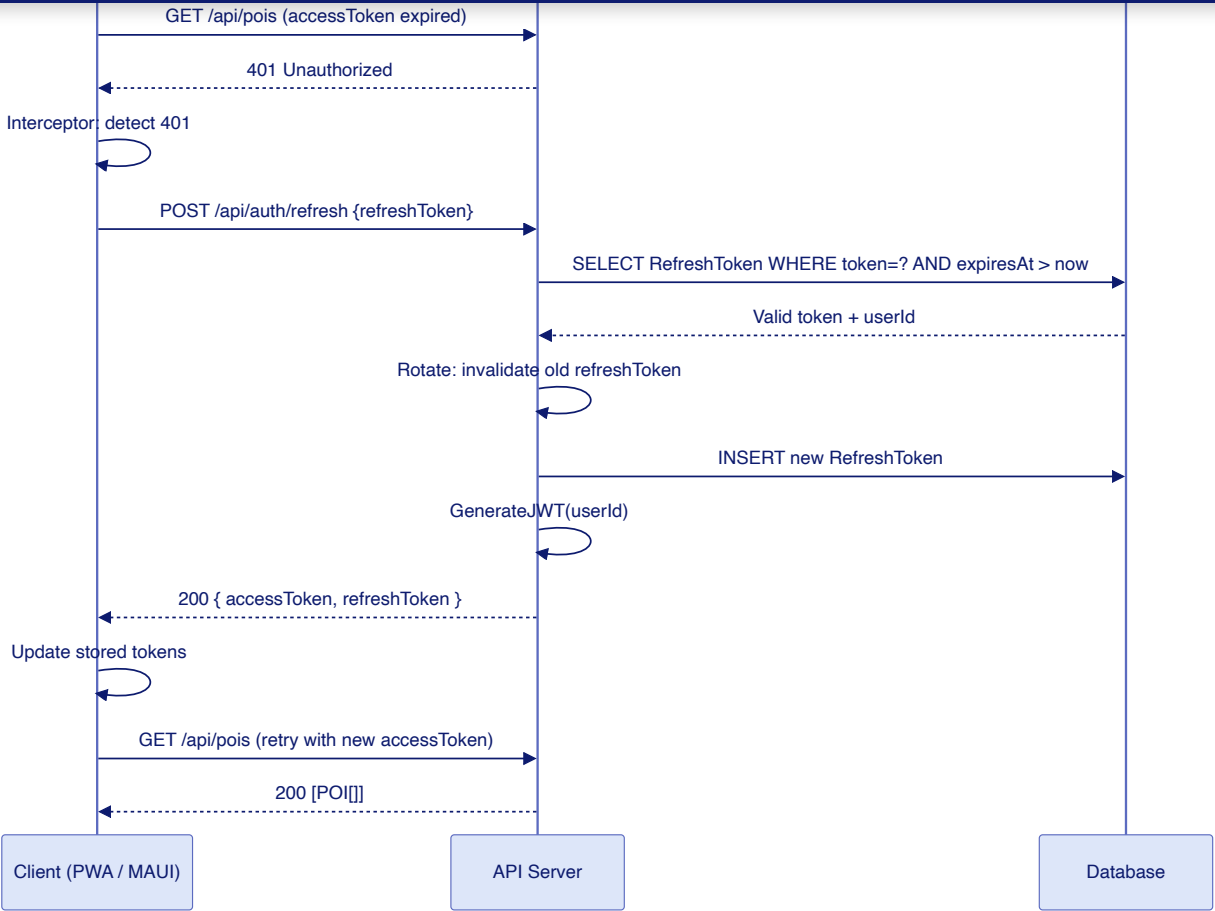
Hình 6.7 — Refresh token rotation: mỗi refresh tạo refreshToken mới, invalidate cái cũ (sliding window).
