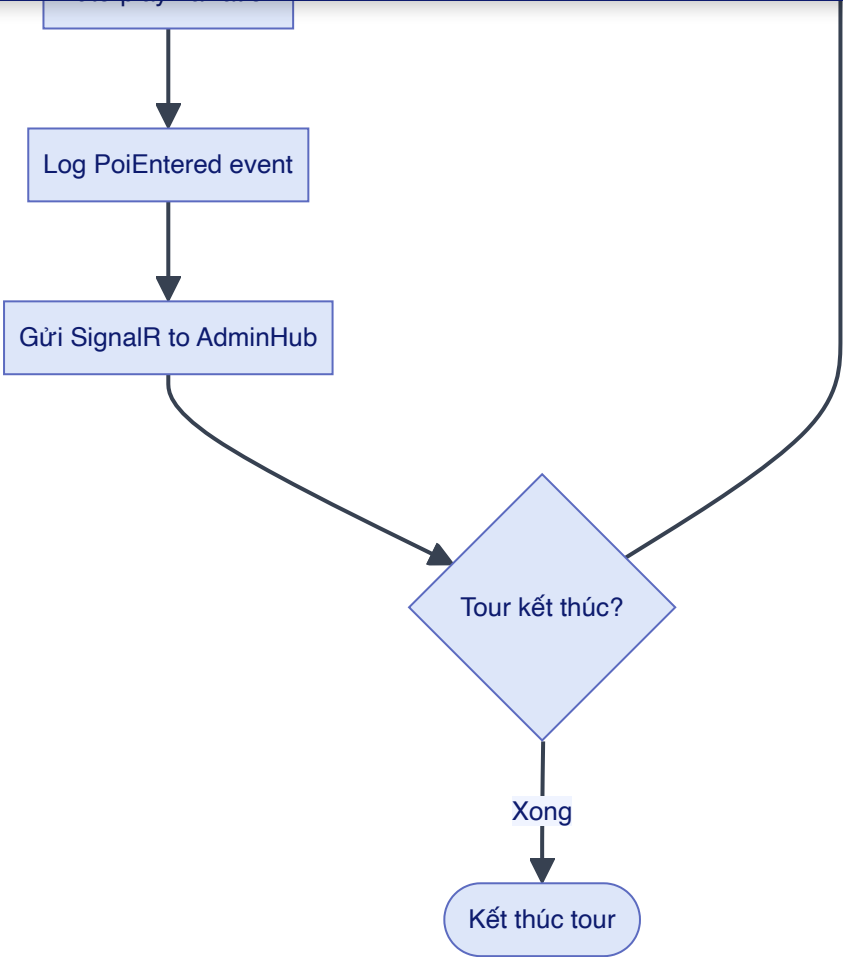
Hình 7.1 — Workflow chính của du khách trong một chuyến tour.
