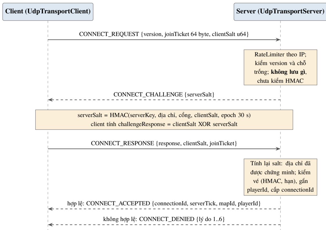
Hình 3.3. Bắt tay challenge – response dùng cookie HMAC: server không cấp tài nguyên cho địa chỉ chưa được chứng minh
