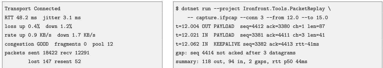
Hình 3.10. Giao diện chẩn đoán: văn bản overlay do TransportDiagnosticsFormatter sinh (trái) và minh họa đầu ra công cụ phát lại gói (phải); các số là minh họa bổ cục
