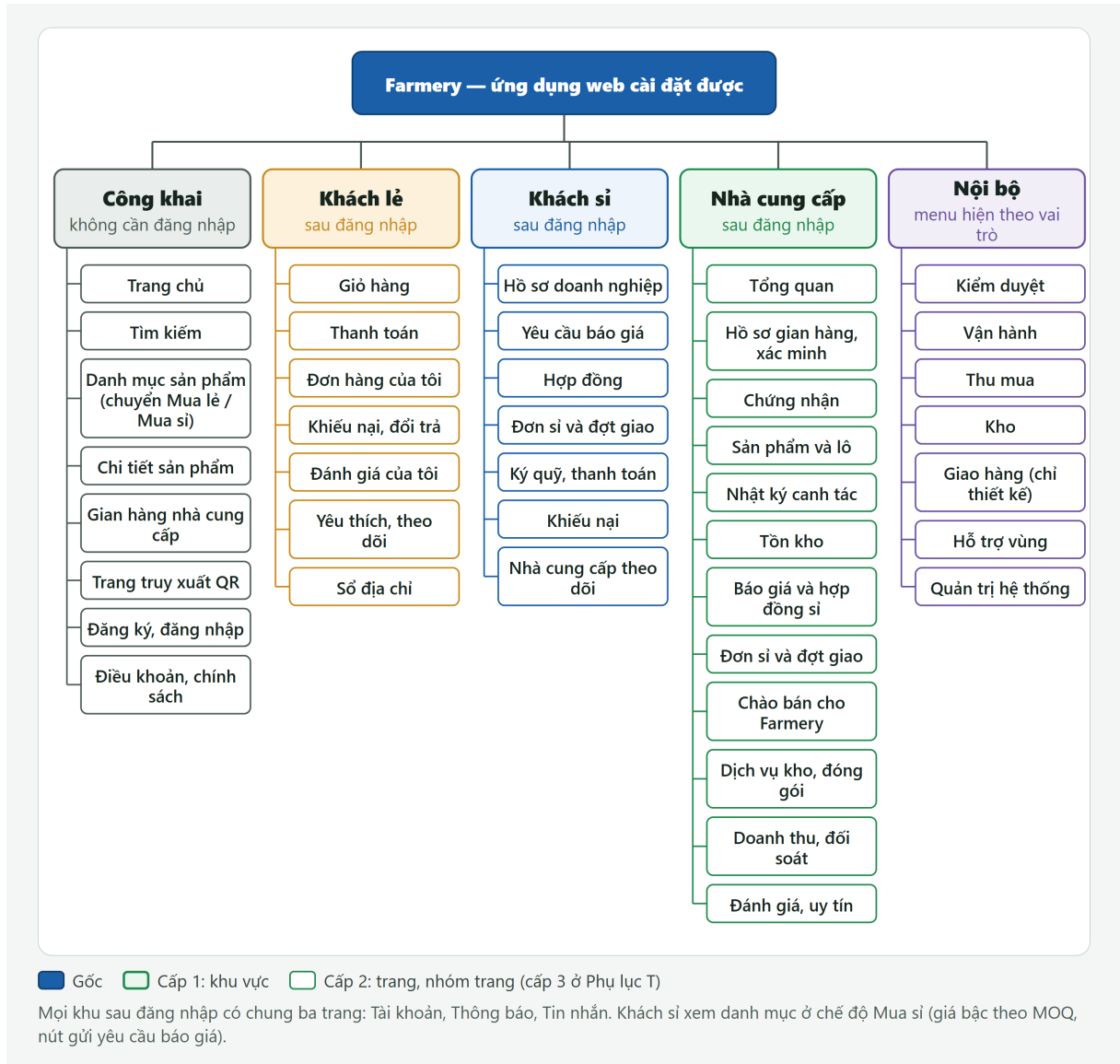
Hình 5.8: Sitemap tổng quan của Farmery (cấp 1 và 2)
