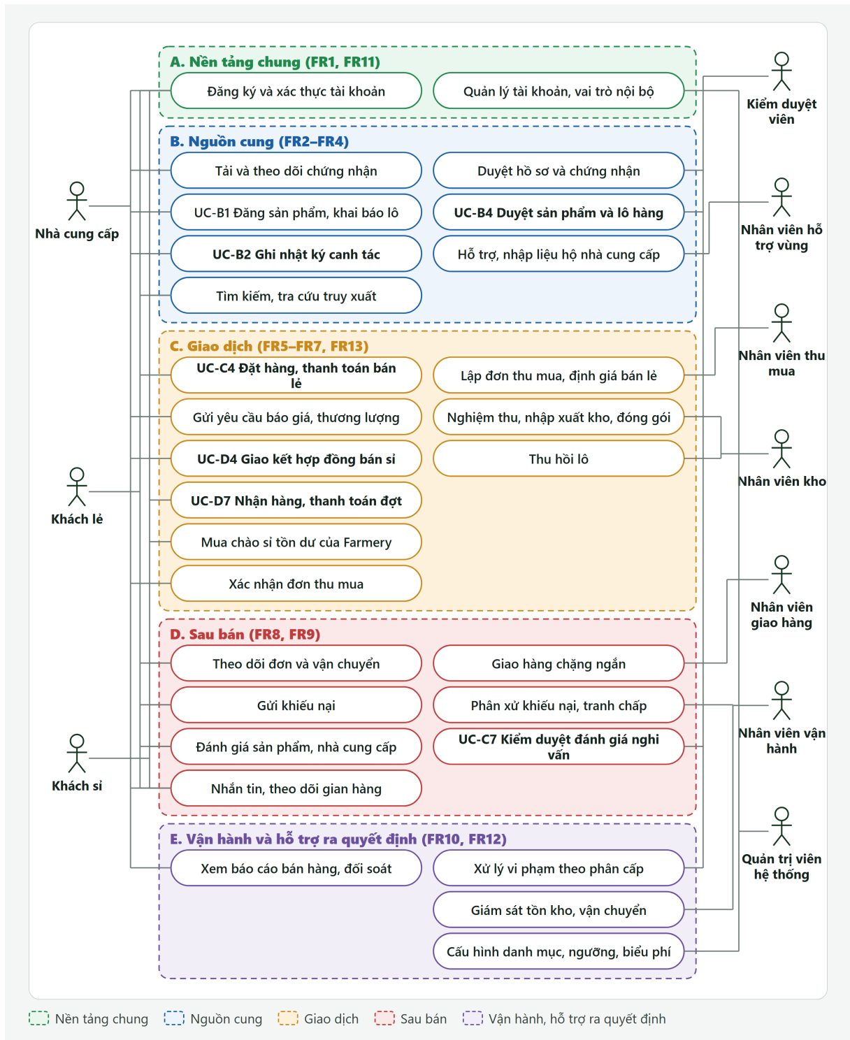
Hình 5.5: Sơ đồ Use Case tổng quan hệ thống Farmery
