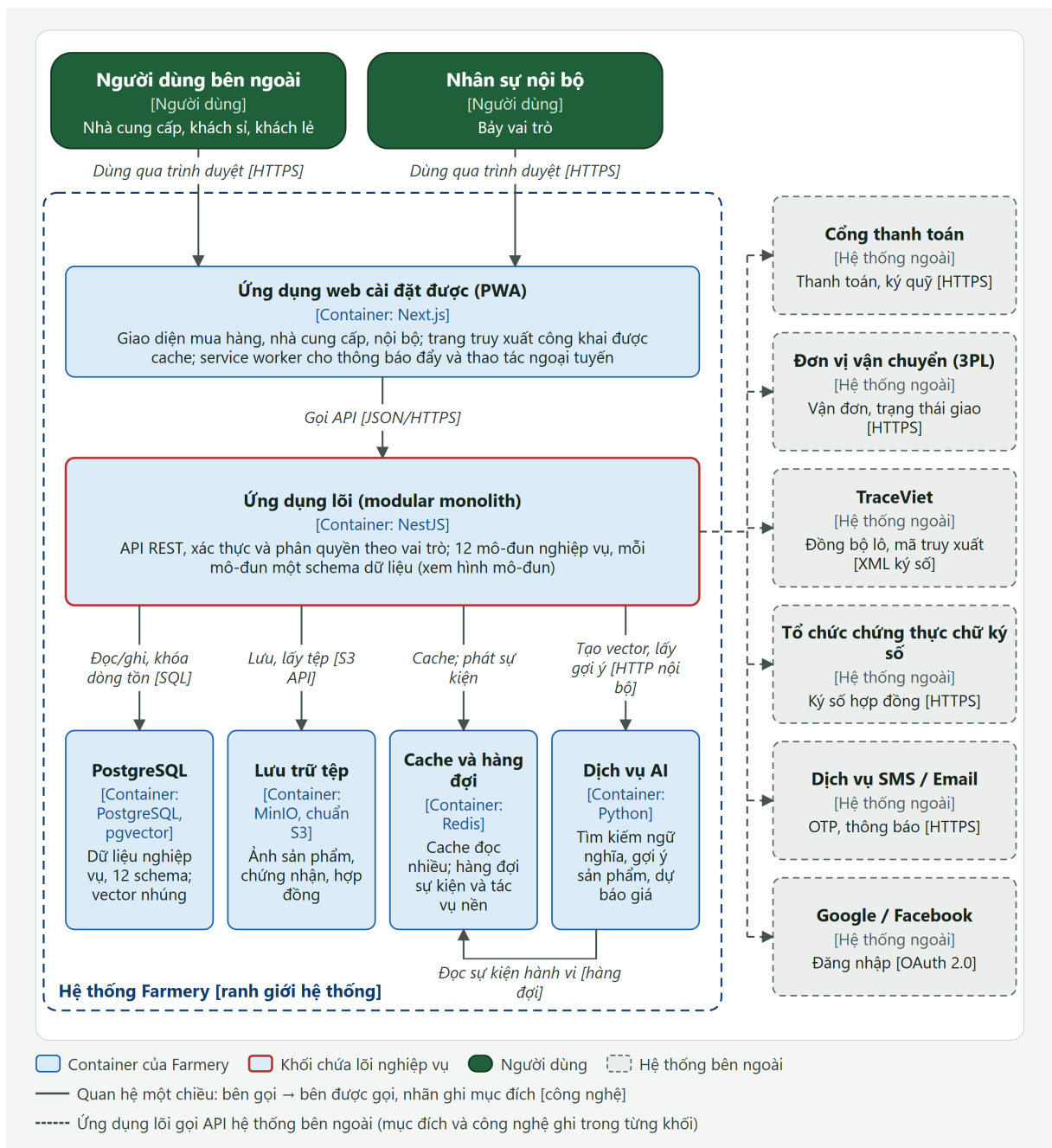
Hình 5.6: Kiến trúc tổng thể của Farmery: các container (C4 mức 2)
