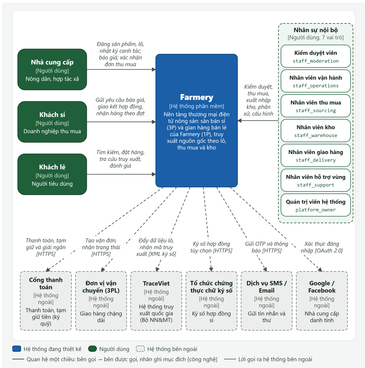
Hình 4.4: Sơ đồ ngữ cảnh của hệ thống Farmery (C4 mức 1)
