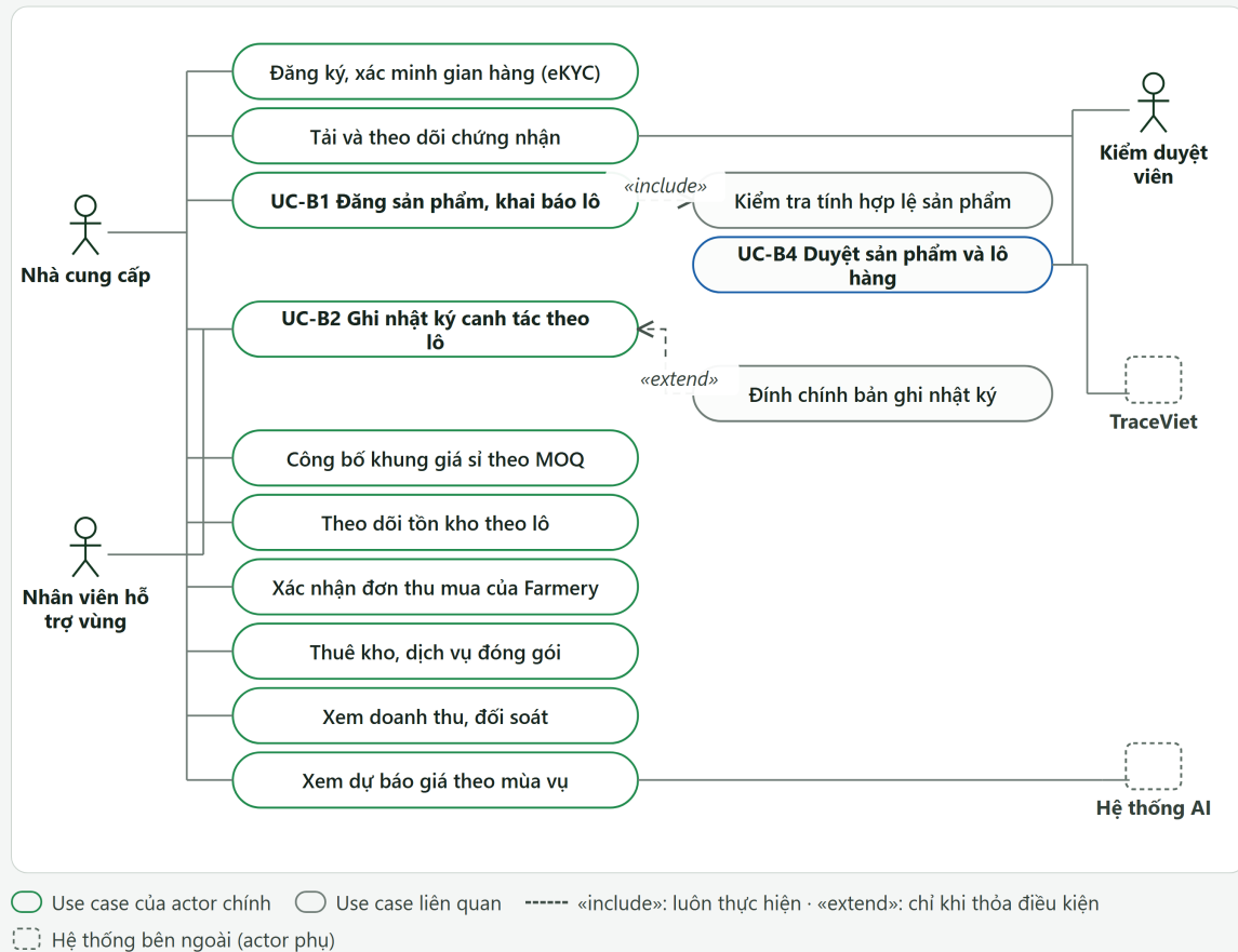
Hình PL.9: Sơ đồ Use Case chi tiết — tác nhân Nhà cung cấp
