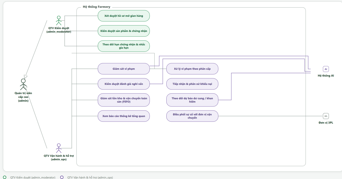
Hình 5.16: Sơ đồ Use Case chi tiết — tác nhân Quản trị viên
