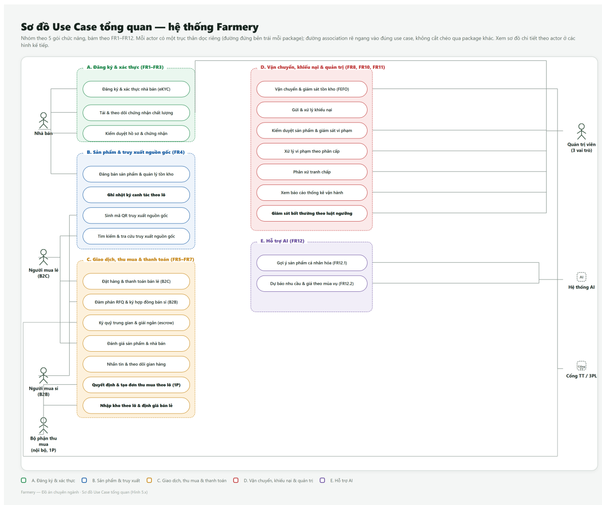
Hình 5.12: Sơ đồ Use Case tổng quan hệ thống Farmery
