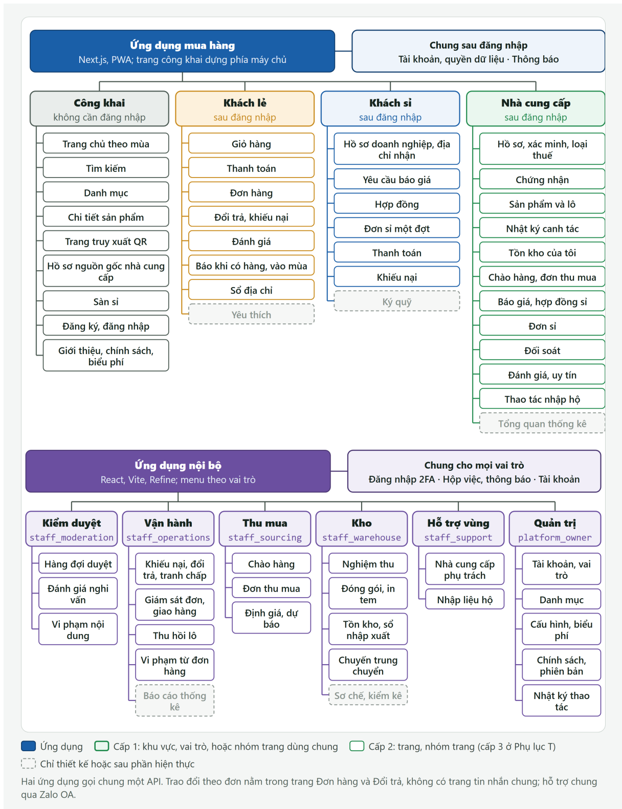
Hình 5.7: Sitemap tổng quan của hai ứng dụng Farmery (cấp 1 và 2)
