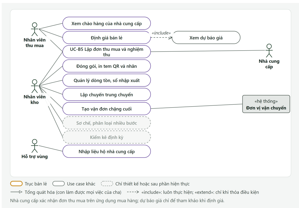
Hình PL.13: Sơ đồ Use Case chi tiết — nhân sự nguồn hàng (thu mua, kho, hỗ trợ vùng)
