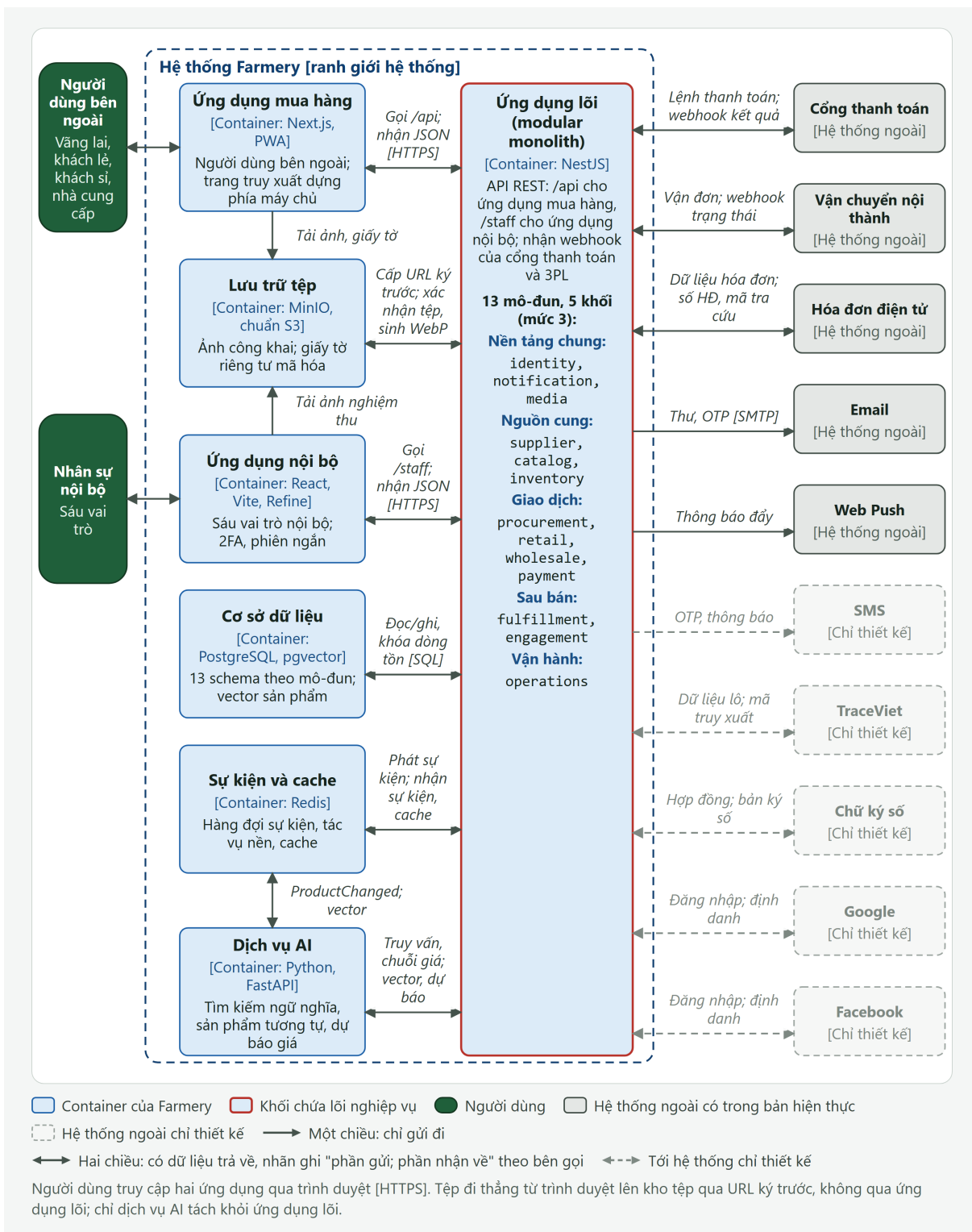
Hình 5.4: Kiến trúc tổng thể của Farmery: các container (C4 mức 2)
