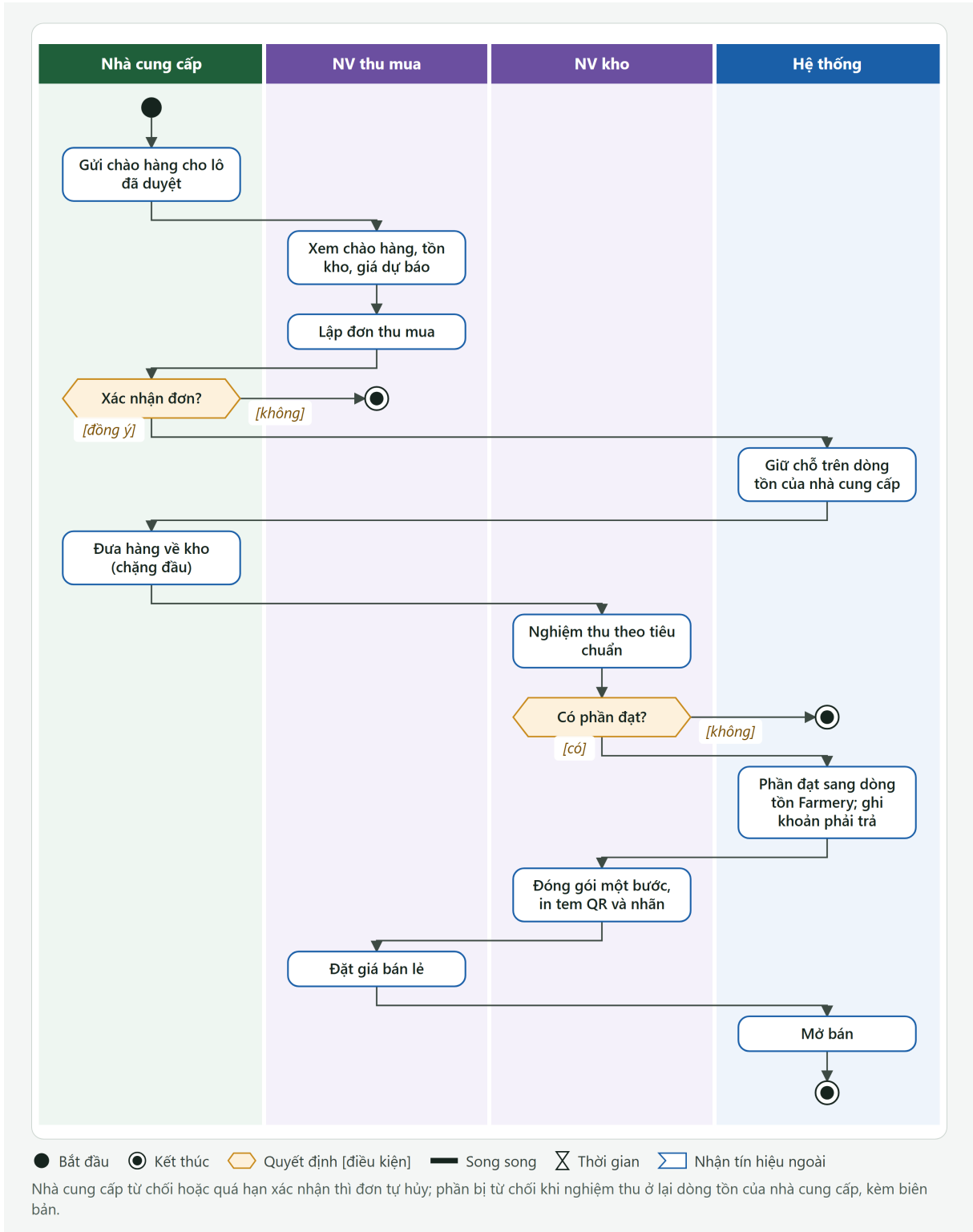
Hình 5.1: Sơ đồ hoạt động: thu mua, nghiệm thu, đóng gói và đặt giá bán lẻ
