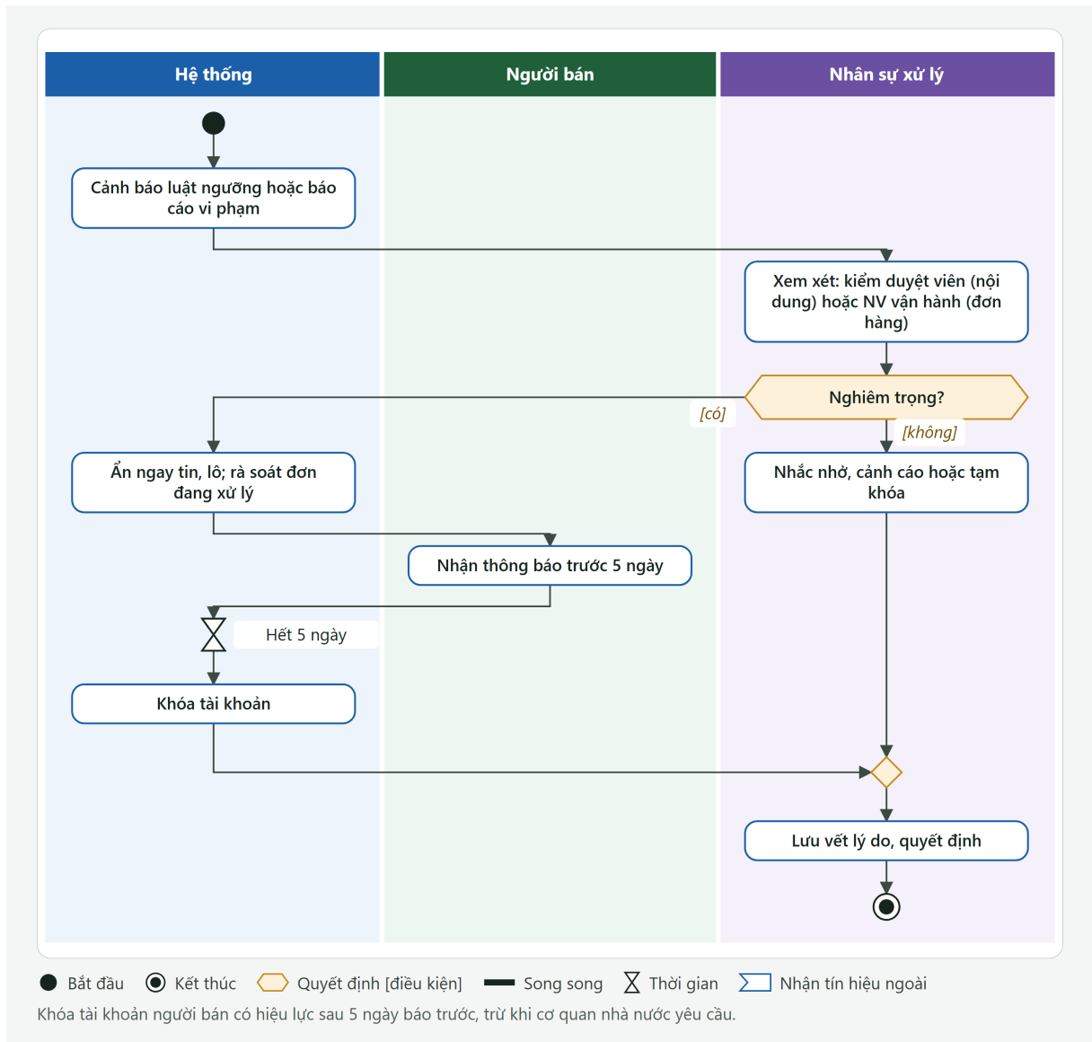
Hình PL.9: Sơ đồ hoạt động: xử lý vi phạm phân cấp
