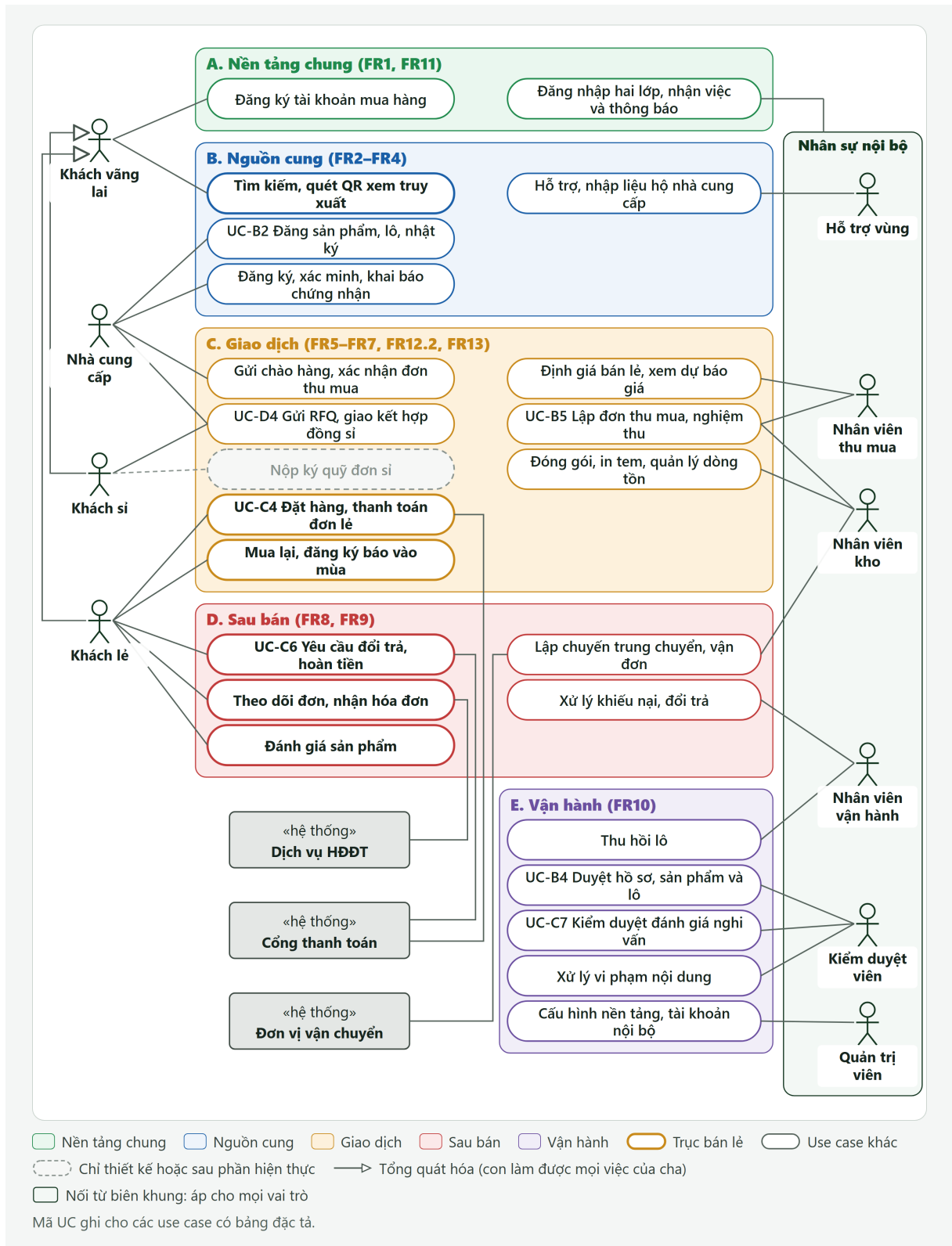
Hình 5.3: Sơ đồ Use Case tổng quan hệ thống Farmery
