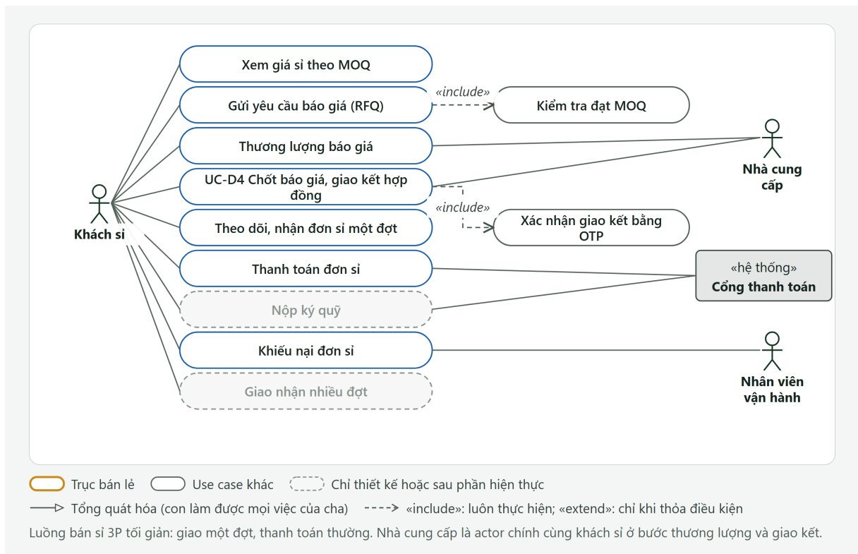
Hình PL.12: Sơ đồ Use Case chi tiết — tác nhân Khách sỉ
