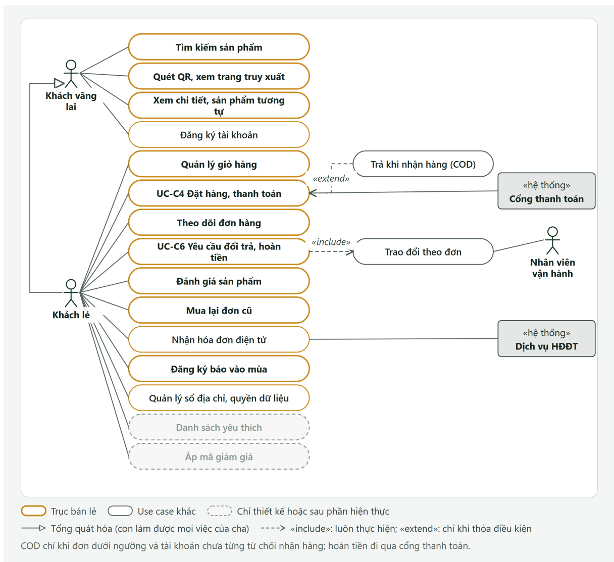
Hình PL.11: Sơ đồ Use Case chi tiết — khách vắng lai và khách lẻ
