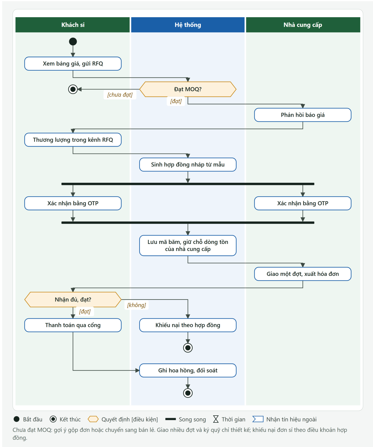
Hình PL.6: Sơ đồ hoạt động: bán sỉ từ yêu cầu báo giá, hợp đồng tới giao một đợt
