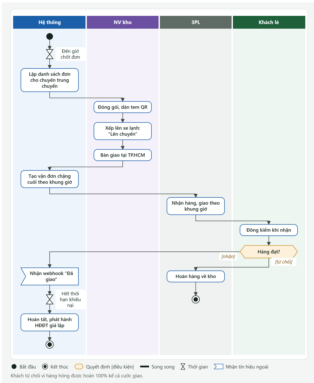
Hình PL.2: Sơ đồ hoạt động: giao nhận đơn lẻ qua ba chặng
