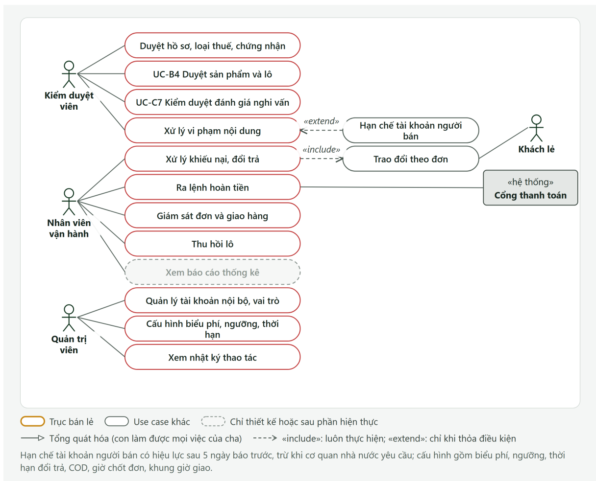
Hình PL.14: Sơ đồ Use Case chi tiết — nhân sự kiểm duyệt, vận hành và quản trị viên
