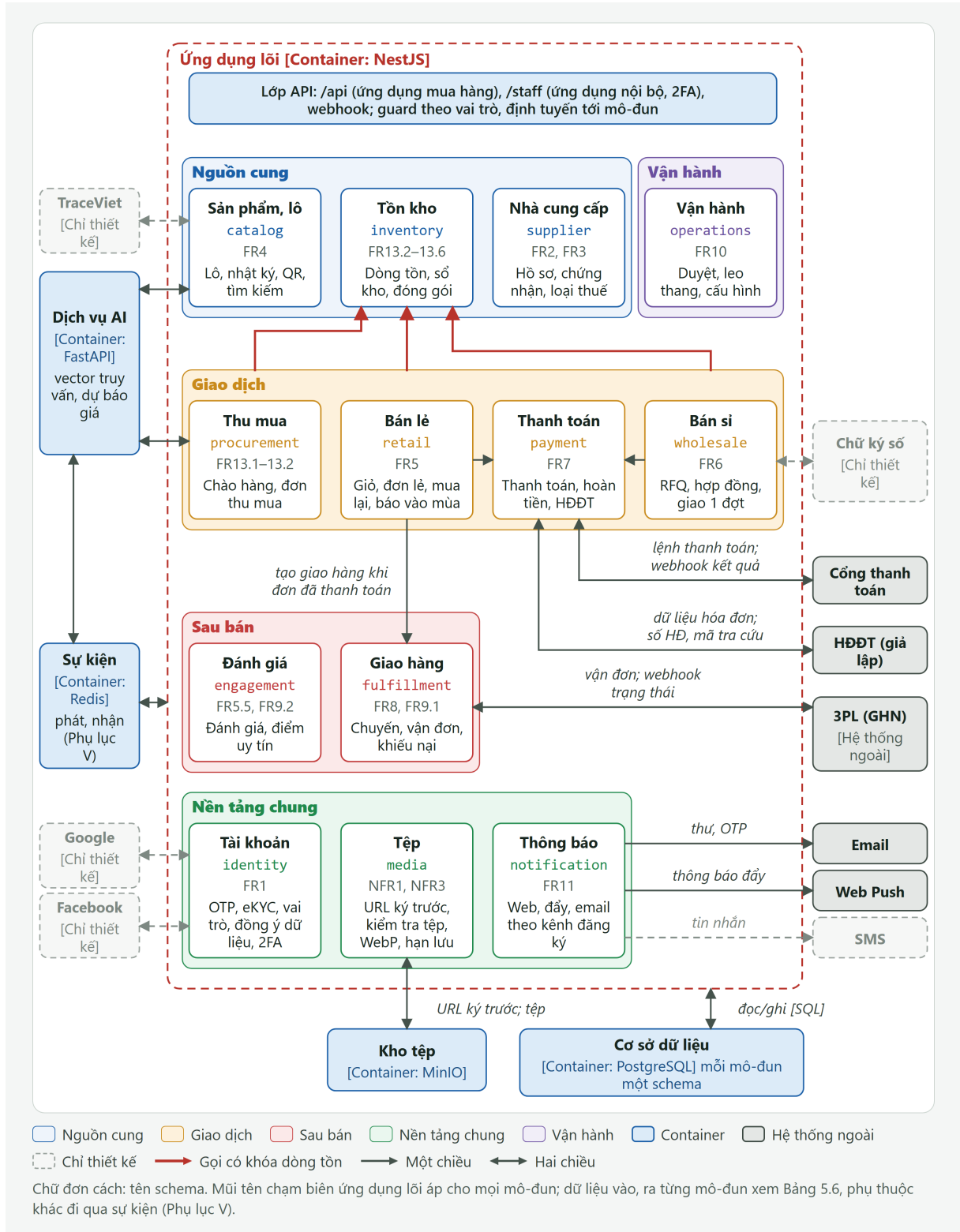
Hình 5.5: Các mô-đun của ứng dụng lõi (C4 mức 3)
