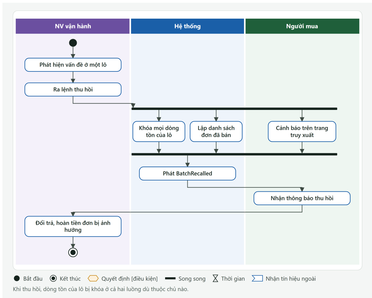
Hình PL.8: Sơ đồ hoạt động: thu hồi lô
