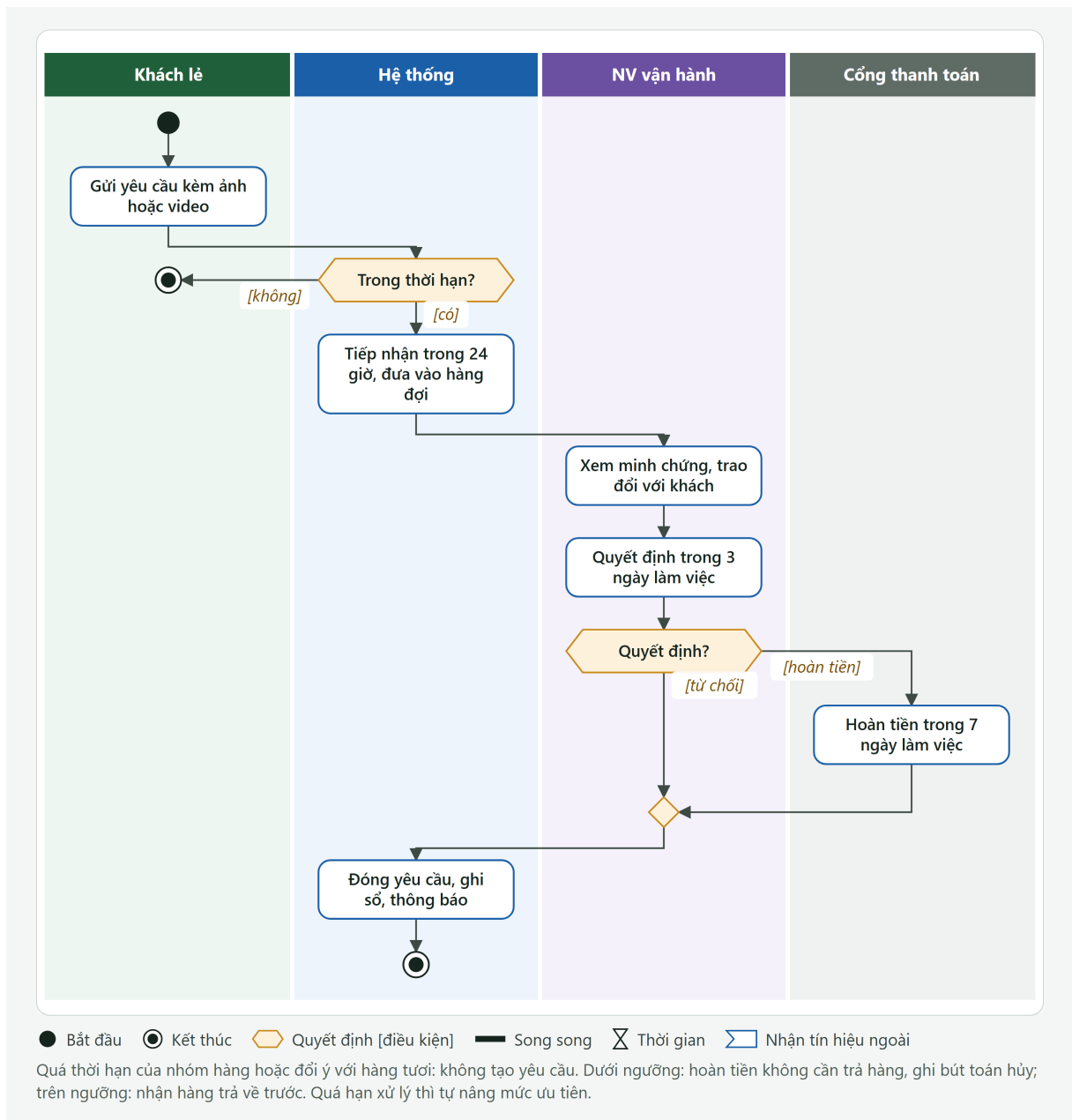
Hình PL.3: Sơ đồ hoạt động: đổi trả và hoàn tiền đơn lẻ
