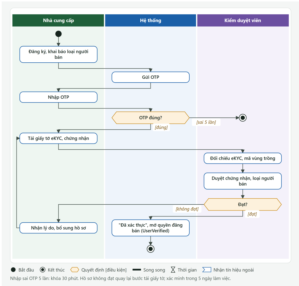
Hình PL.4: Sơ đồ hoạt động: đăng ký, xác minh nhà cung cấp
