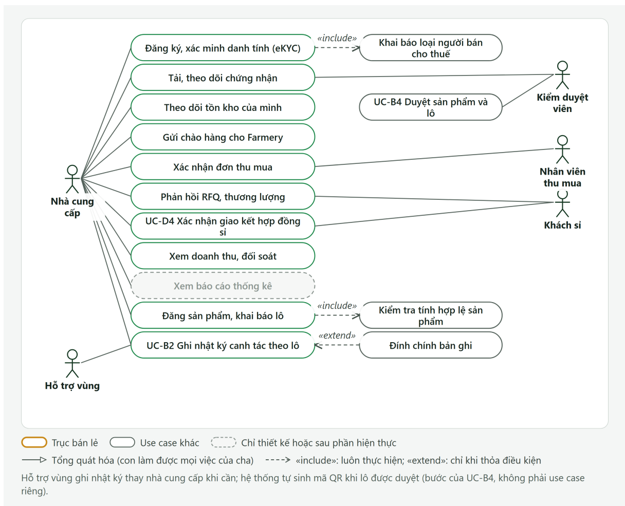
Hình PL.10: Sơ đồ Use Case chi tiết — tác nhân Nhà cung cấp
