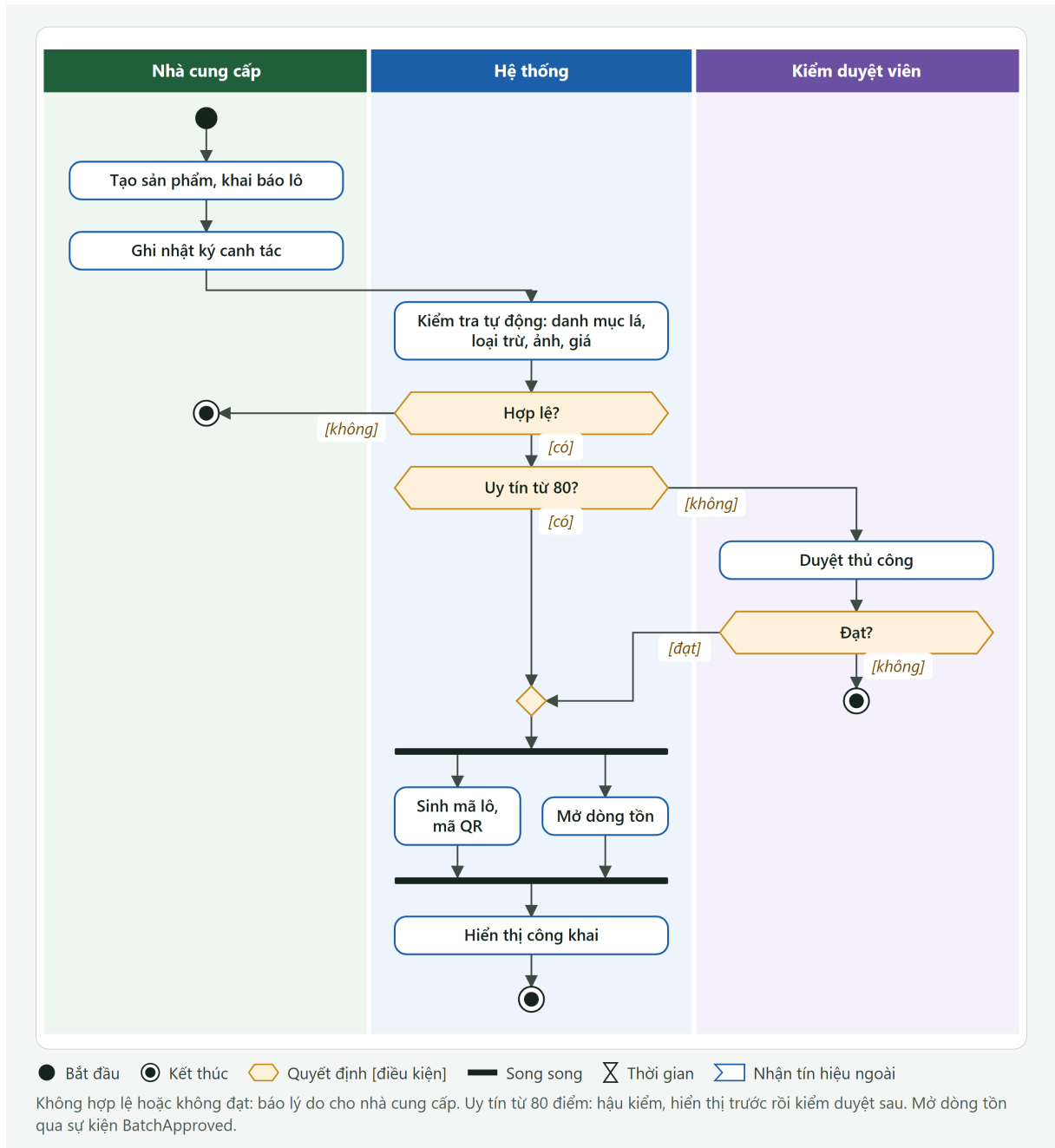
Hình PL.5: Sơ đồ hoạt động: đăng sản phẩm, duyệt lô và sinh mã QR
