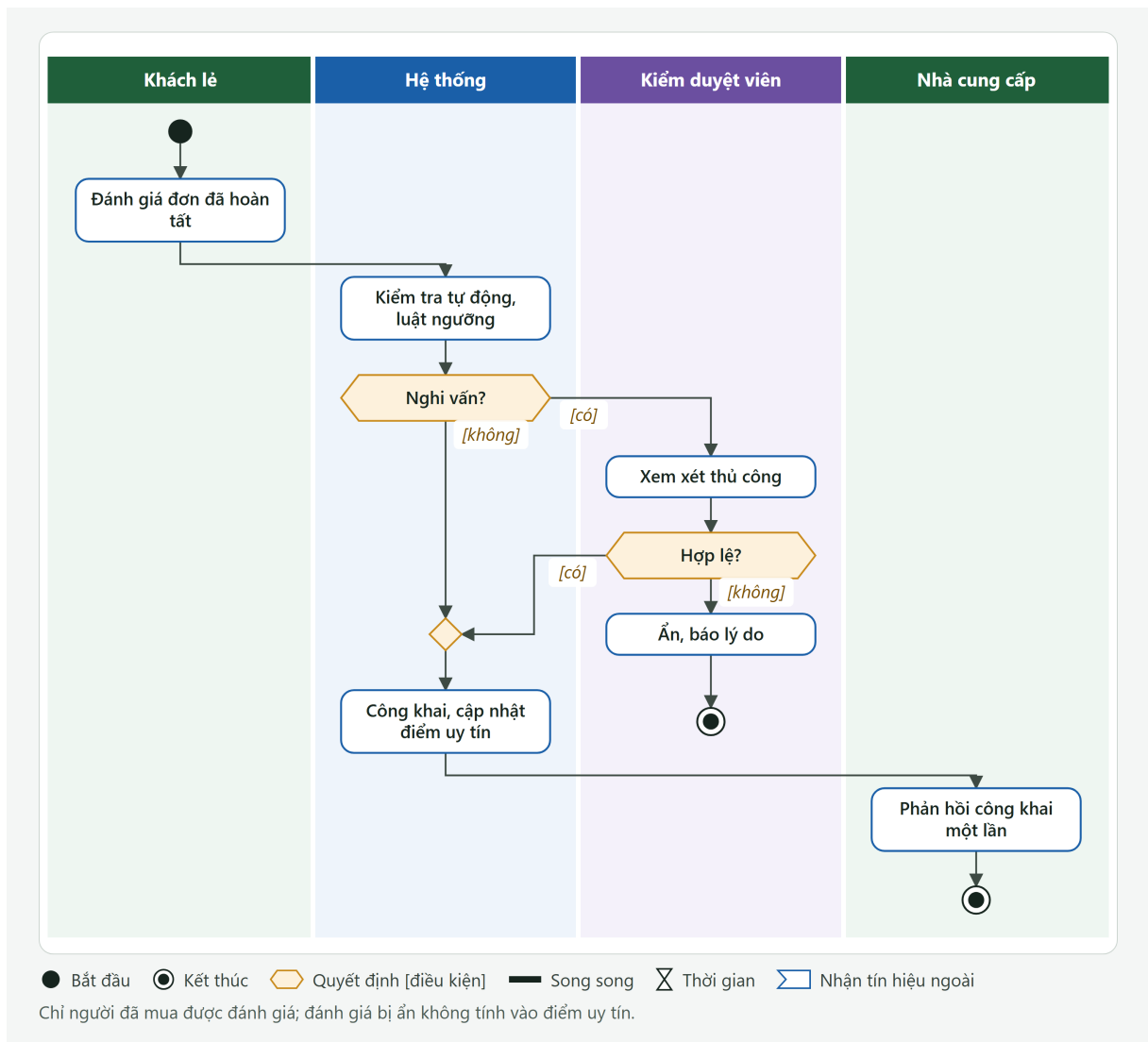
Hình PL.7: Sơ đồ hoạt động: đánh giá và kiểm duyệt đánh giá
