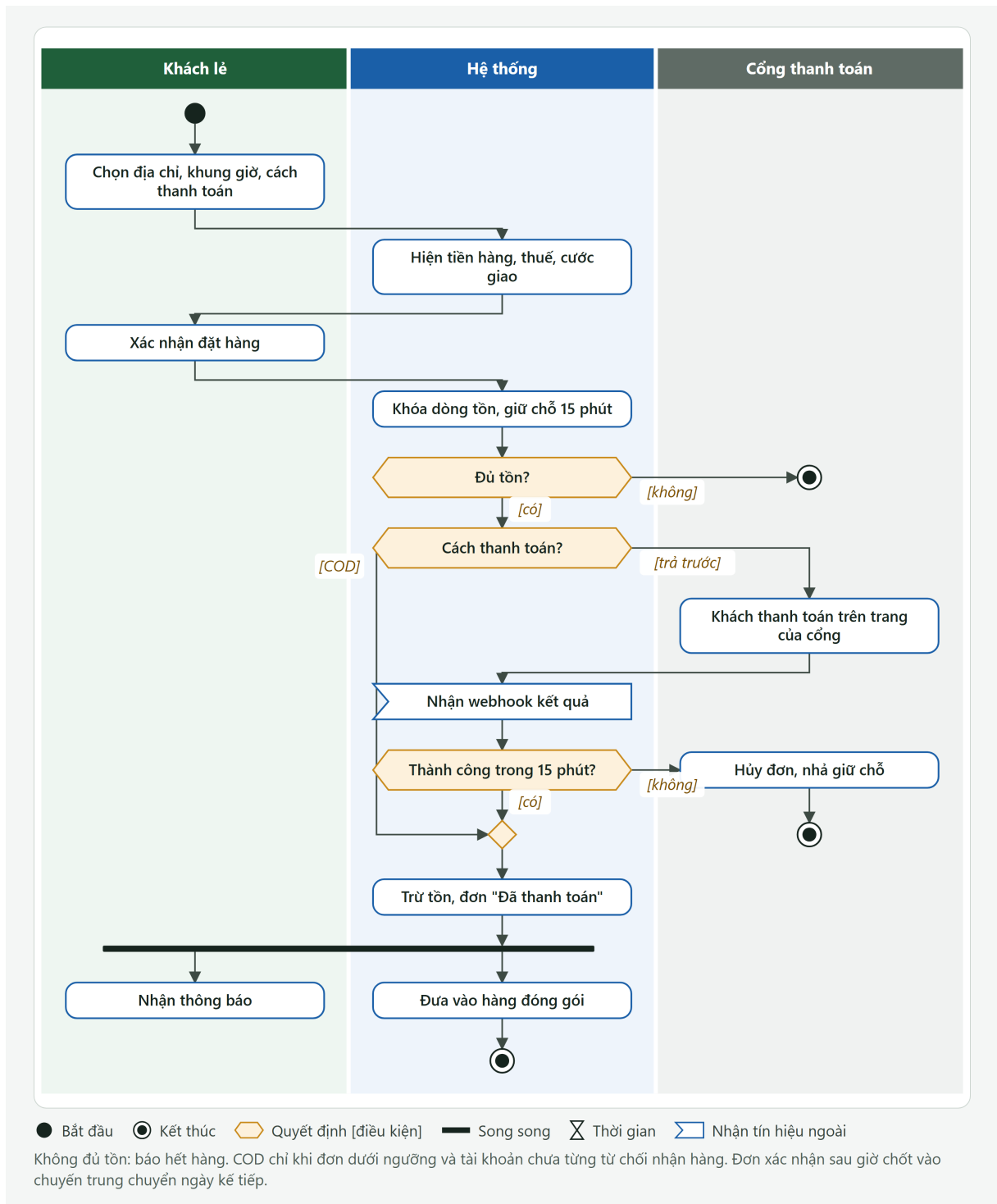
Hình 5.2: Sơ đồ hoạt động: đặt hàng, giữ chỗ tồn kho và thanh toán đơn lẻ
