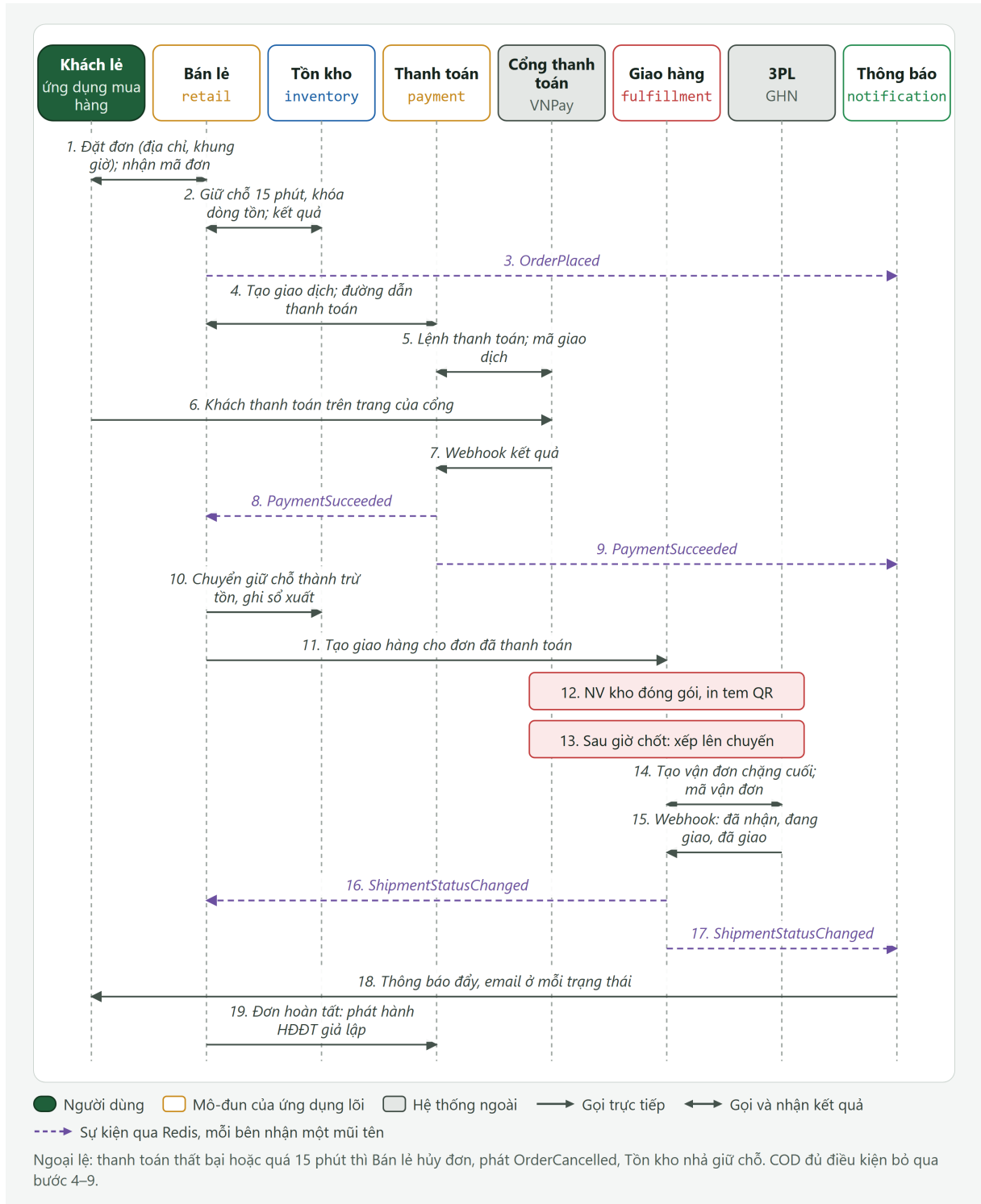
Hình 5.6: Luồng một đơn bán lẻ qua các mô-đun và hệ thống bên ngoài
