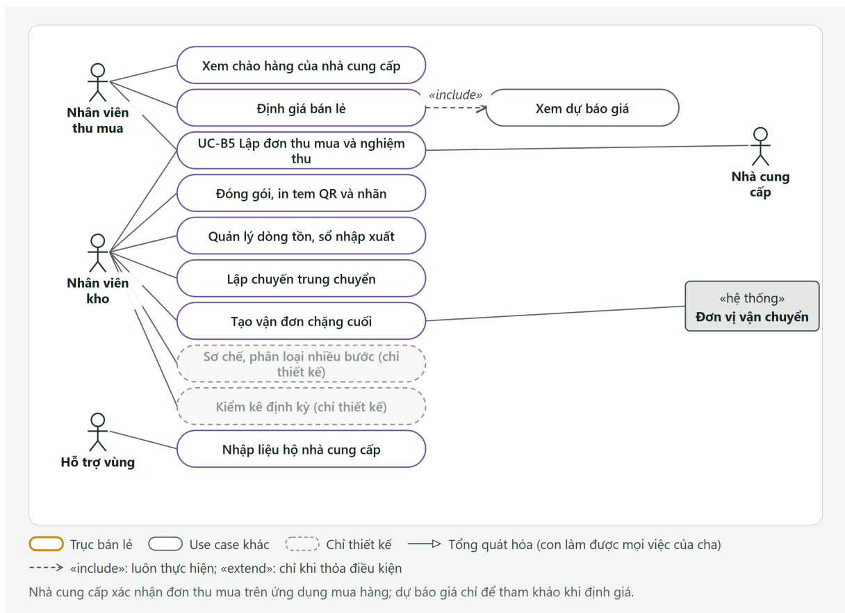
Hình PL.12: Sơ đồ Use Case chi tiết — nhân sự nguồn hàng (thu mua, kho, hỗ trợ vùng)
