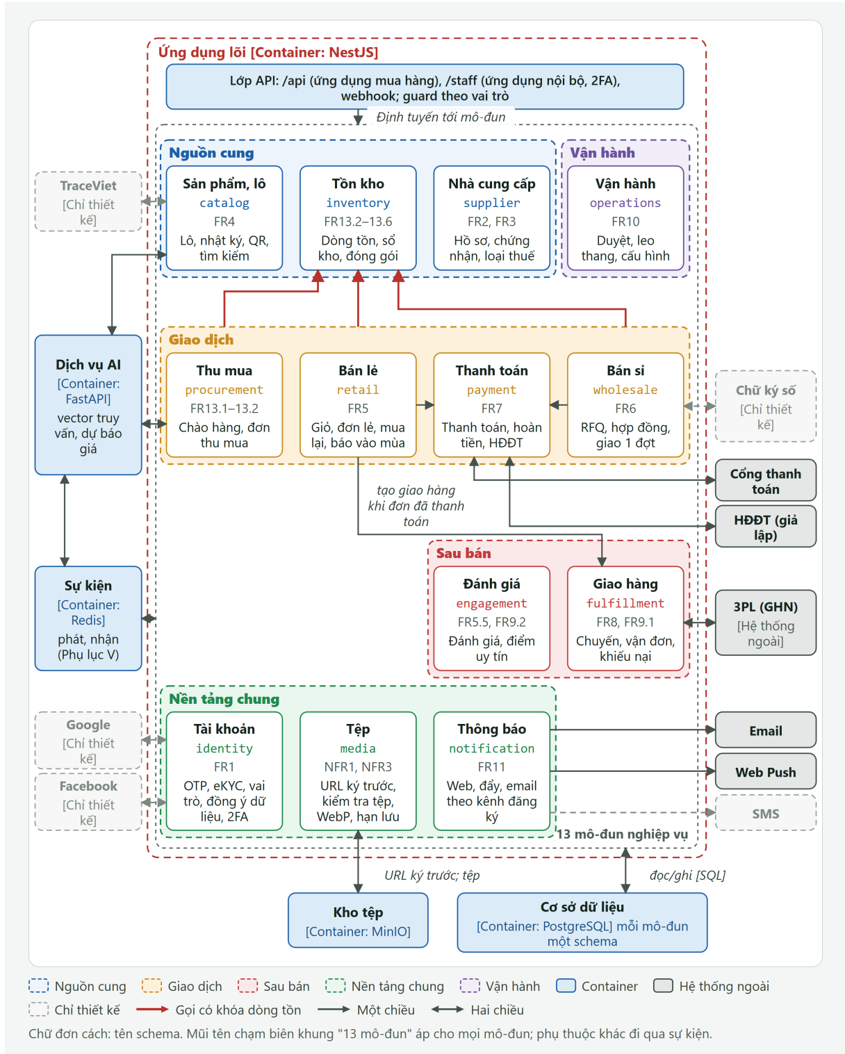
Hình 5.7: Các mô-đun của ứng dụng lõi (C4 mức 3)
