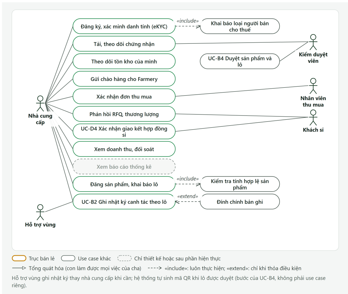
Hình PL.8: Sơ đồ Use Case chi tiết — tác nhân Nhà cung cấp
