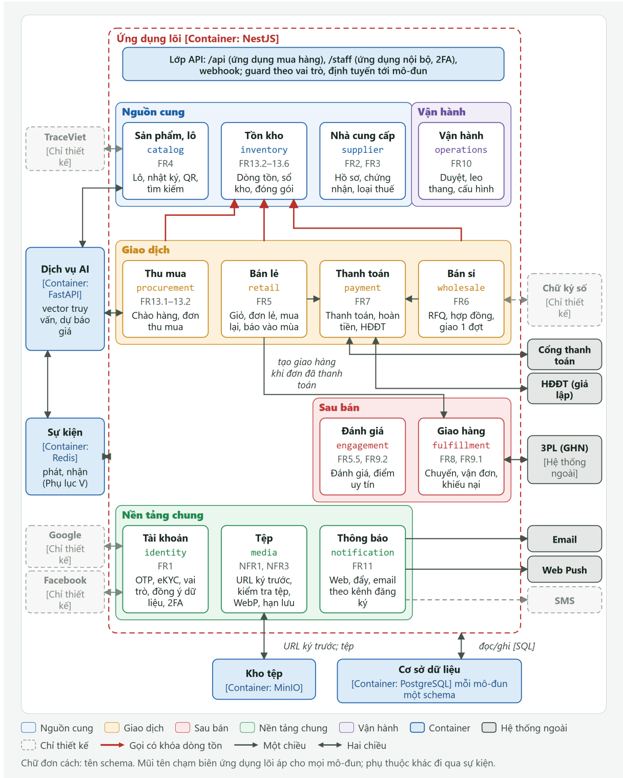
Hình 5.5: Các mô-đun của ứng dụng lõi (C4 mức 3)
