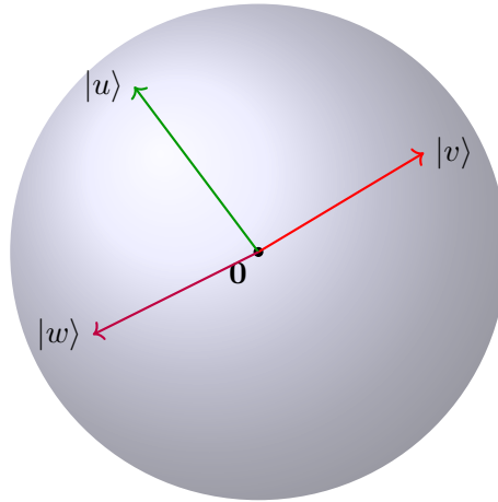
Hình 2: Minh họa vector và không gian vector
