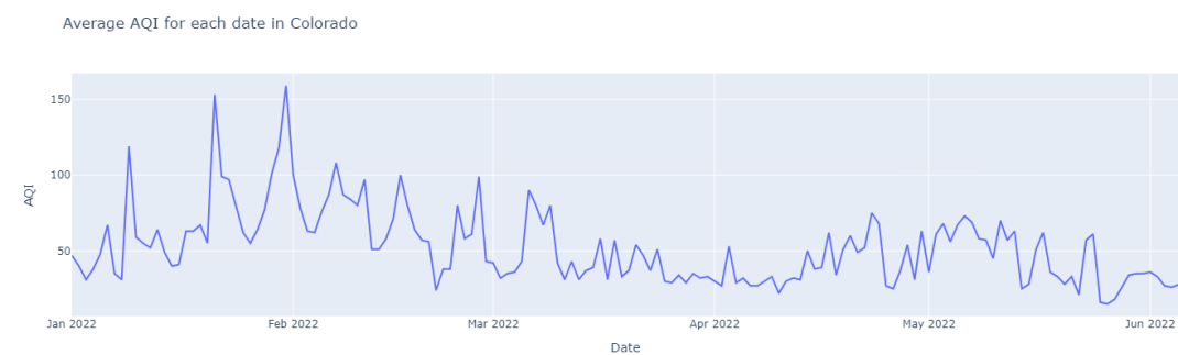
Hình 26: AQI trung bình của Colorado theo thời gian
