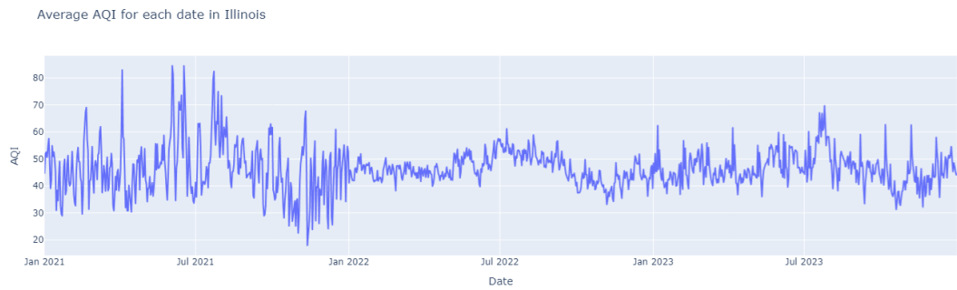
Hình 31: AQI trung bình của Illinois theo thời gian
