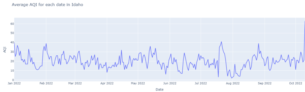
Hình 30: AQI trung bình của Idaho theo thời gian
