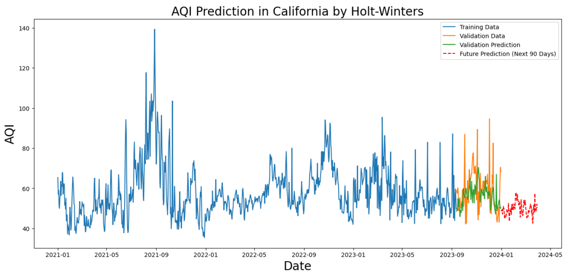
Hình 37: Dự đoán quý 1/2024 chất lượng không khí ở California sử dụng mô hình Holt-Winters
