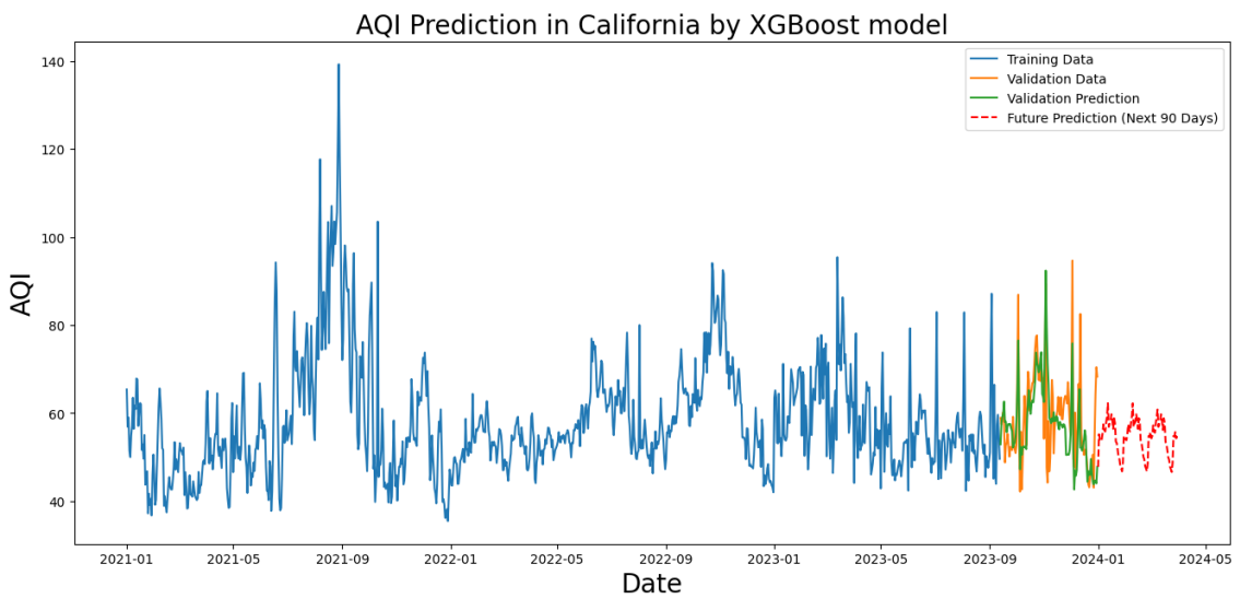
Hình 35: Dự đoán quý 1/2024 chất lượng không khí ở California sử dụng mô hình XGBoost
