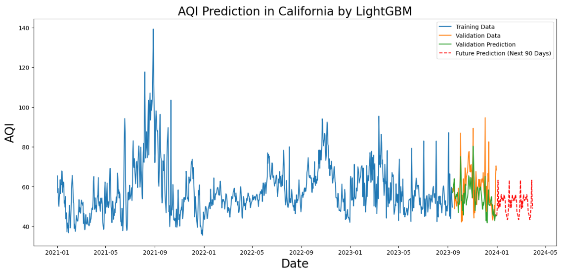
Hình 36: Dự đoán quý 1/2024 chất lượng không khí ở California sử dụng mô hình LightGBM
