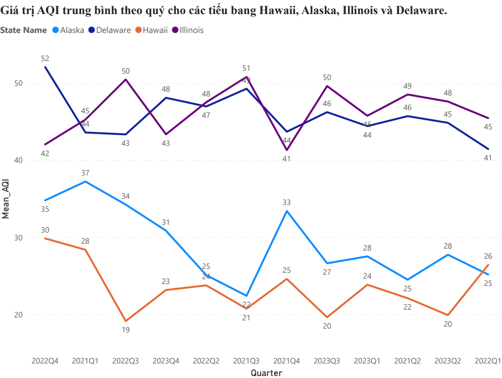
Hình 20: Giá trị AQI trung bình theo quý cho 4 tiểu bang.
