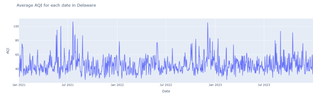
Hình 28: AQI trung bình của Delaware theo thời gian
