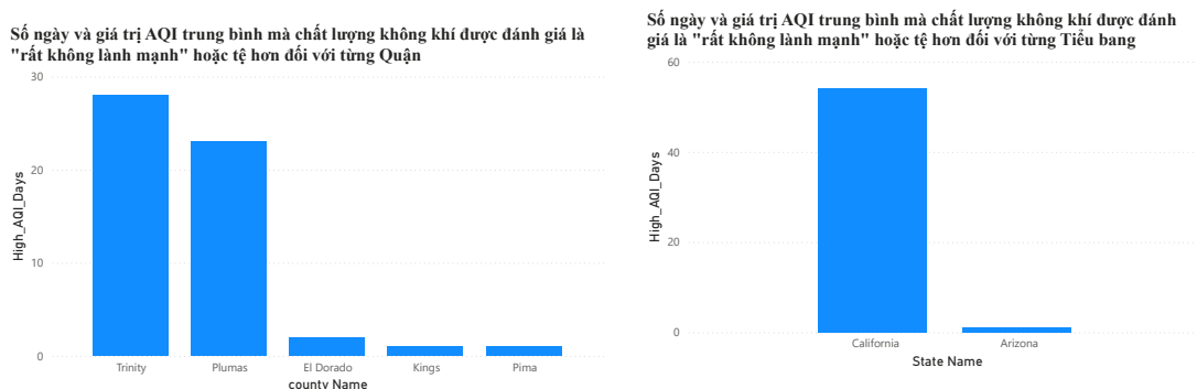
Hình 18: Số ngày và giá trị AQI trung bình với chất lượng không khí "rất không lành mạnh" hoặc tệ hơn.
