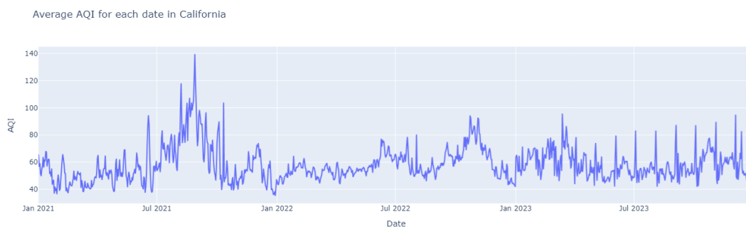
Hình 25: AQI trung bình của California theo thời gian
