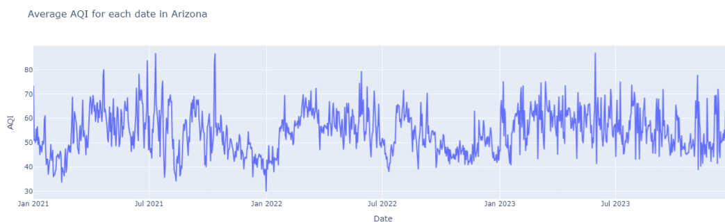
Hình 24: AQI trung bình của Arizona theo thời gian
