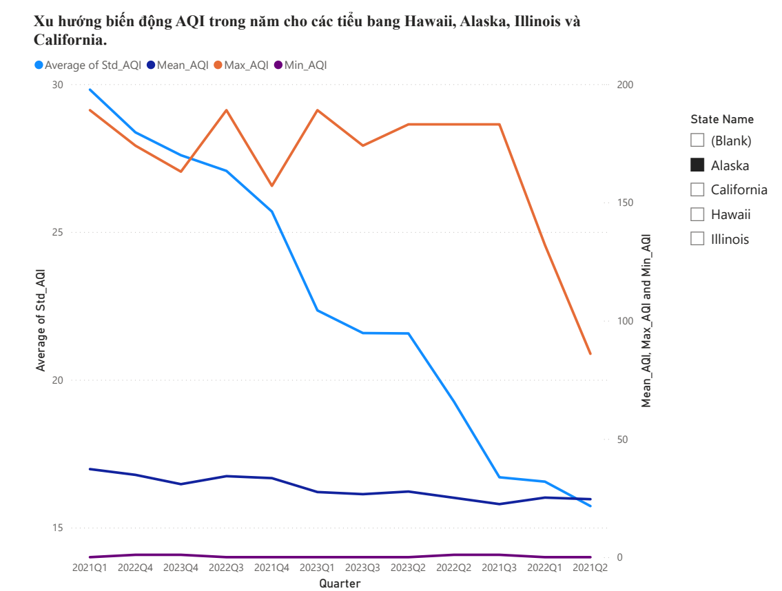
Hình 21: Xu hướng biến động AQI trong năm cho 4 tiểu bang.
