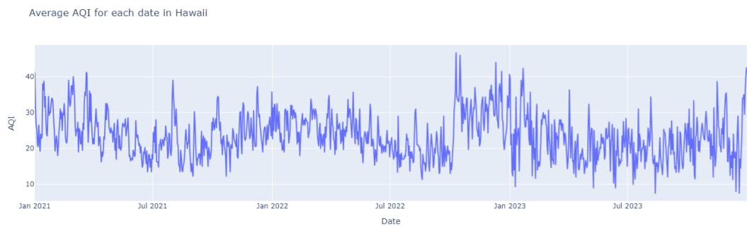
Hình 29: AQI trung bình của Hawaii theo thời gian
