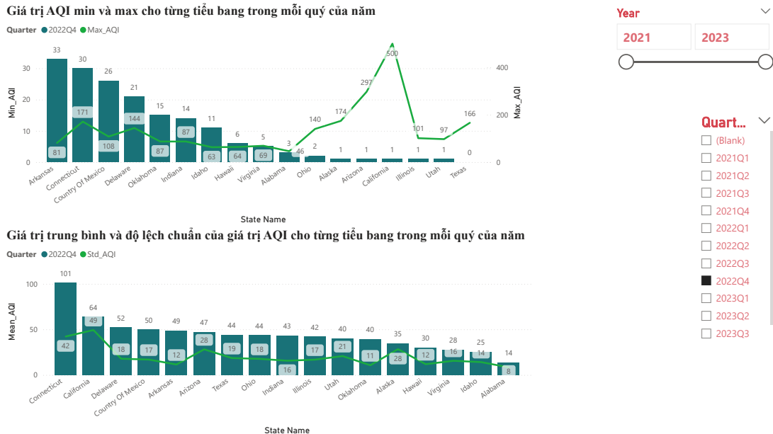
Hình 17: Biểu đồ thể hiện giá trị AQI min, max, trung bình và độ lệch chuẩn của các tiểu bang trong từng quý.
