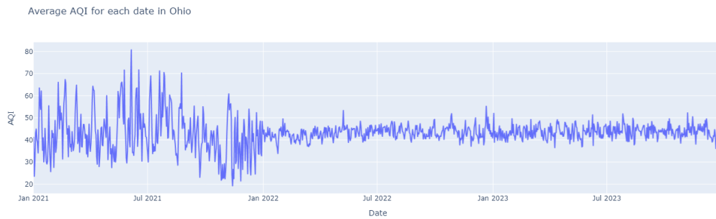
Hình 32: AQI trung bình của Ohio theo thời gian
