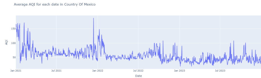
Hình 27: AQI trung bình của Country of Mexico theo thời gian
