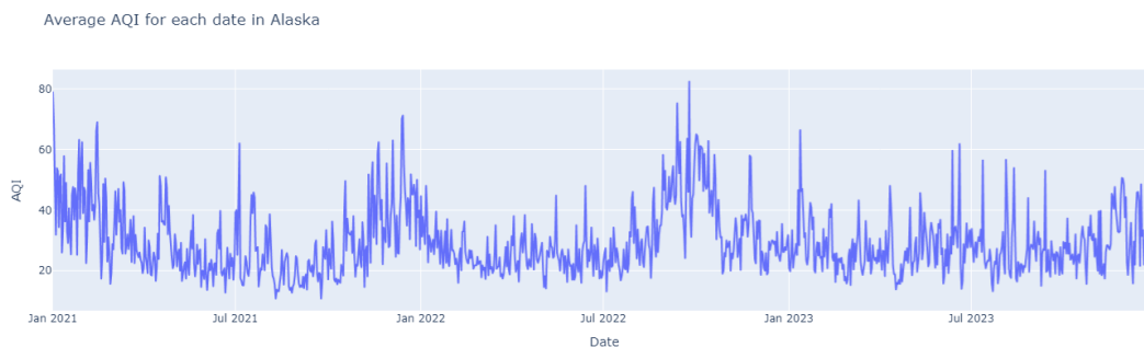
Hình 23: AQI trung bình của Alaska theo thời gian
