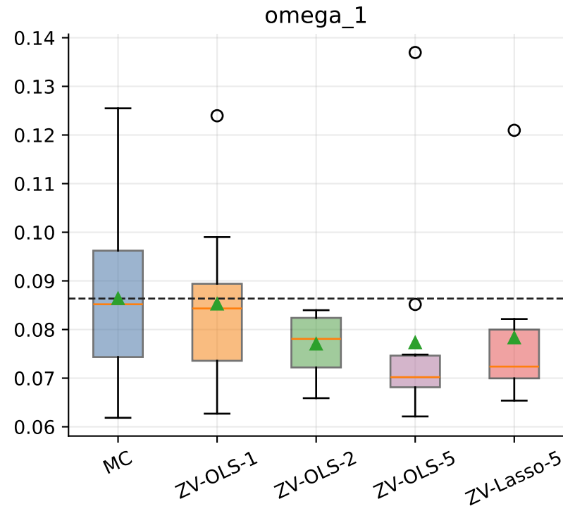
Repeated-run posterior mean estimates: eurUSD
