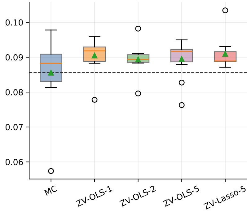
Repeated-run posterior mean estimates: eurUSD
