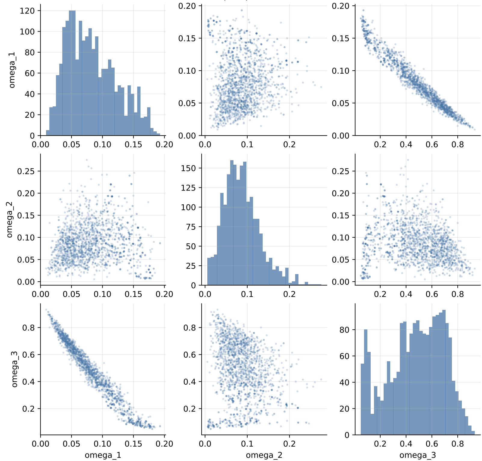
Posterior pair plots: eurUSD
