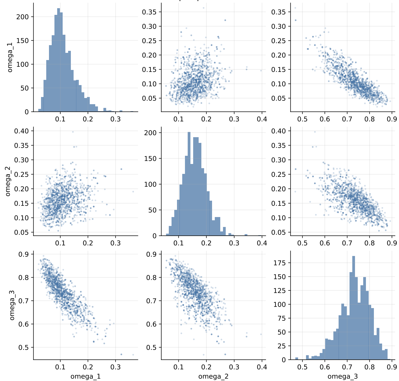
Posterior pair plots: simulated
