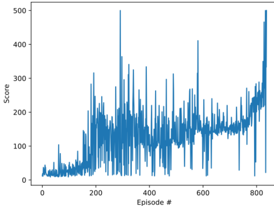
Hình 1.7: Learning Curve của DQN trên môi trường CartPole-v1
