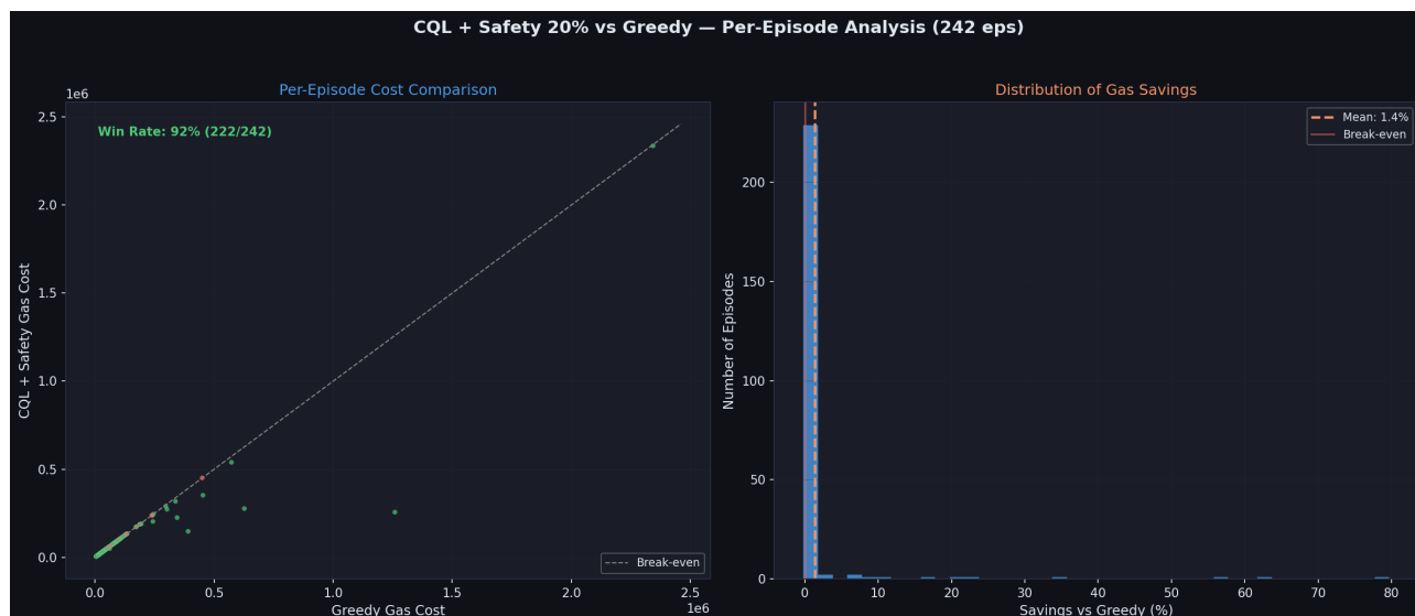
Hình 2.7: Trái: Scatter plot so sánh Gas Cost từng episode (CQL vs Greedy). Điểm xanh: CQL thắng; điểm đỏ: CQL thua. Hầu hết điểm nằm dưới đường break-even. Phải: Phân phối mức tiết kiệm (%). CQL tiết kiệm trung bình 1.4% mỗi episode, với một số episodes đạt tới 79.7%.
