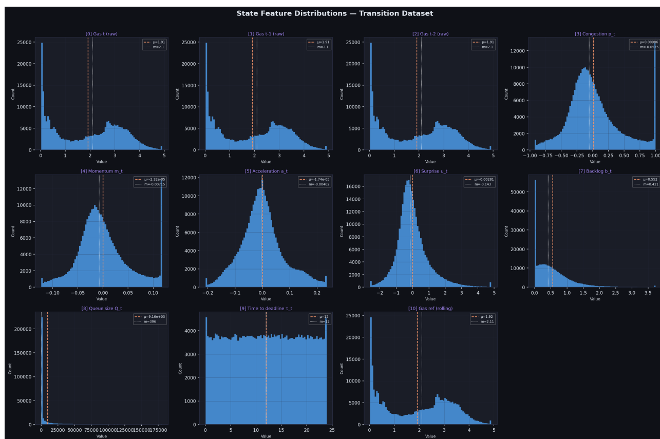
Hình 2.1: Phân phối 11 đặc trưng trạng thái trong tập dữ liệu. Đường cam nét đứt: giá trị trung bình ( \mu ); đường trắng chấm: trung vị ( m ). Các đặc trưng g_t , g_{t-1} , g_{t-2} (giá gas) có phân phối bimodal phản ánh 2 chế độ thị trường (thanh khoản thấp và cao).
