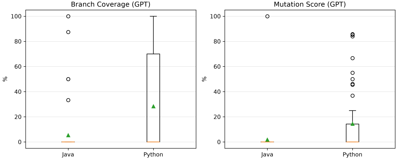
Phan phối chất lượng test GPT (CC 5-10)
