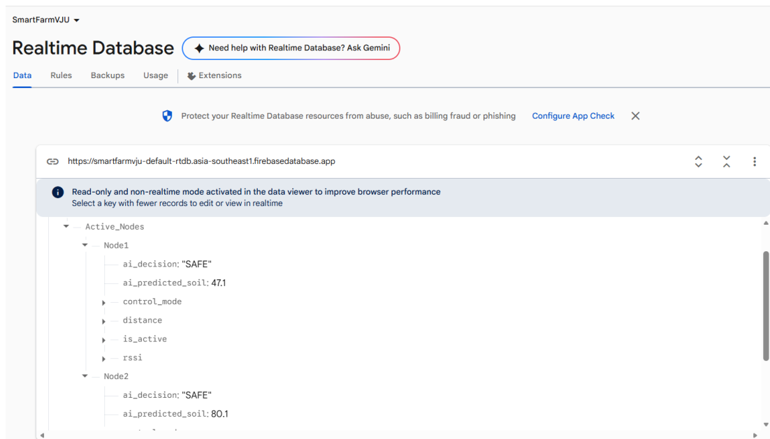
Hình 7.22. Chạy AI Inference để dự đoán giá trị độ ẩm đất và phân loại quyết định (giá trị độ ẩm đất dự đoán được đẩy lên lưu vào firebase đồng thời phân loại quyết định điều khiển tương ứng)
