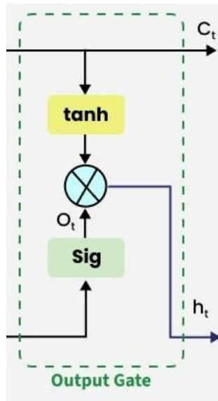
Hình 3.17. Output gate
