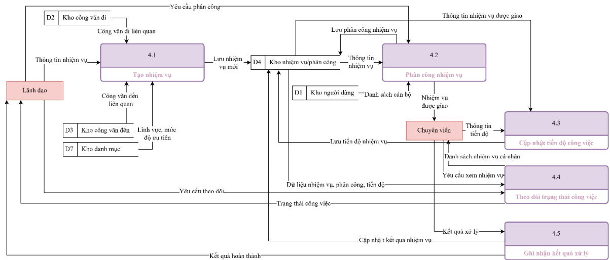
Hình 3.11 DFD mức 2 – 4.0 Quản lý phân công công việc
