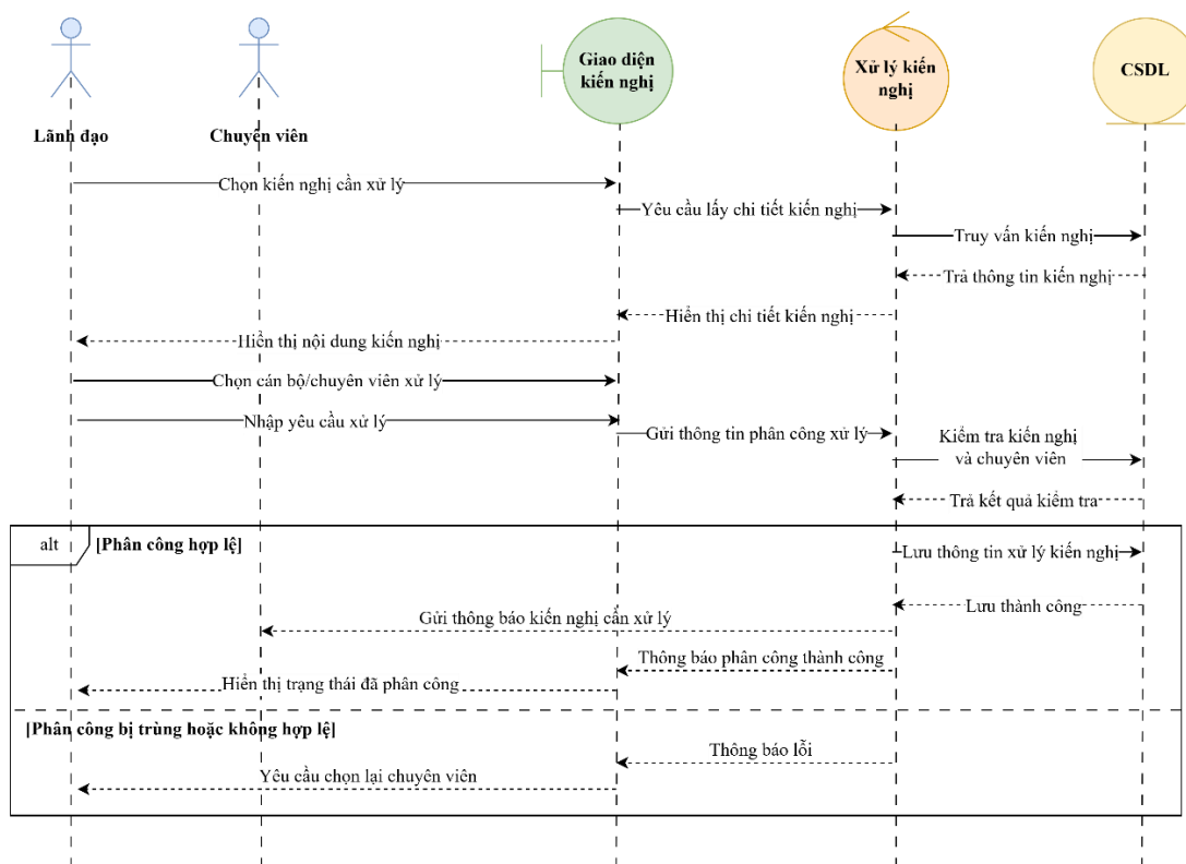
Hình 3.27 Lược đồ tuần tự UC28 – Phân công xử lý kiến nghị
