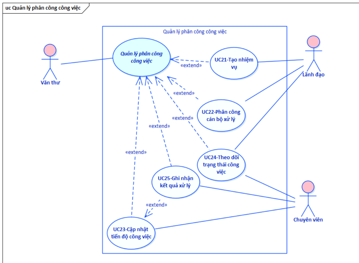
Hình 3.20 Sơ đồ Use Case Quản lý phân công công việc
