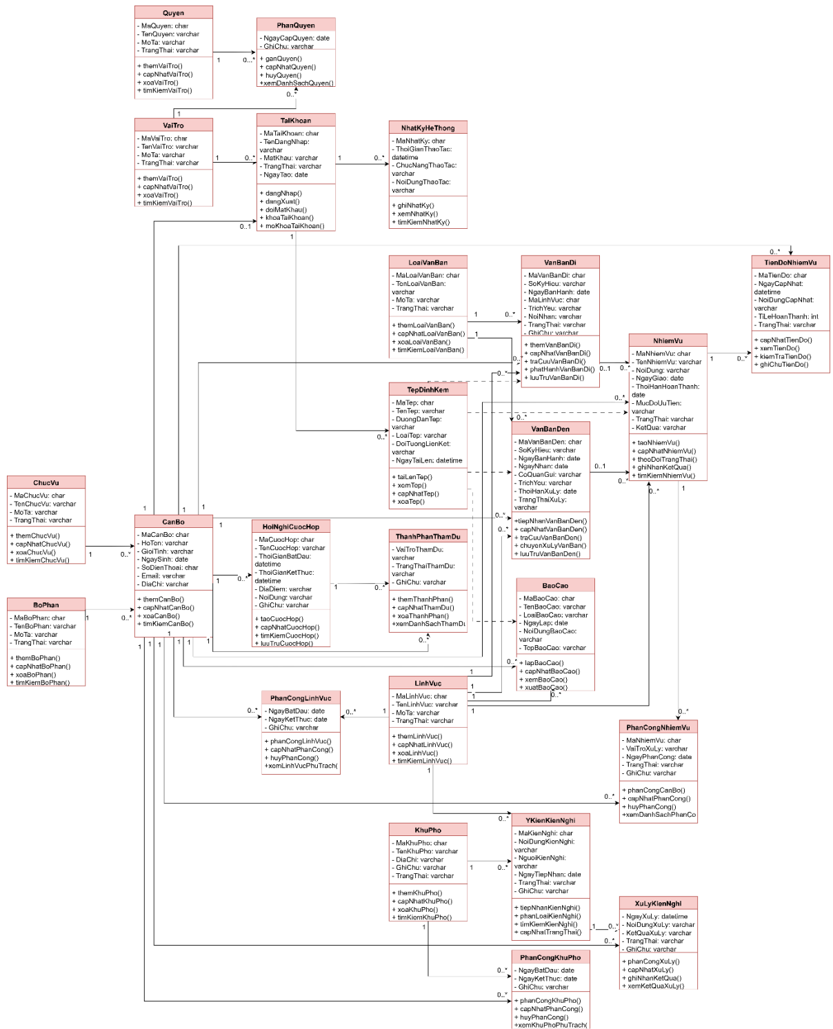
Hình 3.15 Sơ đồ lớp UML
