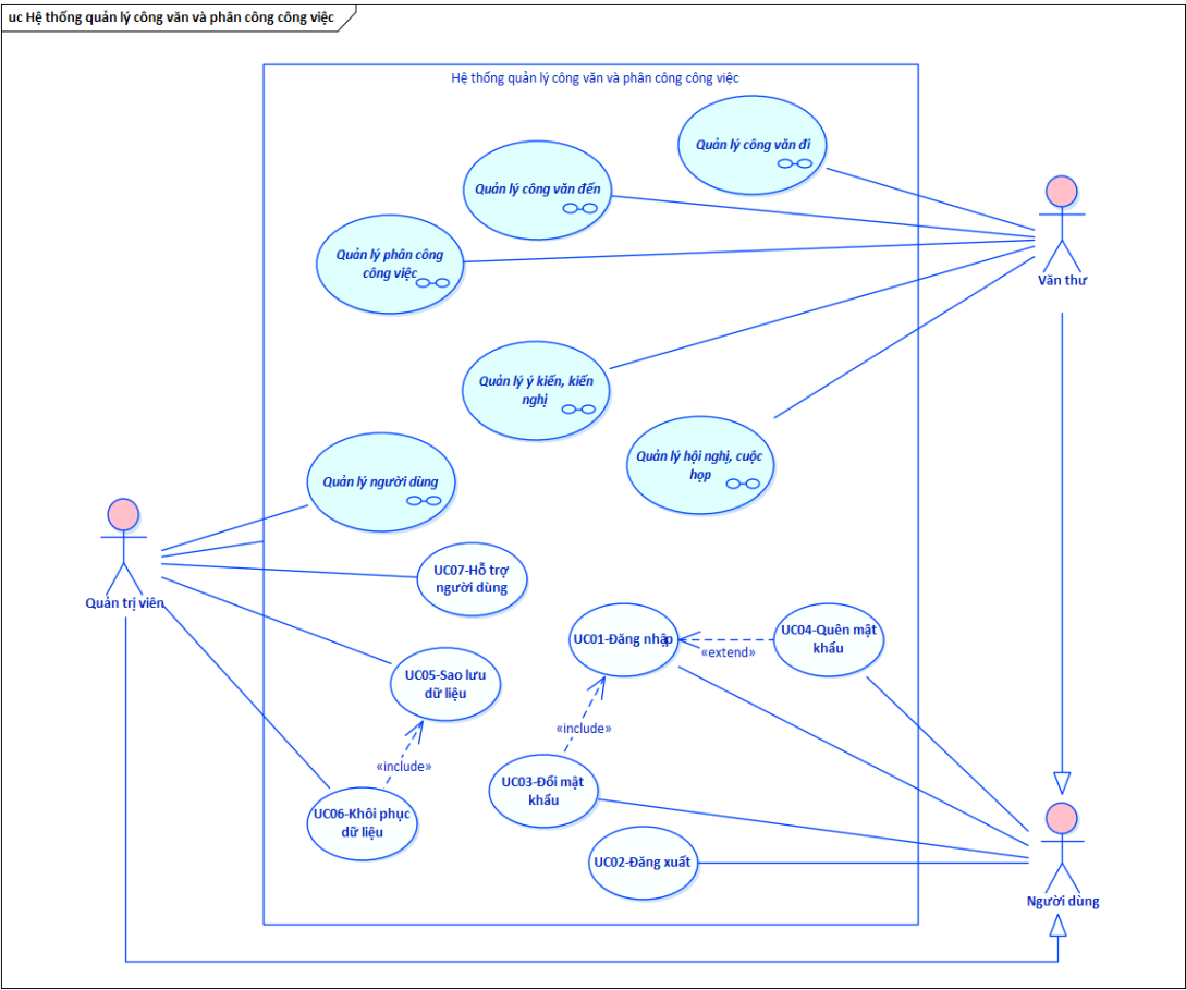
Hình 3.16 Sơ đồ Use case mức tổng thể
