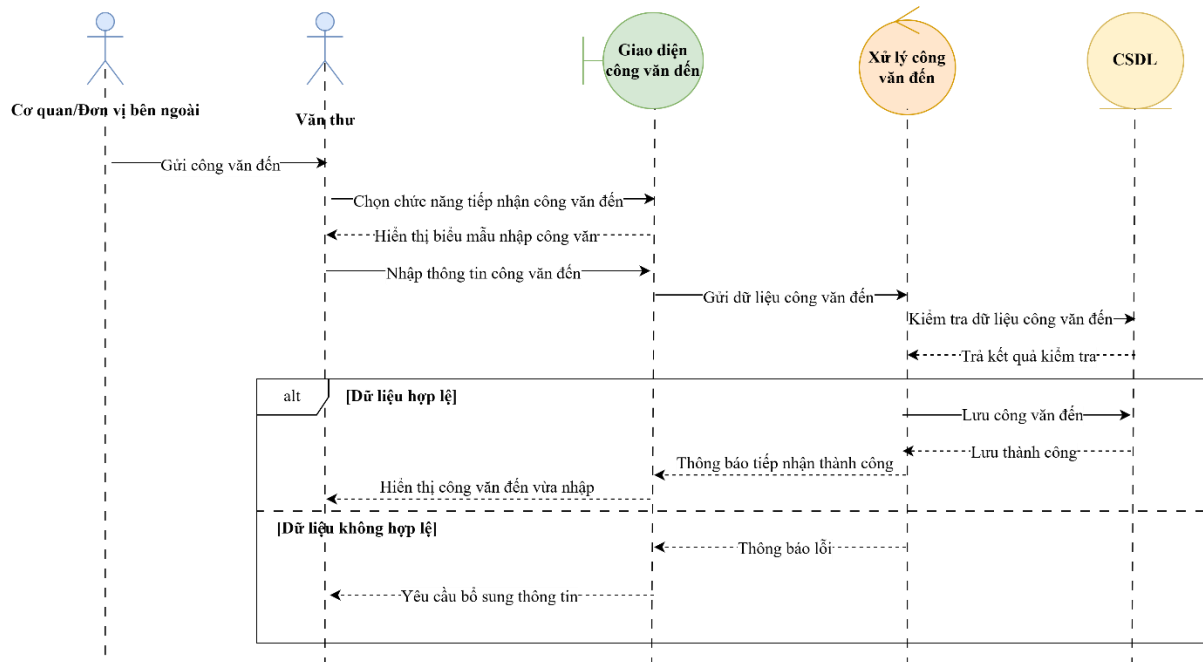
Hình 3.25 Lược đồ tuần tự UC16 – Tiếp nhận công văn đến
