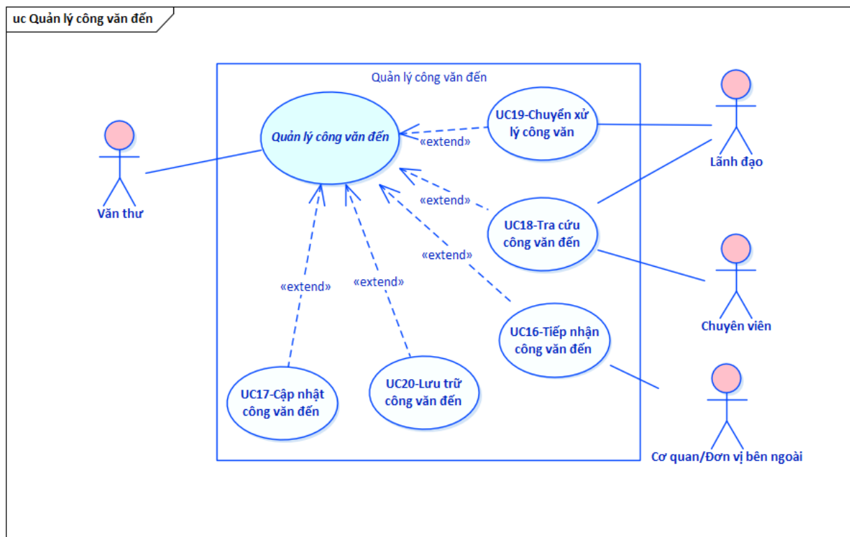
Hình 3.19 Sơ đồ Use Case Quản lý công văn đến
