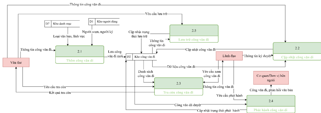
Hình 3.9 DFD mức 2 – 2.0 Quản lý công văn đi
