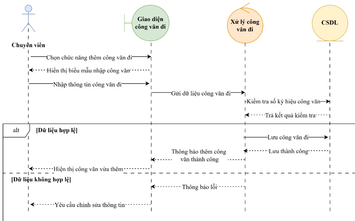
Hình 3.24 Lược đồ tuần tự UC11 – Thêm công văn đi
