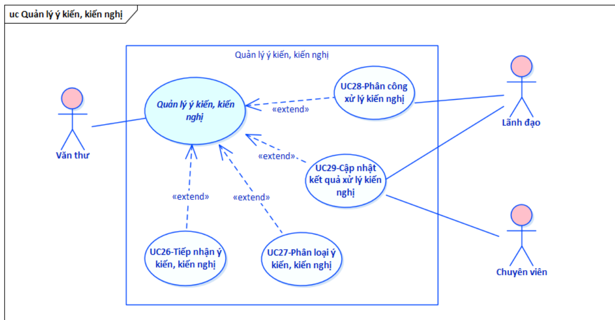
Hình 3.21 Sơ đồ Use Case Quản lý ý kiến, kiến nghị
