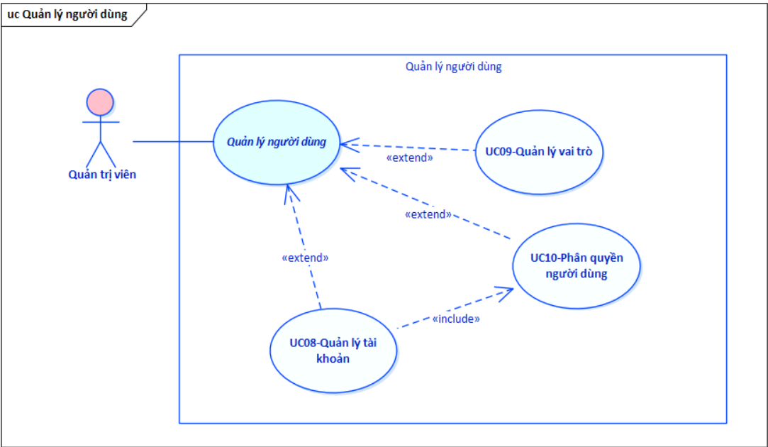
Hình 3.17 Sơ đồ Use Case Quản lý người dùng
