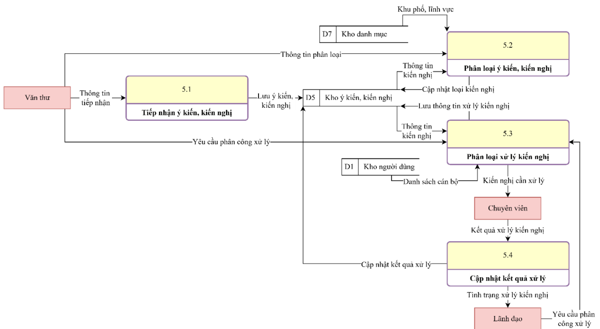
Hình 3.12 DFD mức 2 – 5.0 Quản lý ý kiến, kiến nghị
