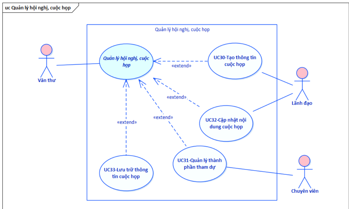
Hình 3.22 Sơ đồ Use Case Quản lý hội nghị, cuộc họp
