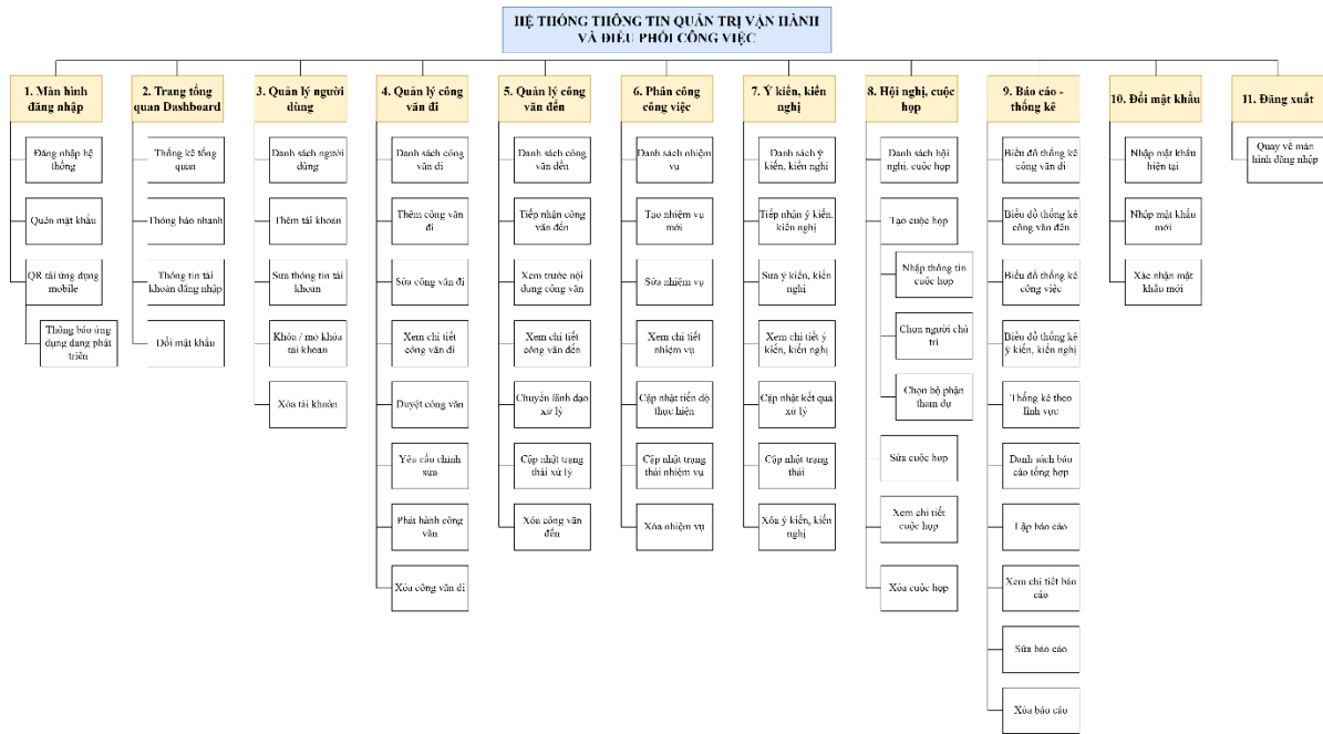
Hình 4.1 Sơ đồ phân cấp giao diện toàn hệ thống
