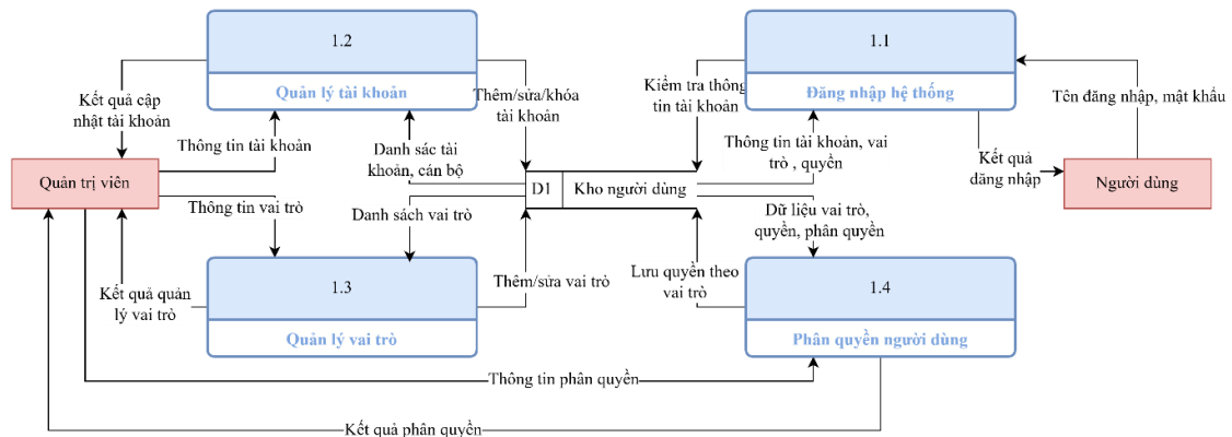
Hình 3.8 DFD mức 2 – 1.0 Quản lý người dùng
