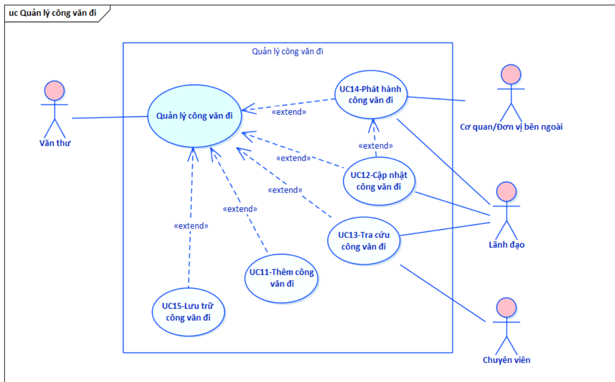
Hình 3.18 Sơ đồ Use Case Quản lý công văn đi
