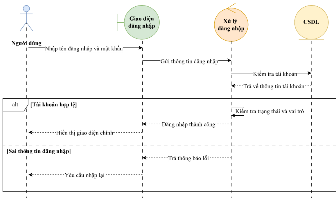
Hình 3.23 Lược đồ tuần tự UC01 – Đăng nhập
