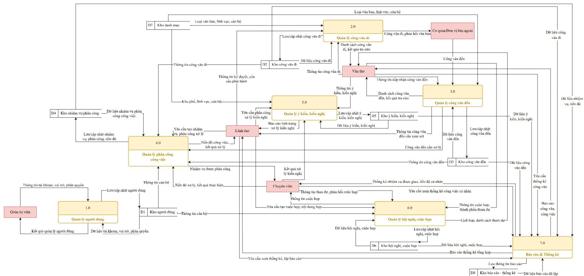
Hình 3.7 DFD mức 1
