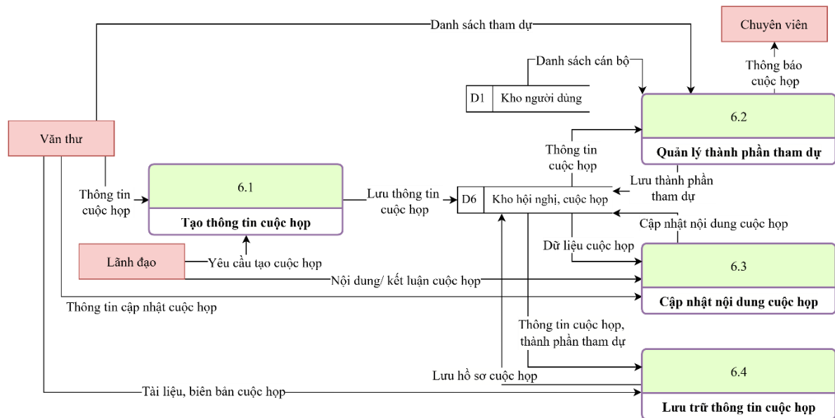
Hình 3.13 DFD mức 2 – 6.0 Quản lý hội nghị, cuộc họp
