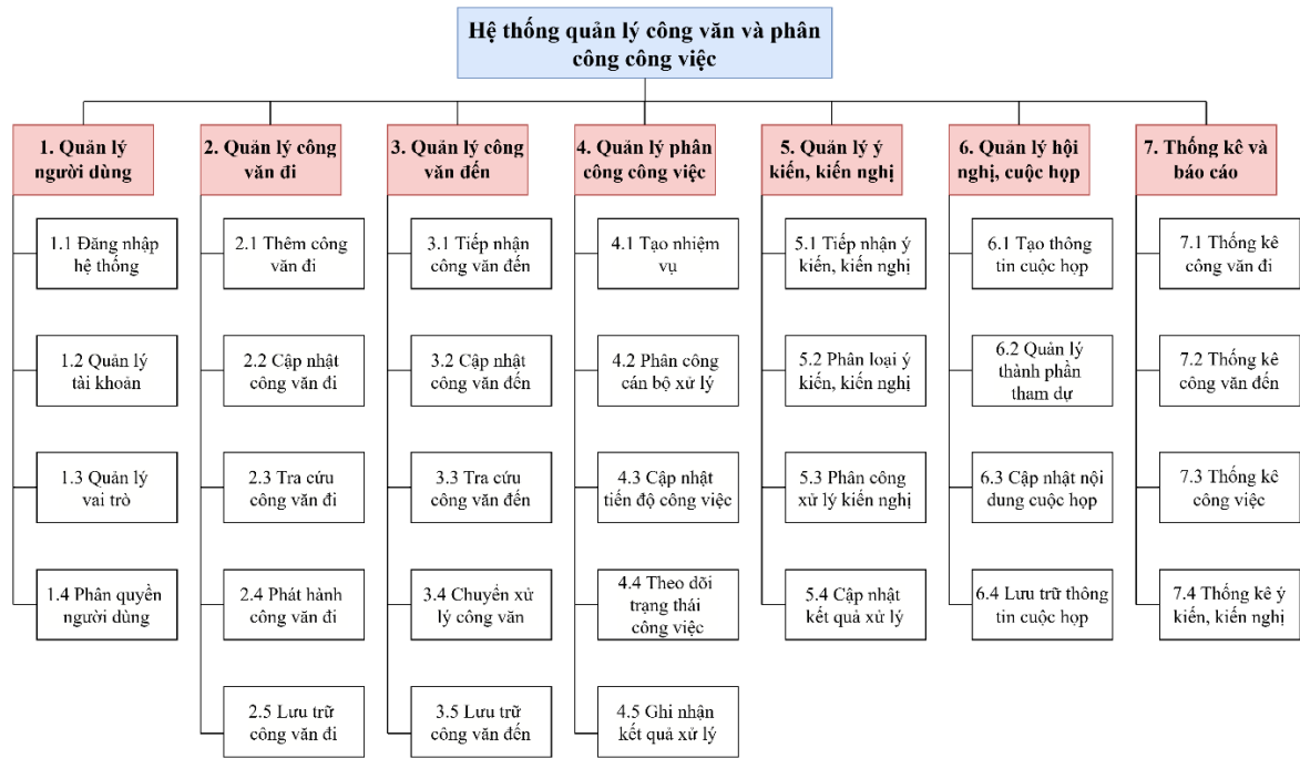
Hình 3.5 Mô hình phân cấp chức năng (BFD)
