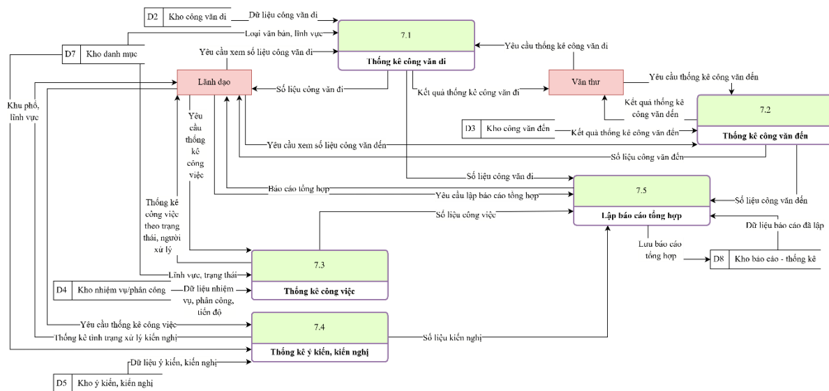
Hình 3.14 DFD mức 2 – 7.0 Quản lý báo cáo – thống kê
