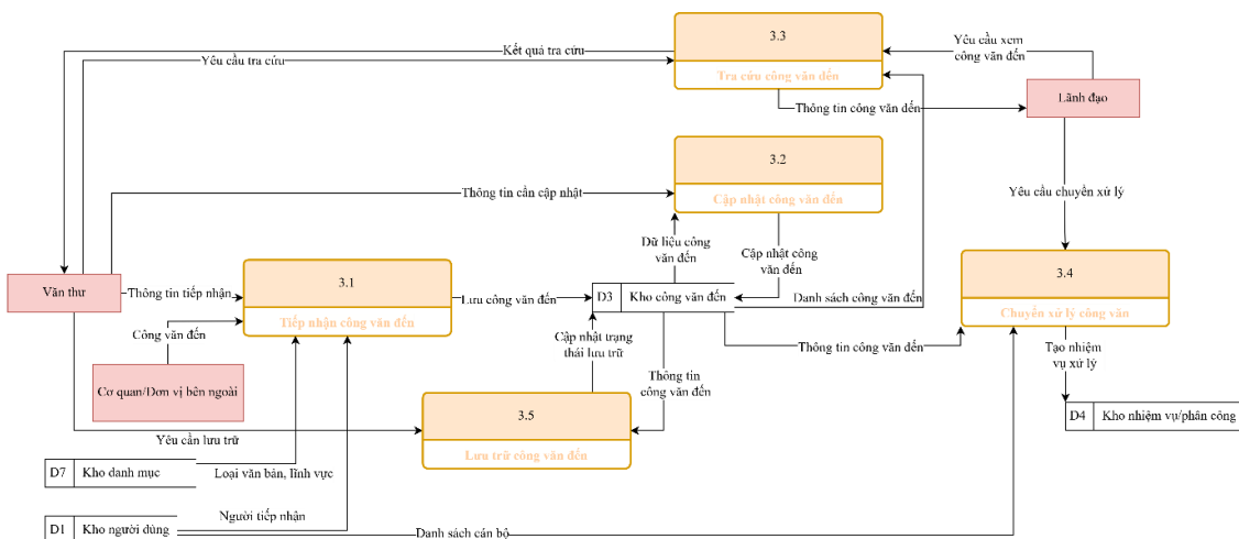
Hình 3.10 DFD mức 2 – 3.0 Quản lý công văn đến
