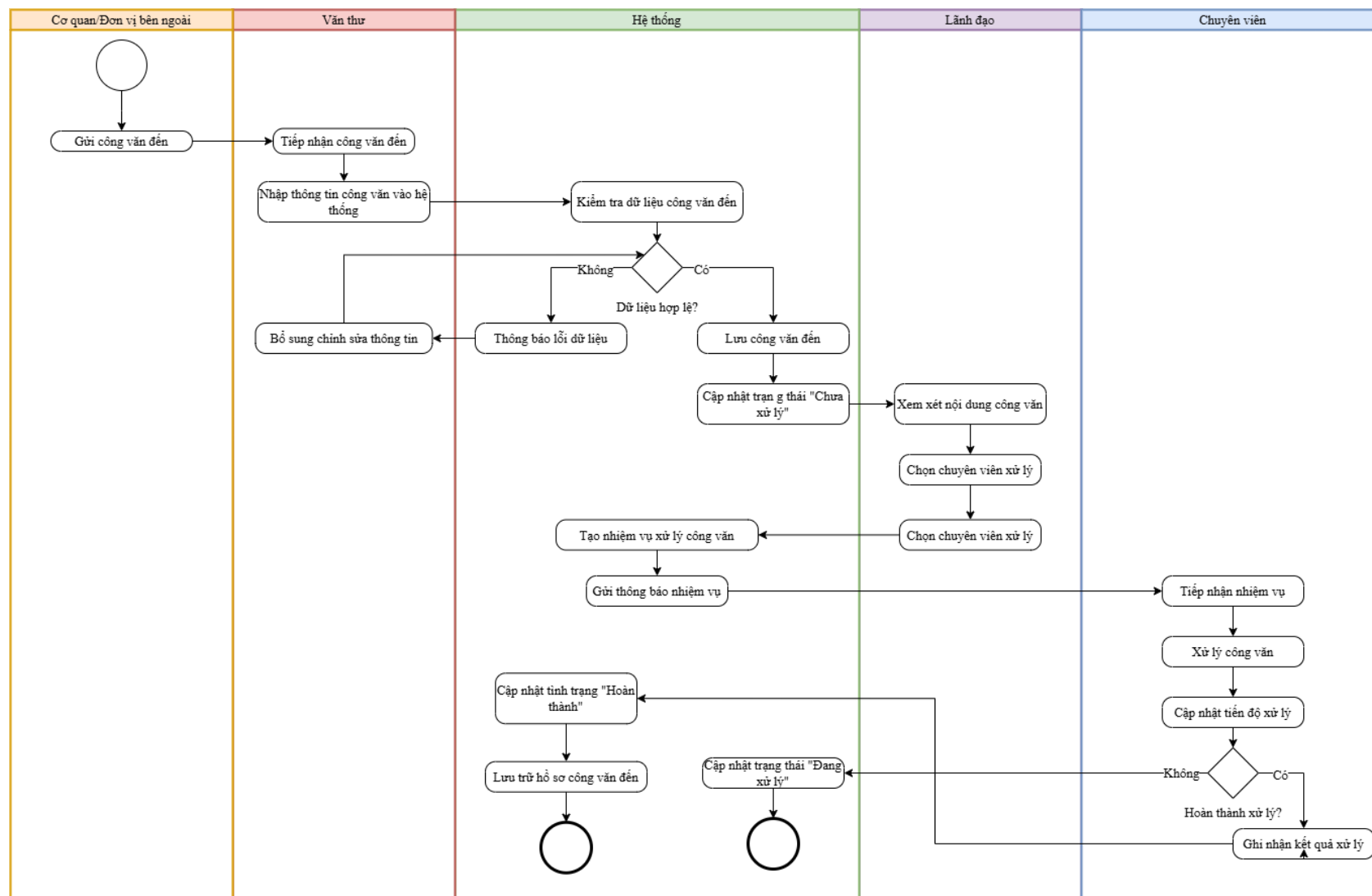
Hình 3.2 Quy trình xử lý công văn đến
