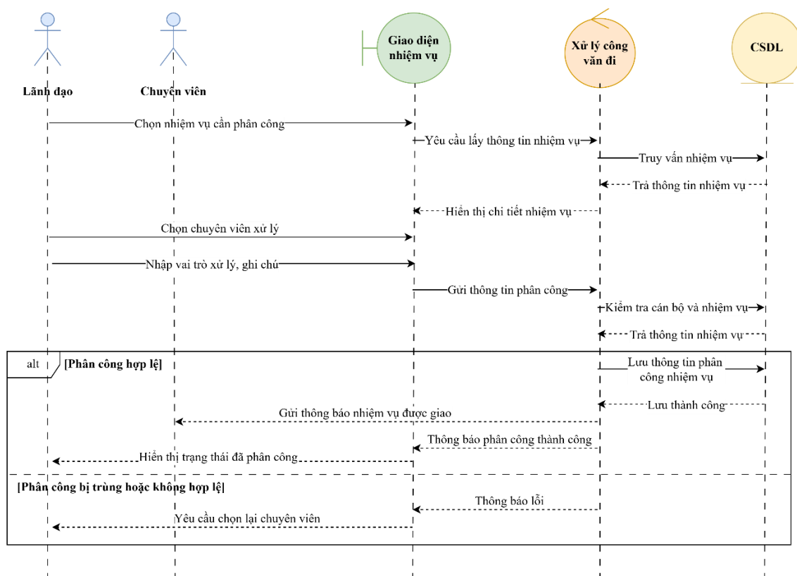
Hình 3.26 Lược đồ tuần tự UC22 – Phân công cán bộ xử lý
