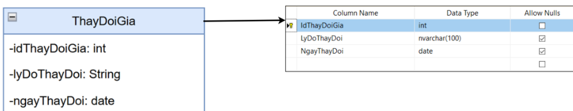
Hình 63. Ảnh xạ thực thể ThayDoiGia
