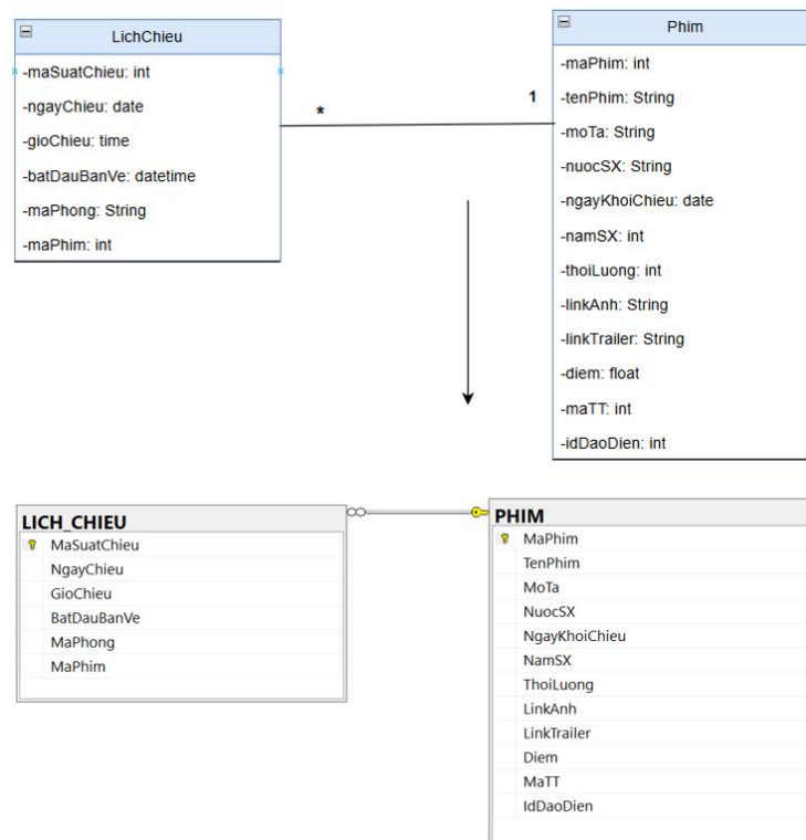
Hình 72. Liên kết thực thể 1-N LichChieu và Phim
