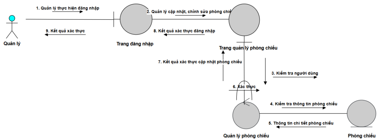
Hình 11. Biểu đồ giao tiếp quản lý phòng chiếu
