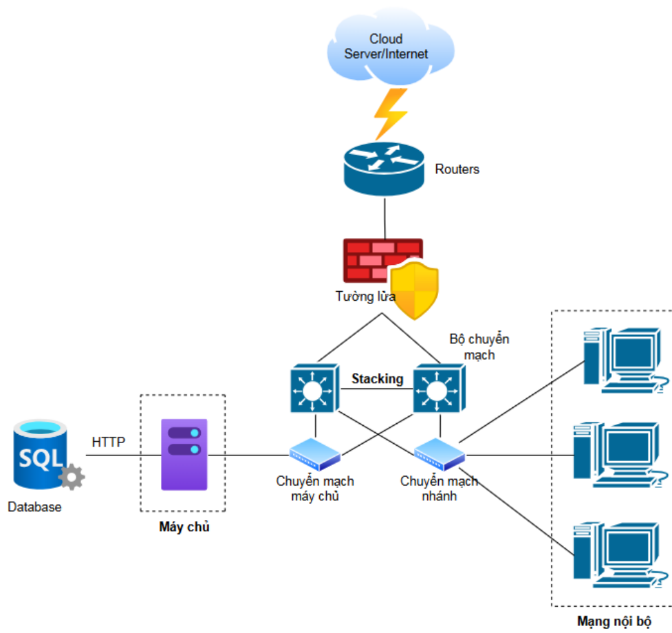
Hình 46. Sơ đồ mạng của hệ thống đặt vé
