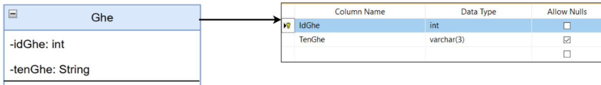
Hình 54. Ảnh xạ thực thể Ghe
