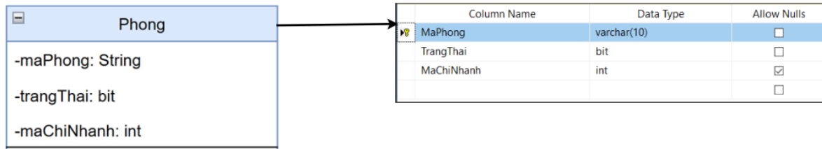
Hình 60. Ảnh xạ thực thể Phong
