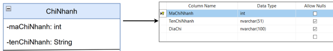
Hình 48. Ánh xạ thực thể ChiNhanh
