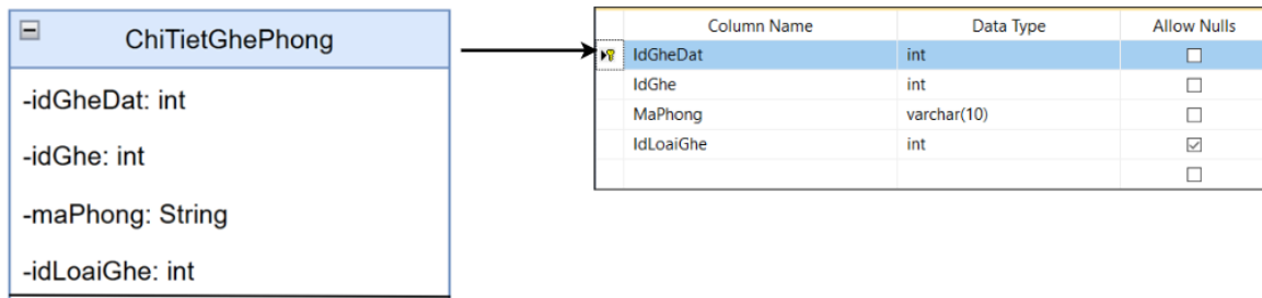
Hình 49. Ánh xạ thực thể ChiTietGhePhong
