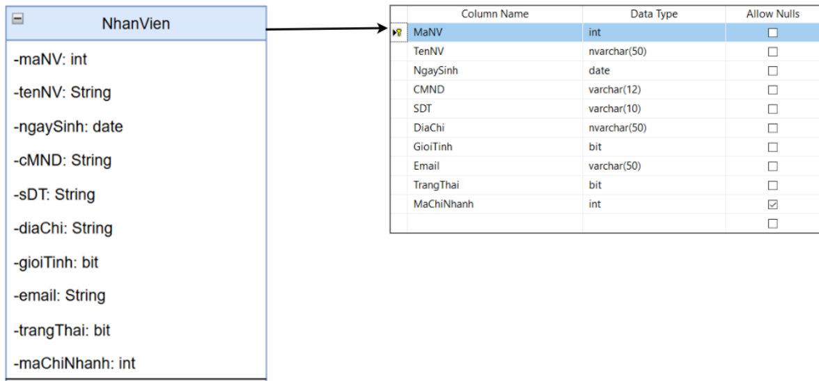
Hình 58. Ảnh xạ thực thể NhanVien
