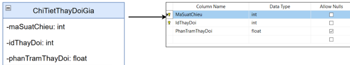
Hình 50. Ảnh xạ thực thể ChiTietThayDoiGia
