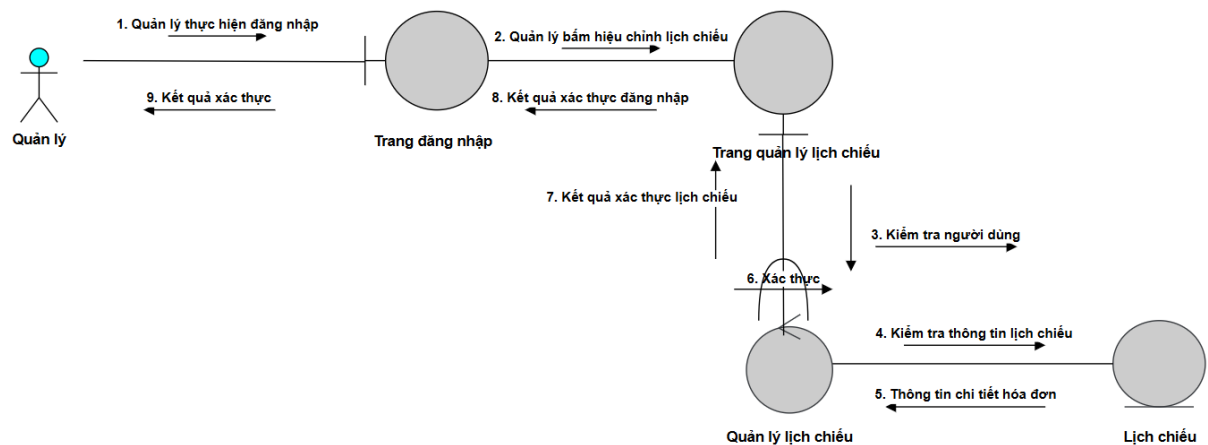
Hình 7. Biểu đồ giao tiếp quản lý lịch chiếu
