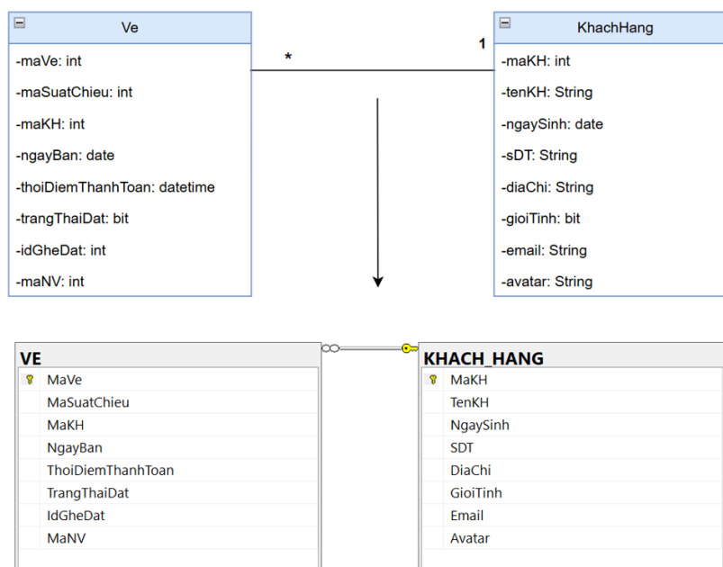
Hình 80. Liên kết thực thể 1-N Ve và KhachHang
