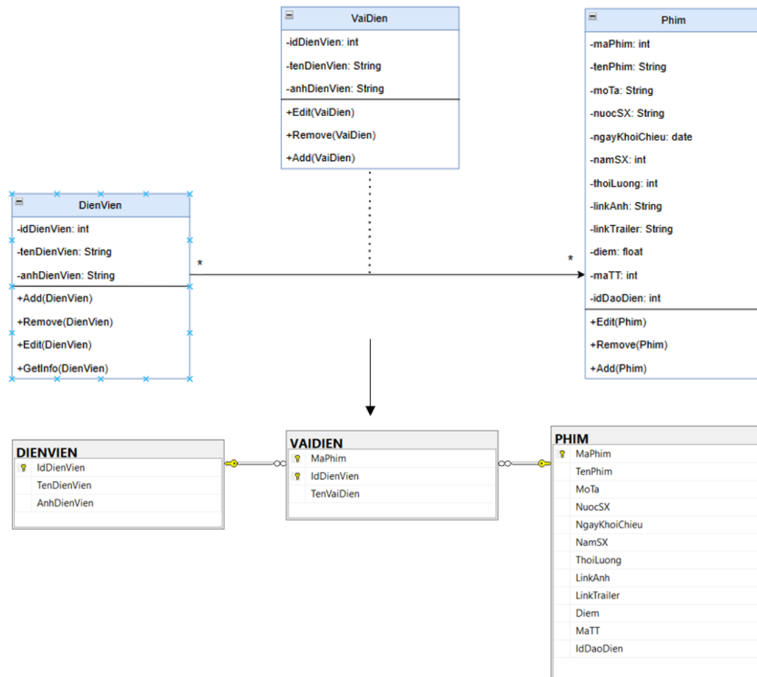
Hình 86. Liên kết thực thể N-N Phim và DienVien
