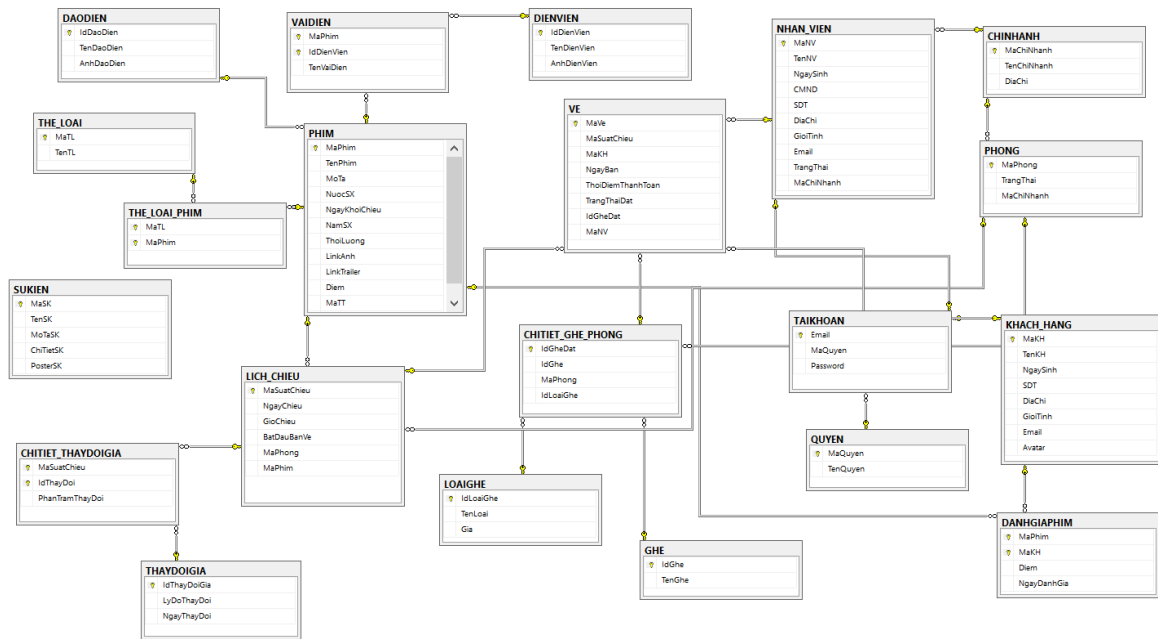
Hình 47: Sơ đồ Diagram của cơ sở dữ liệu
