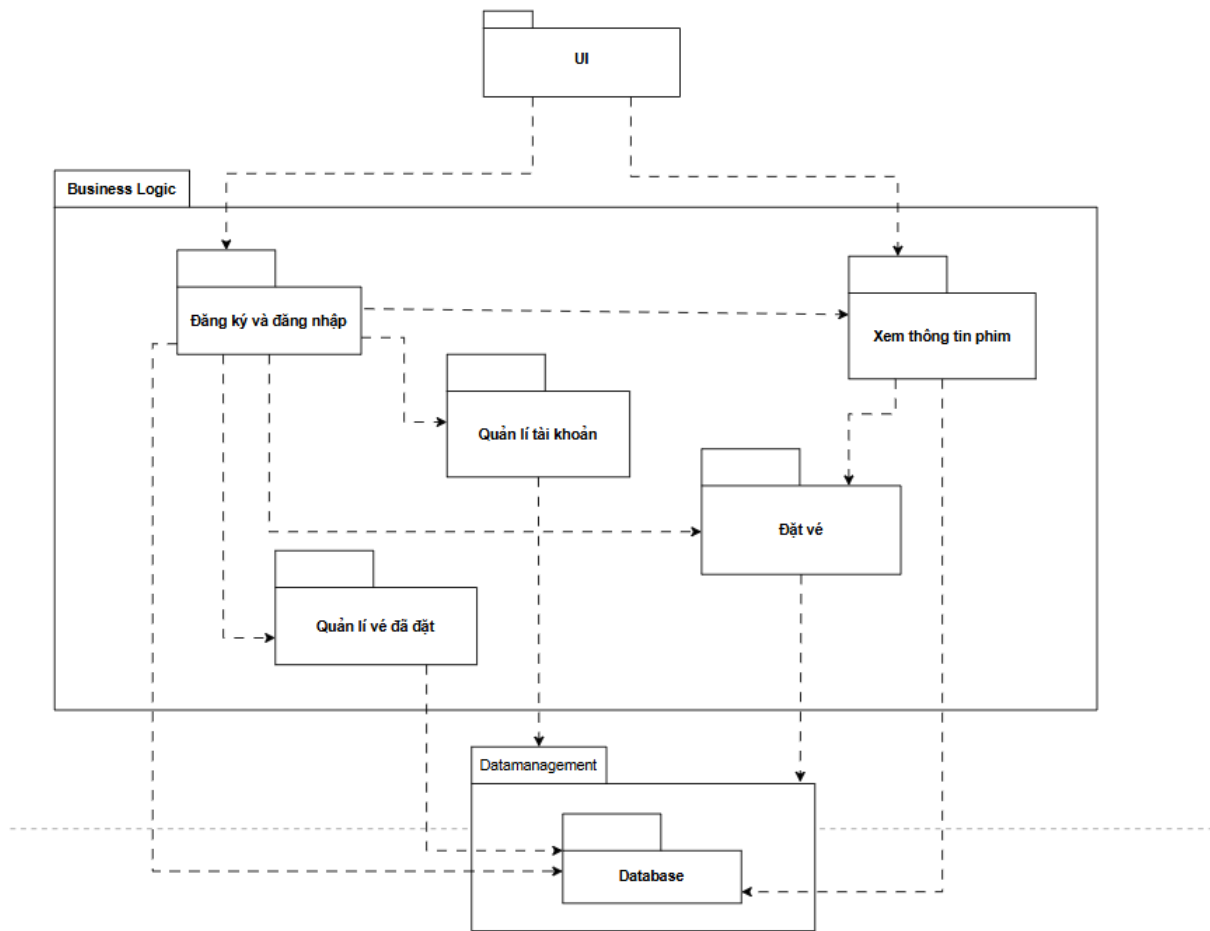
Hình 43. Sơ đồ gói khách hàng
