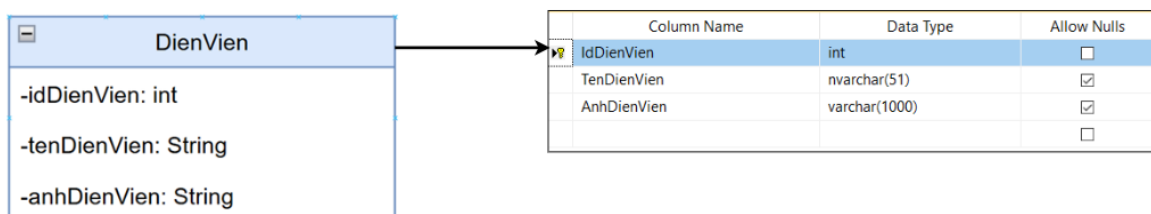
Hình 53. Ảnh xạ thực thể DienVien
