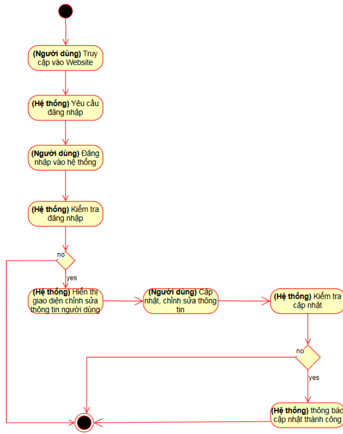
Hình 14. Biểu đồ hoạt động quản lý thông tin người dùng hệ thống
