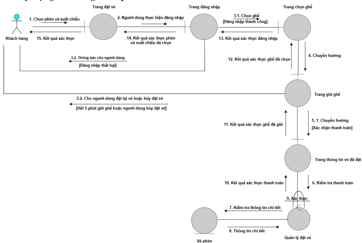
Hình 1. Biểu đồ giao tiếp khách hàng đặt vé xem phim
