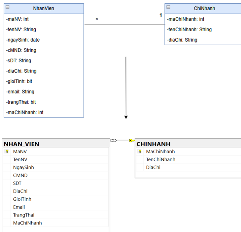
Hình 78. Liên kết thực thể 1-N NhanVien và ChiNhanh
