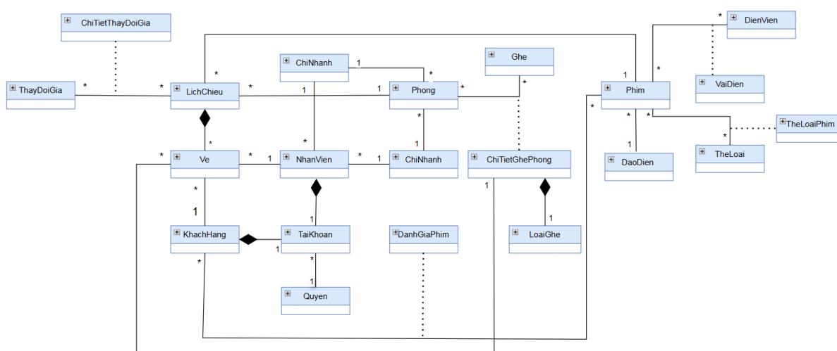
Hình 40. Sơ đồ lớp hệ thống đặt vé xem phim
