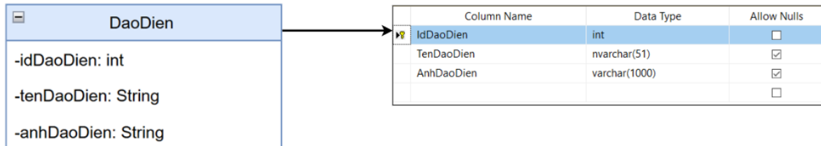
Hình 52. Ảnh xạ thực thể DaoDien
