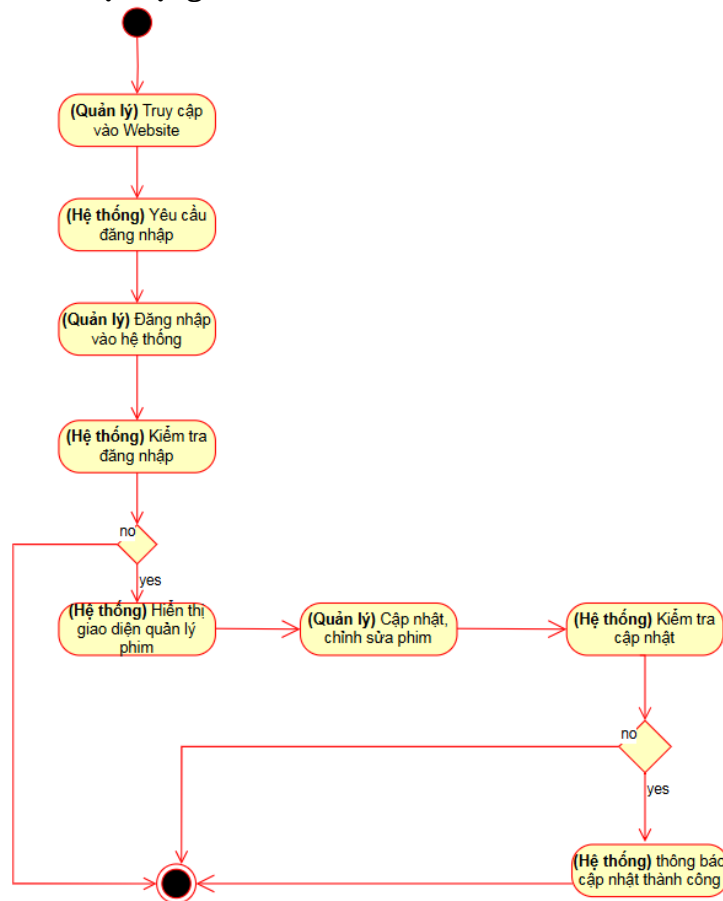
Hình 10. Biểu đồ hoạt động quản lý phim
