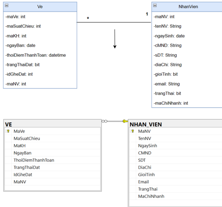
Hình 76. Liên kết thực thể 1-N Ve và NhanVien
