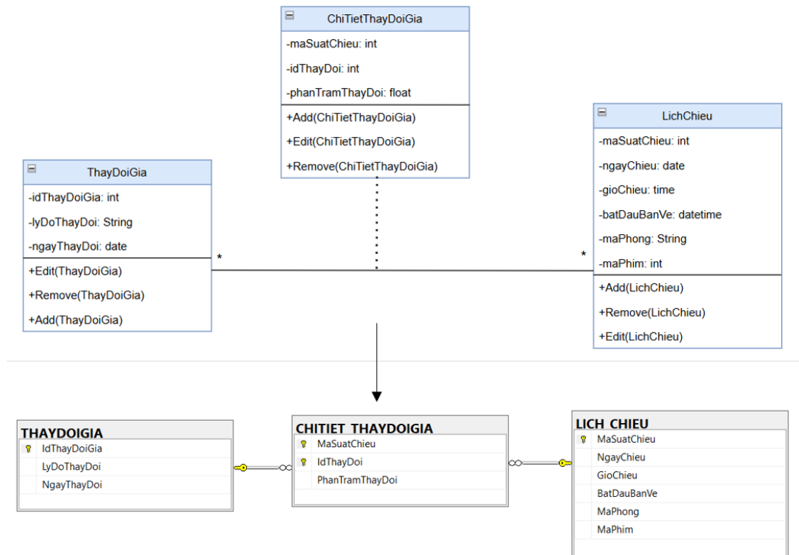
Hình 83. Liên kết thực thể N-N LichChieu và ThayDoiGia
