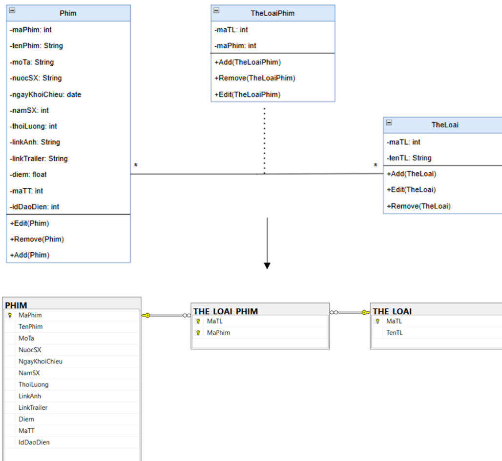
Hình 85. Liên kết thực thể N-N Phim và TheLoai
