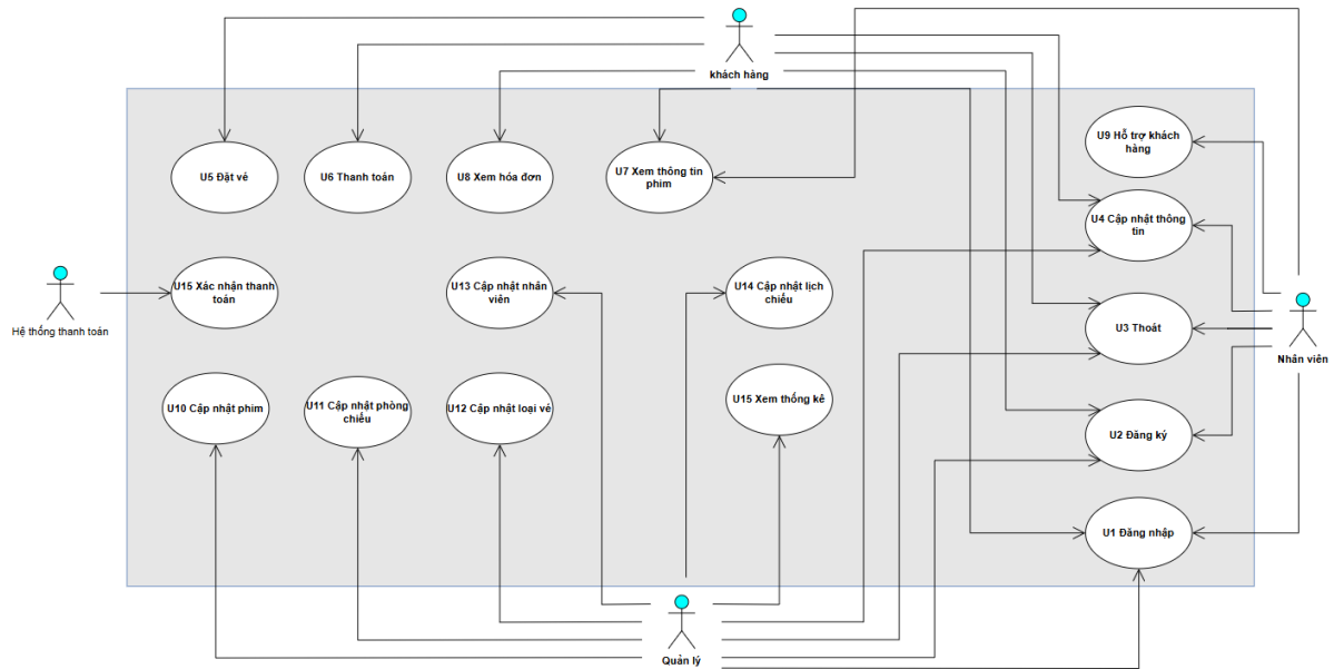
Hình 17. Xác định các ca sử dụng của hệ thống
