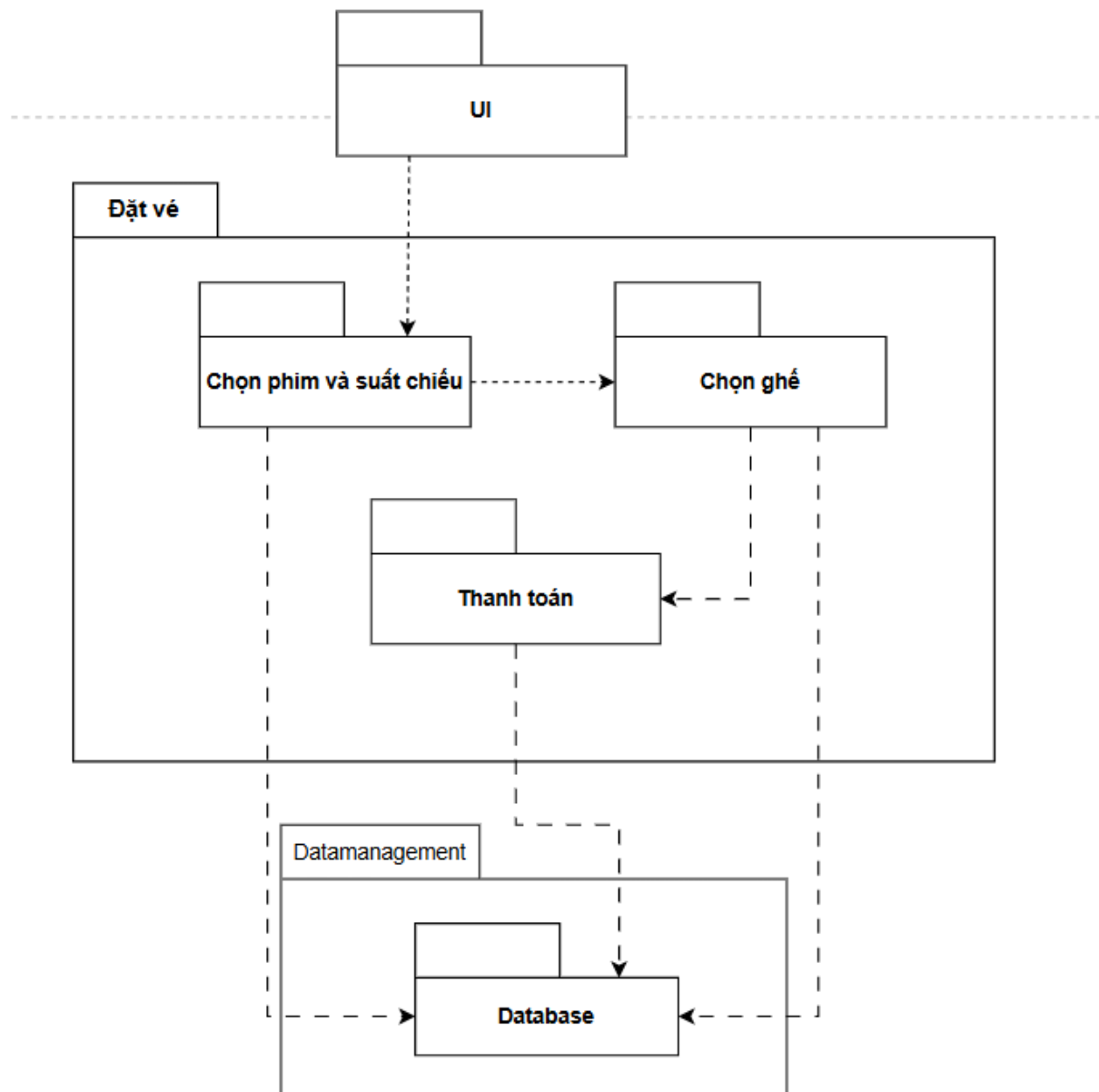
Hình 42. Sơ đồ gói hệ thống đặt vé
