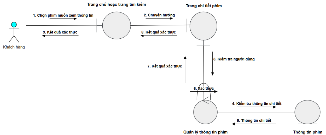
Hình 5. Biểu đồ giao tiếp khách hàng xem thông tin phim
