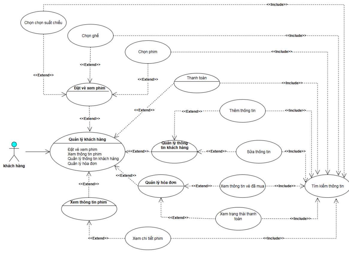
Hình 19. Biểu đồ phân rã ca sử dụng Quản lý khách hàng
