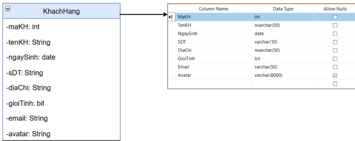
Hình 55. Ảnh xạ thực thể KhachHang
