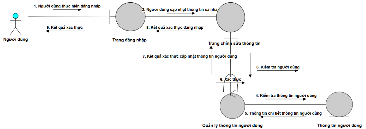
Hình 13. Biểu đồ giao tiếp quản lý thông tin người dùng hệ thống
