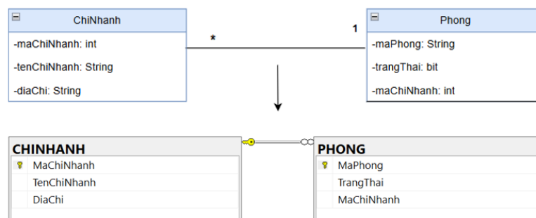
Hình 73. Liên kết thực thể 1-N ChiNhanh và Phong
