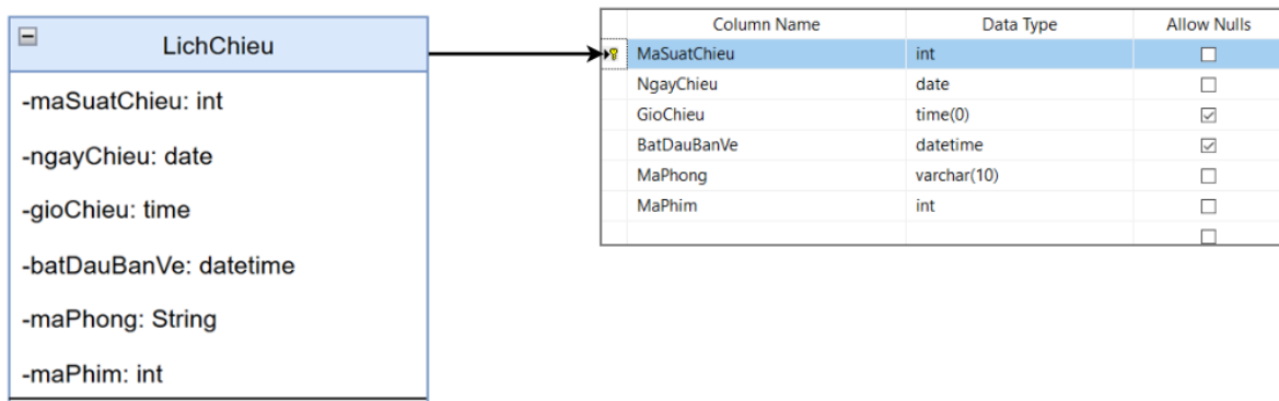
Hình 56. Ảnh xạ thực thể LichChieu
