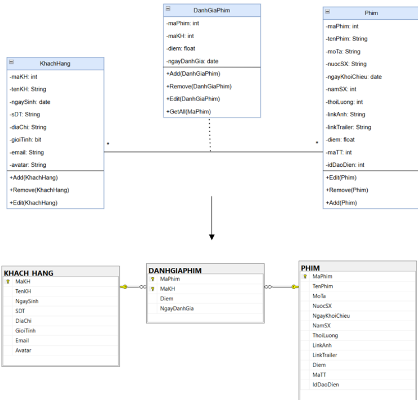
Hình 84. Liên kết thực thể N-N Khách Hàng và Phim
