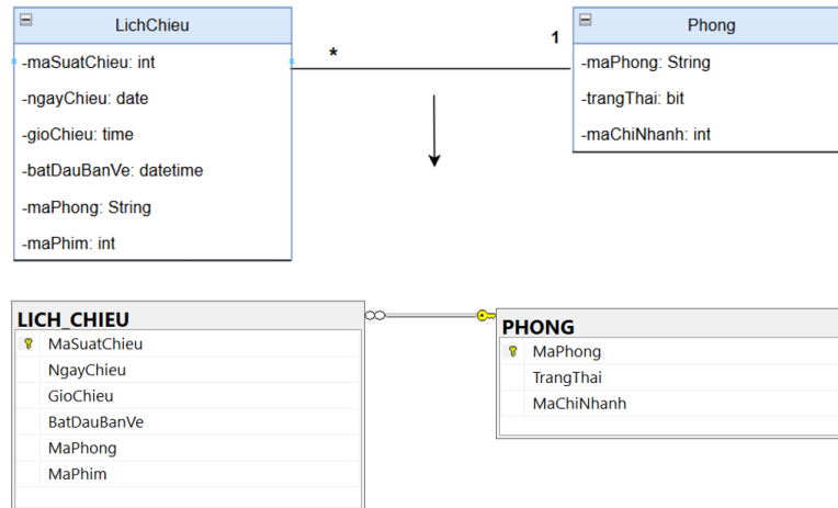
Hình 74. Liên kết thực thể 1-N LichChieu và Phong
