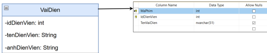
Hình 66. Ảnh xạ thực thể VaiDien
