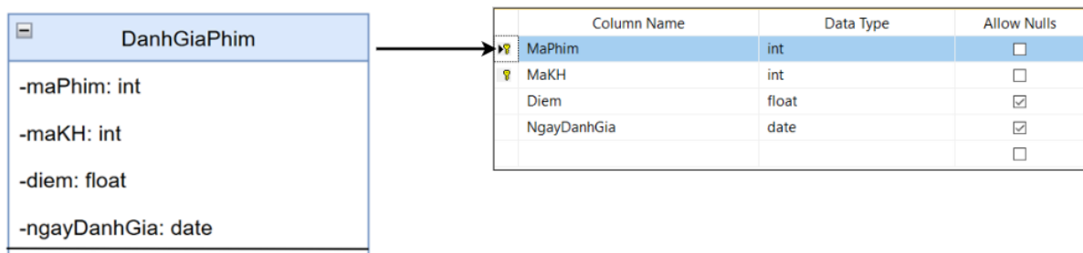
Hình 51. Ảnh xạ thực thể DanhGiaPhim
