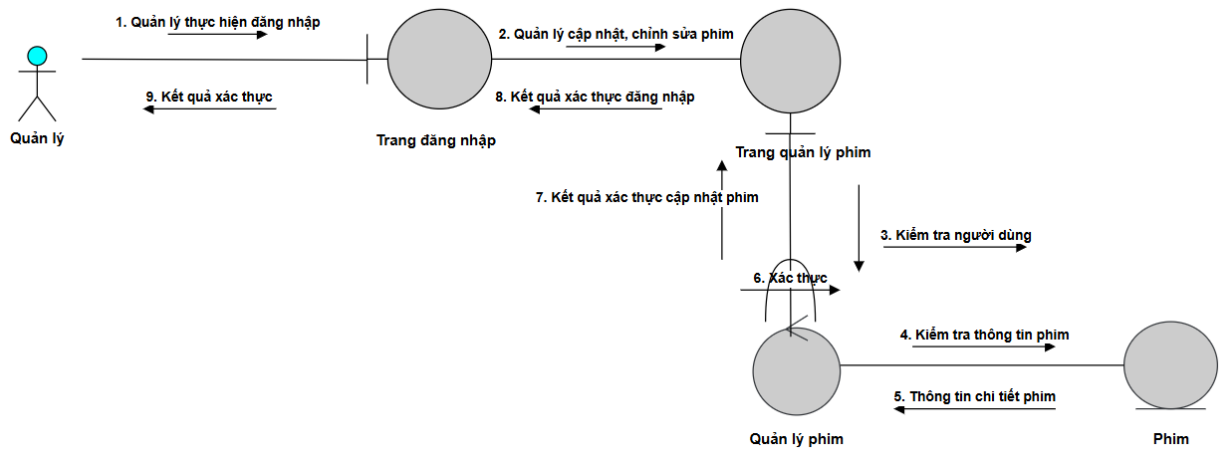
Hình 9. Biểu đồ giao tiếp quản lý phim
