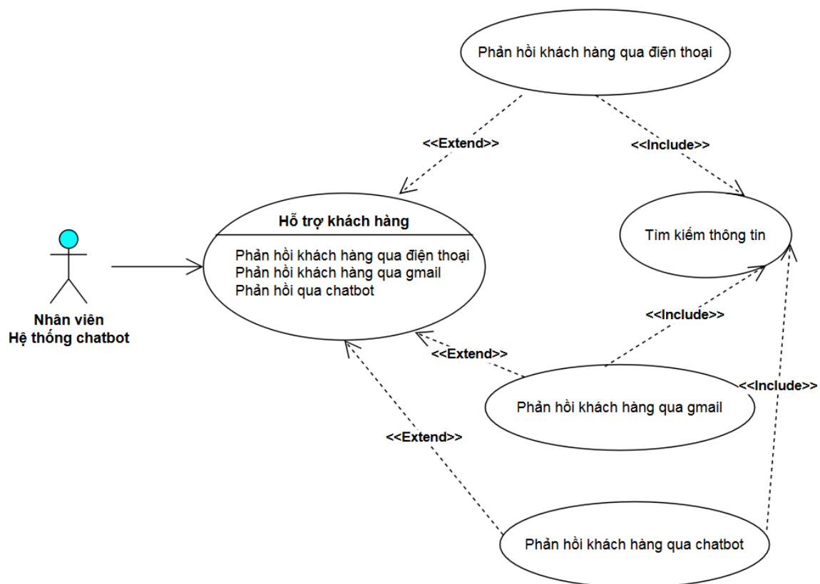
Hình 21. Biểu đồ phân rã ca sử dụng Quản lý hỗ trợ khách hàng
