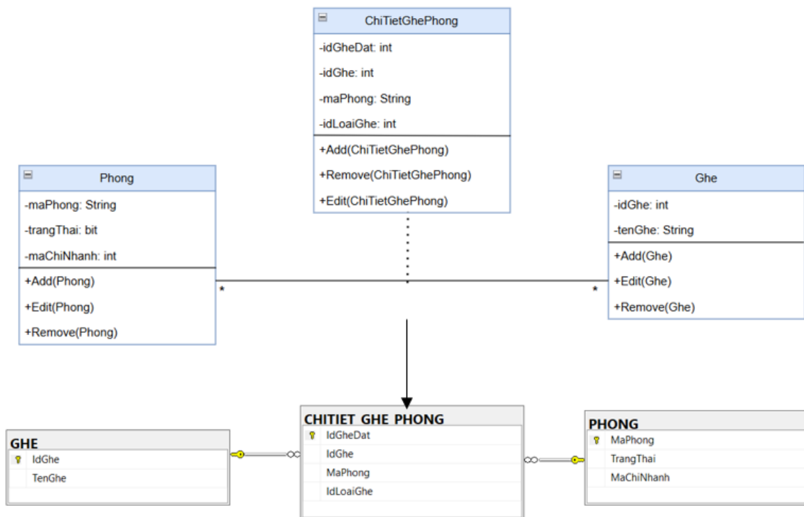
Hình 82. Liên kết thực thể N-N Ghe và Phong
