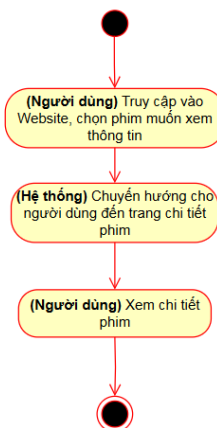
Hình 6. Biểu đồ hoạt động khách hàng xem thông tin phim
