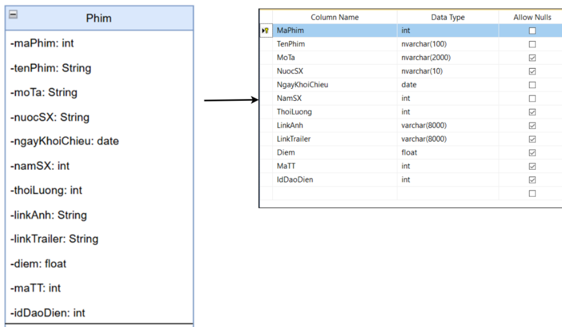
Hình 59. Ảnh xạ thực thể Phim
