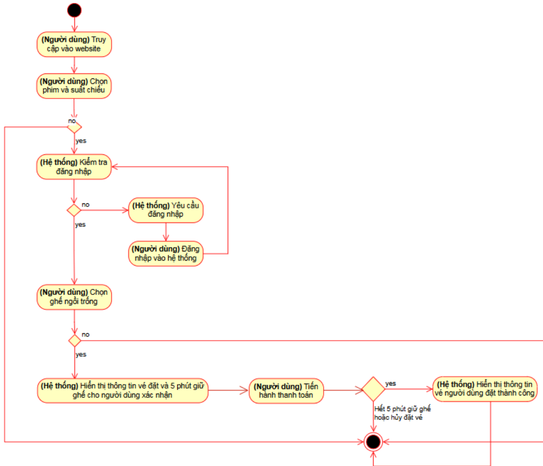
Hình 2. Biểu đồ hoạt động khách hàng đặt vé xem phim
