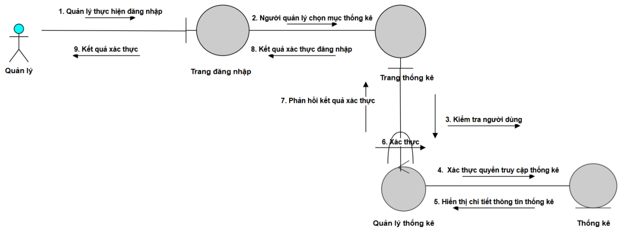
Hình 15. Biểu đồ giao tiếp xem thống kê
