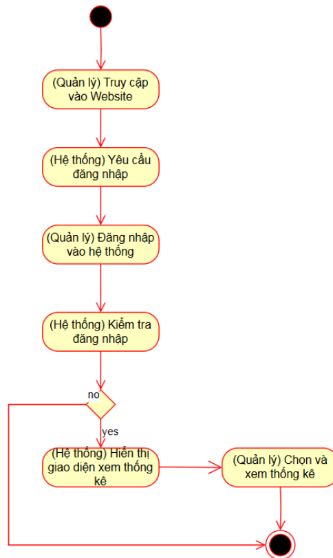
Hình 16. Biểu đồ hoạt động xem thống kê
