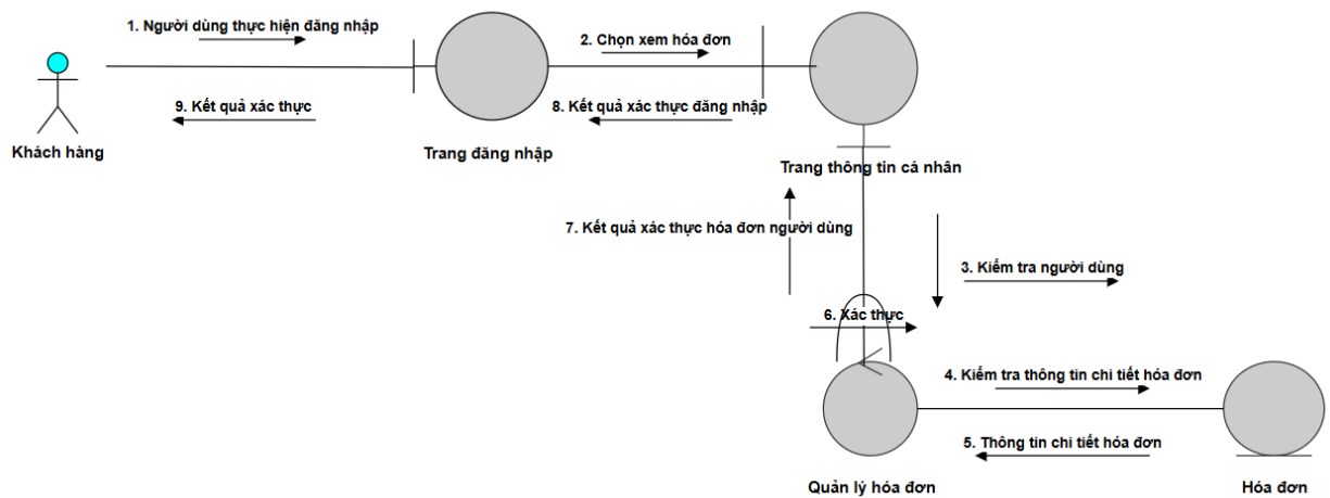
Hình 3. Biểu đồ giao tiếp xem hóa đơn khách hàng
