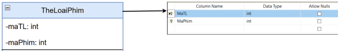
Hình 65. Ảnh xạ thực thể TheLoaiPhim
