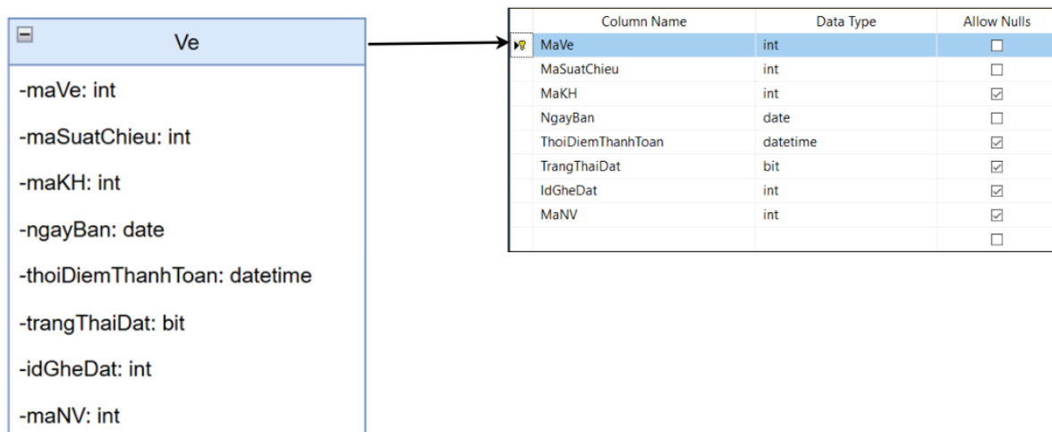
Hình 67. Ảnh xạ thực thể Ve
