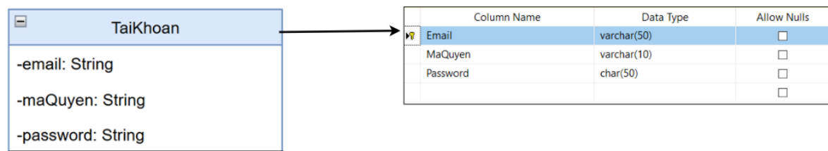
Hình 62. Ảnh xạ thực thể TaiKhoan
