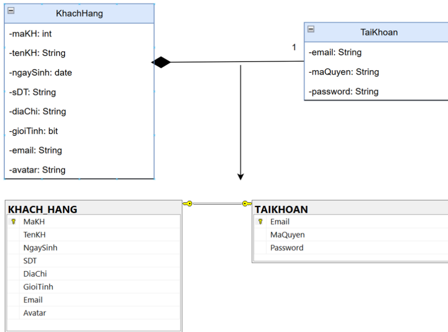
Hình 70. Liên kết thực thể 1-1 KhachHang với TaiKhoan
