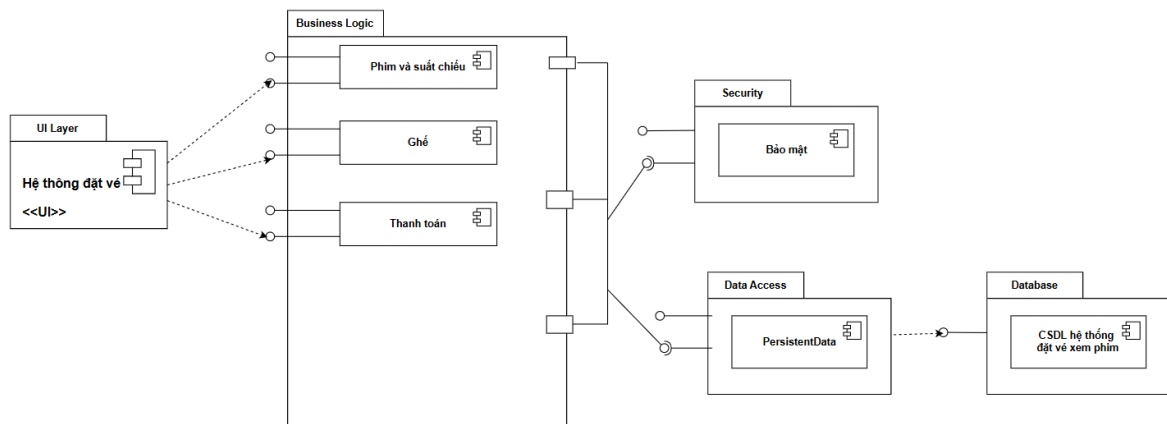
Hình 45. Sơ đồ thành phần theo hệ thống đặt vé
