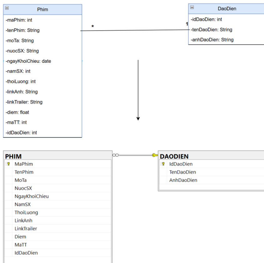
Hình 71. Liên kết thực thể 1-N Phim và DaoDien
