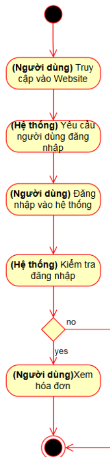
Hình 4. Biểu đồ hoạt động xem hóa đơn khách hàng
