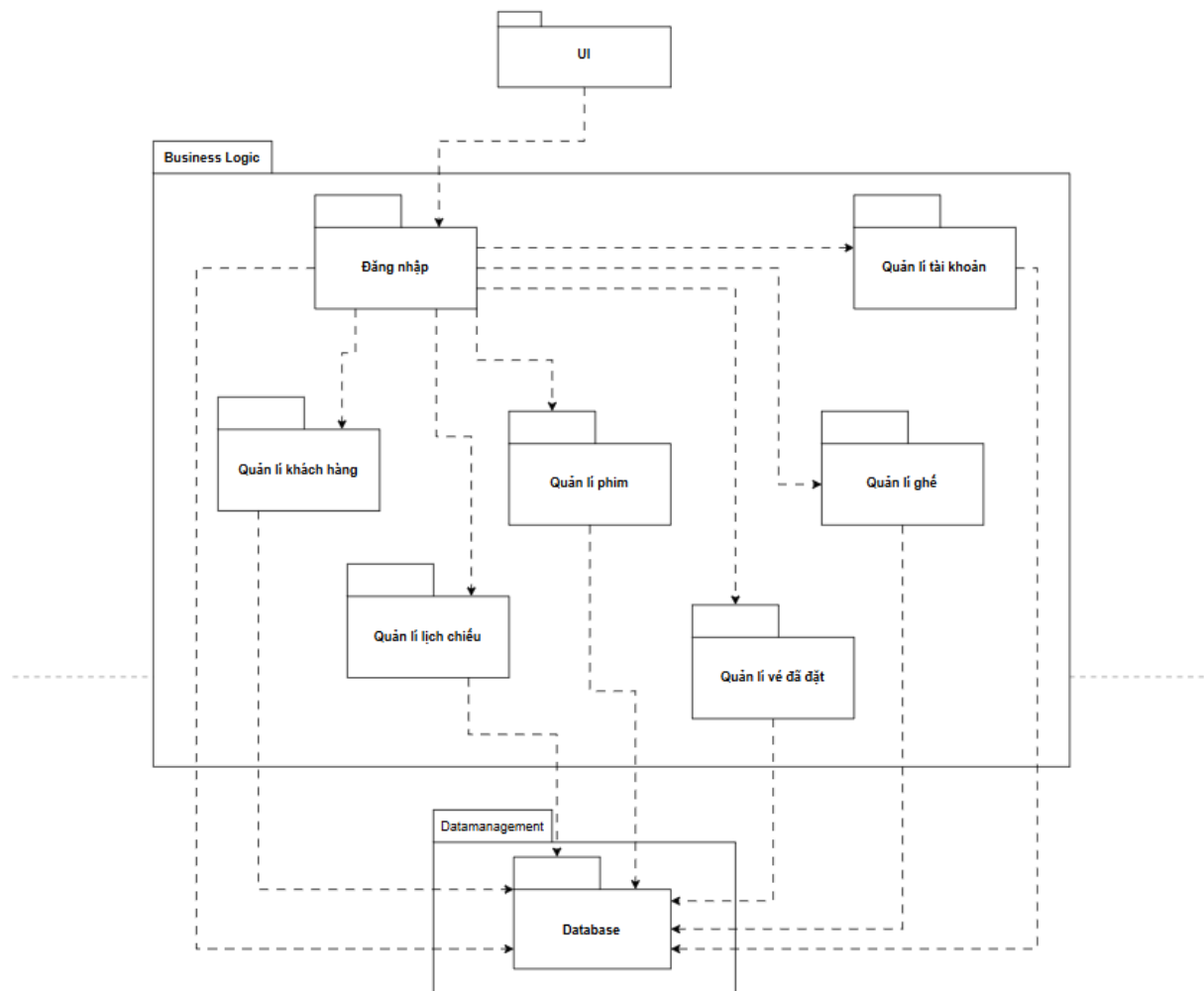
Hình 41. Sơ đồ gói quản lý
