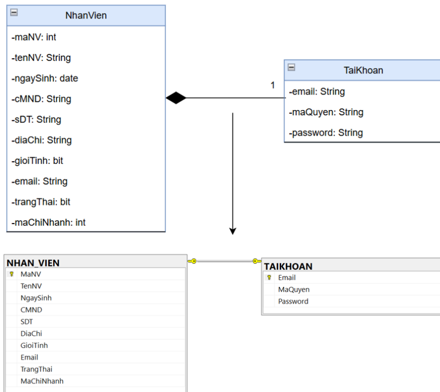
Hình 69. Liên kết thực thể 1-1 NhanVien với TaiKhoan
