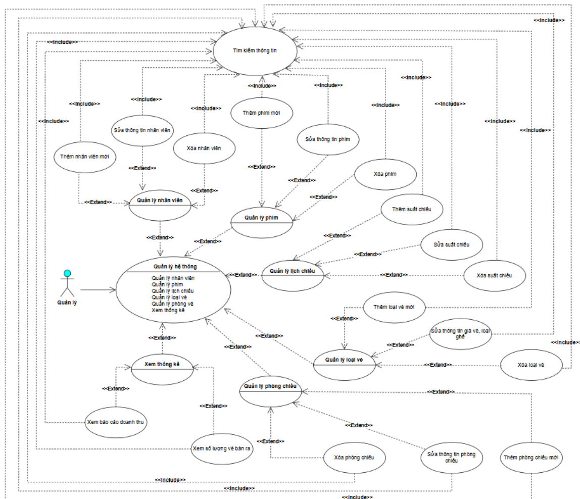
Hình 20. Biểu đồ phân rã ca sử dụng Quản lý hệ thống
