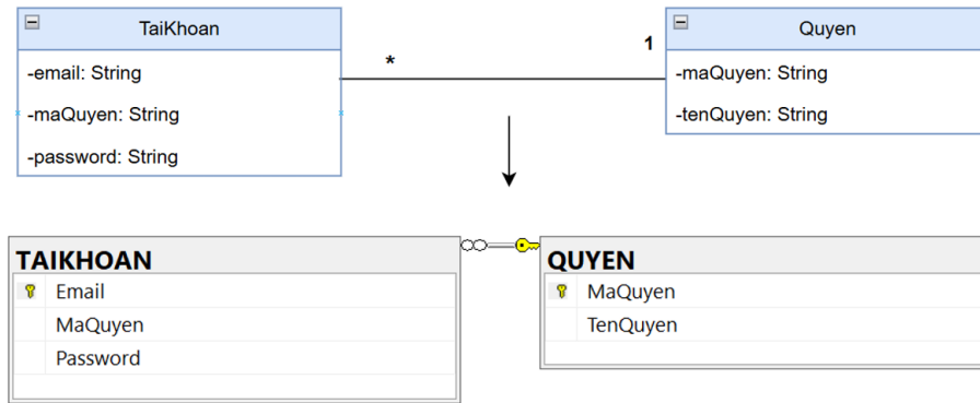
Hình 81. Liên kết thực thể 1-N TaiKhoan và Quyen
