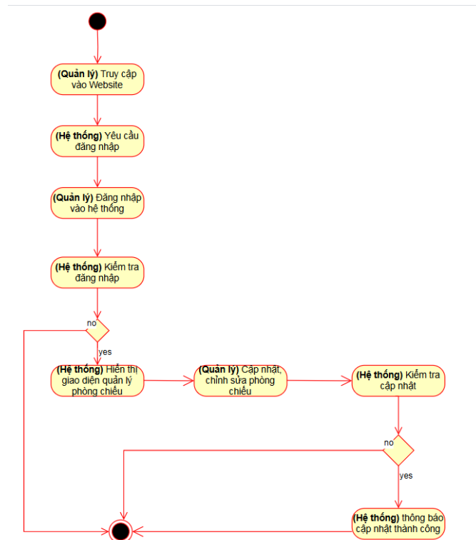
Hình 12. Biểu đồ hoạt động quản lý phòng chiếu
