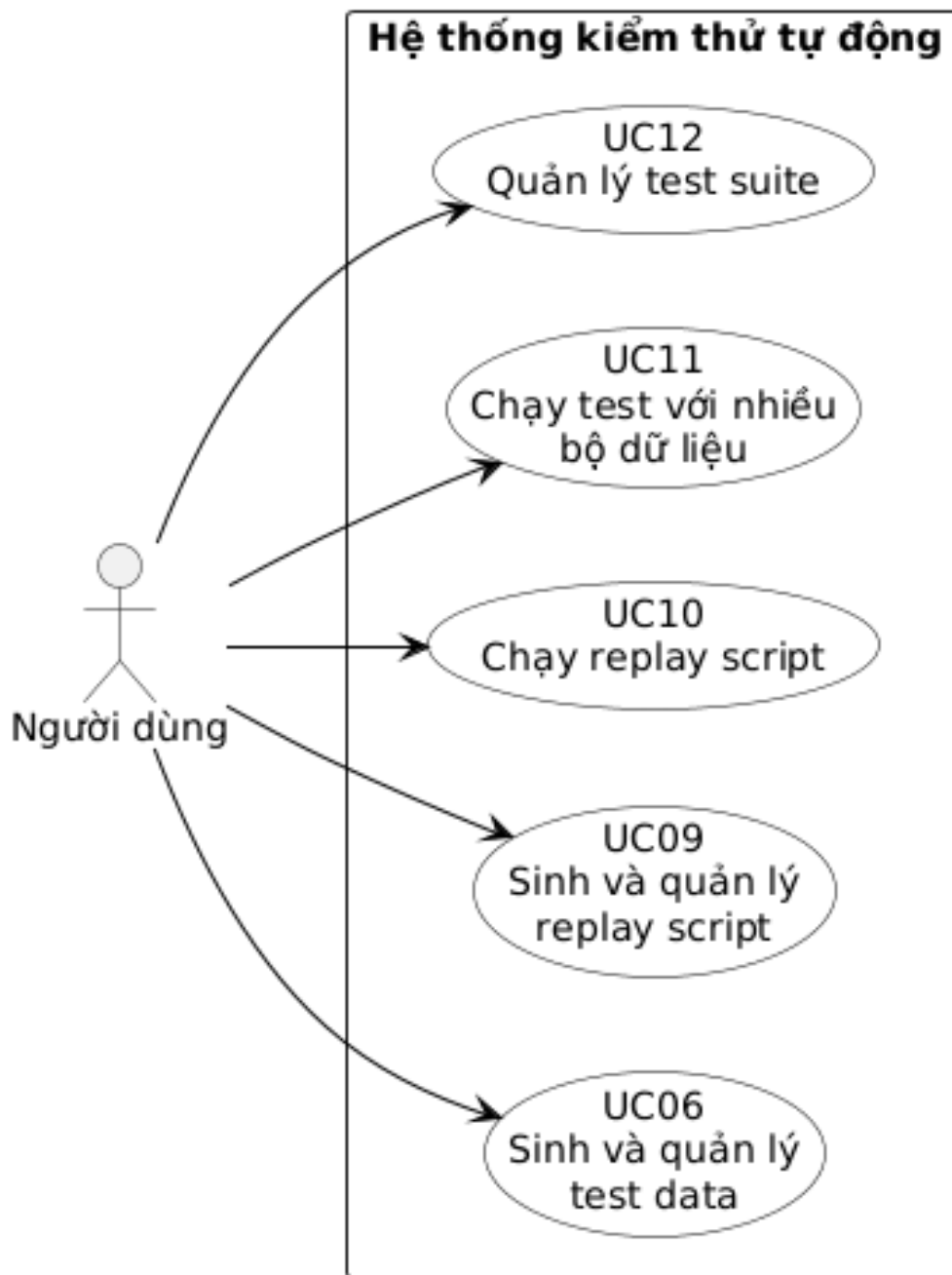
Hình 3.3: Use case replay script, test data và test suite
