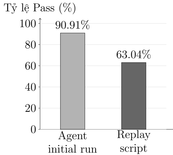
Hình 6.1: So sánh tỷ lệ Pass giữa Agent và Replay Script
