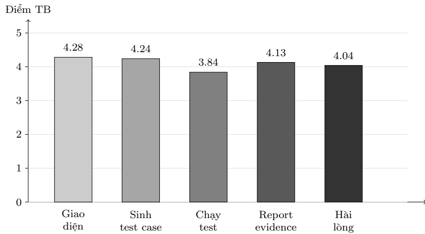
Hình 6.2: Điểm trung bình khảo sát theo nhóm tiêu chí
