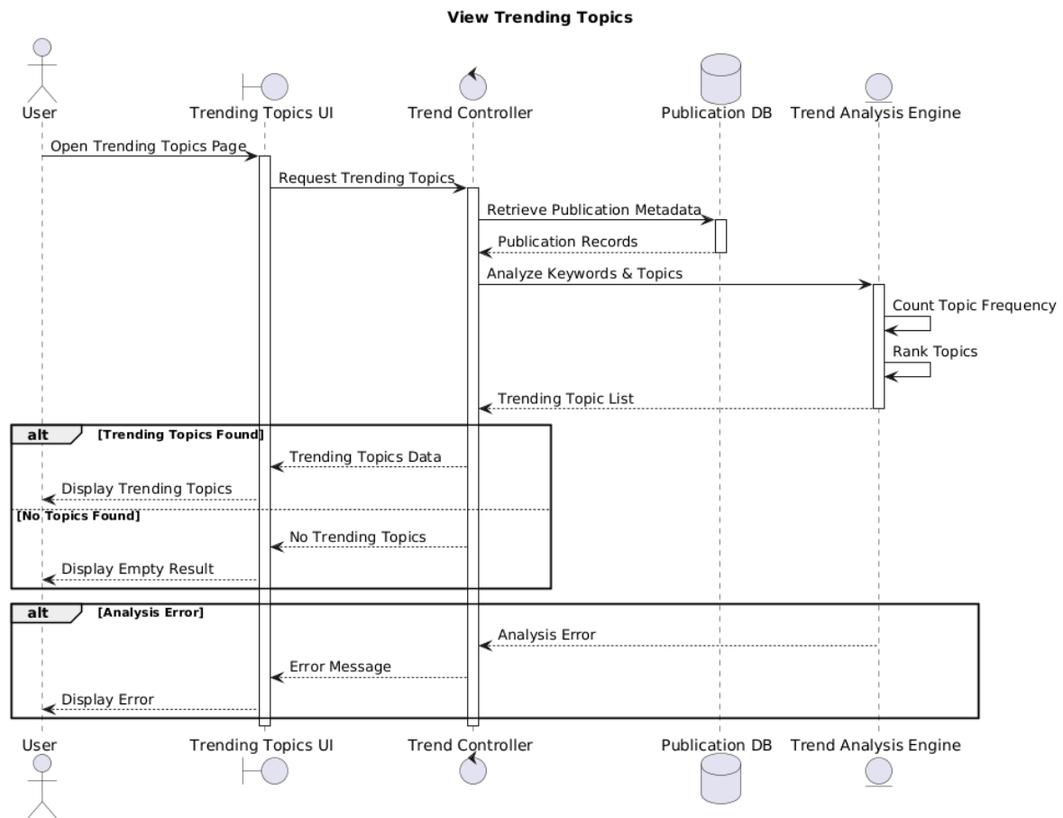
Hình 41: Sequence diagram
