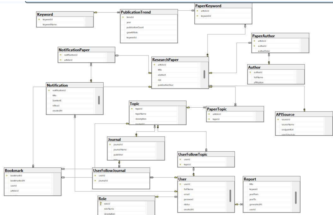
Hình 7: Database Design
