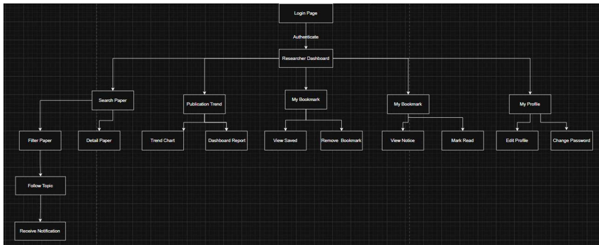
Hình 4: Screen Description
