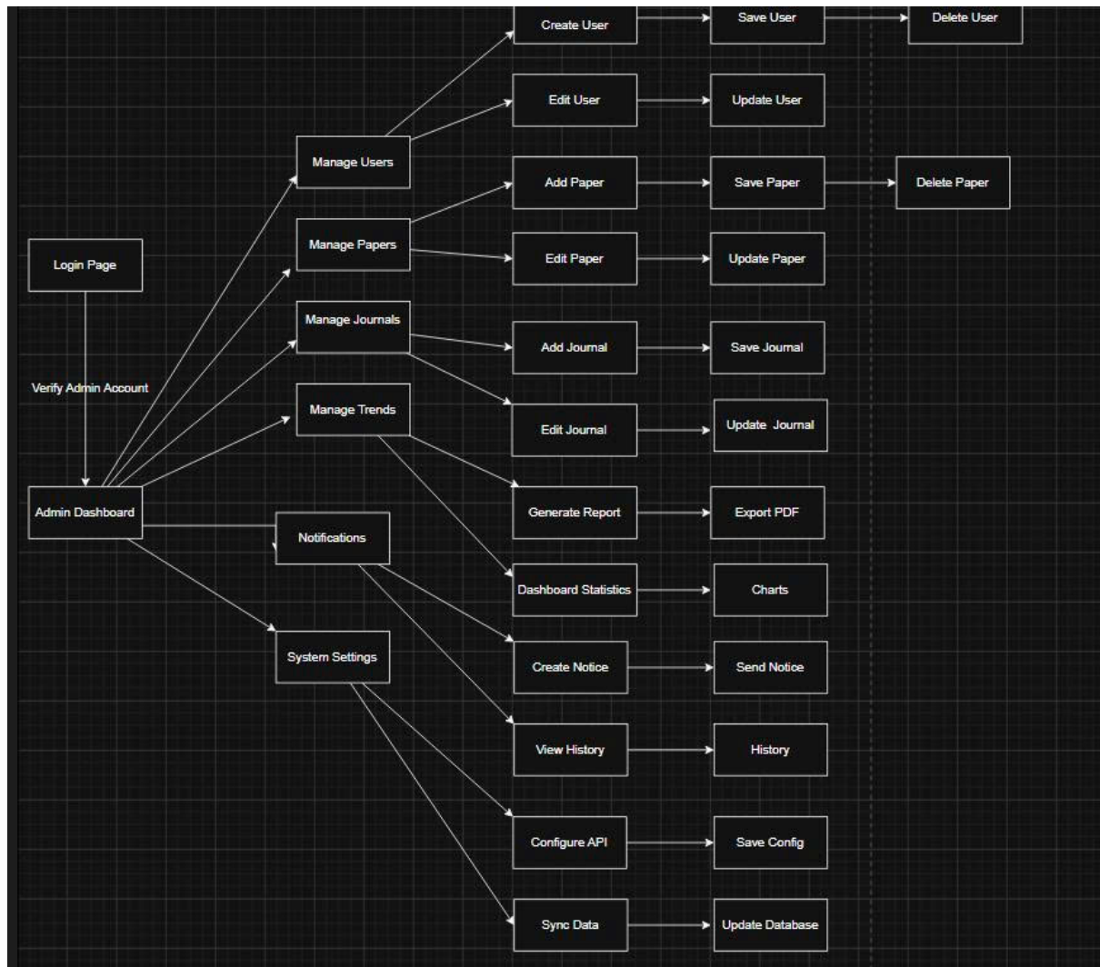
Hình 3: Screens Flow
