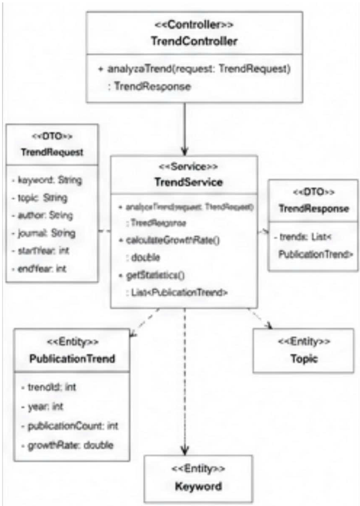
Hình 2: Class Diagram: Track Publication Trends
