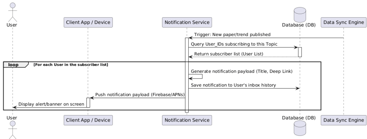
Hình 80: Sequence diagram
