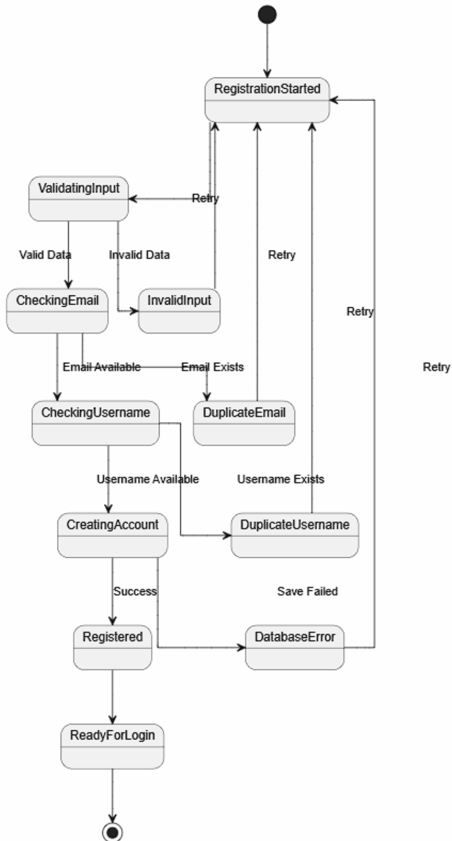
Hình 43: State diagram
