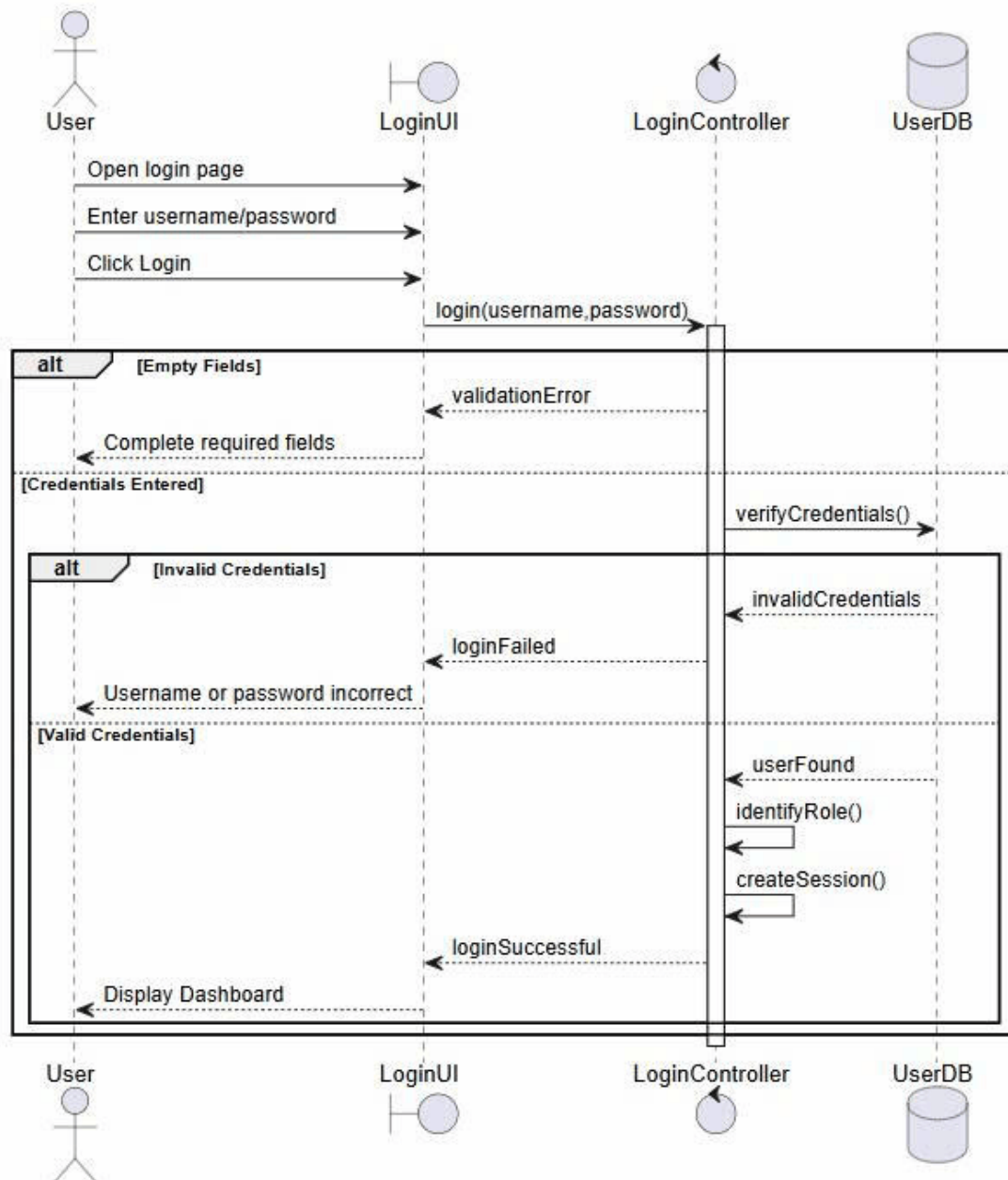
Hình 46: Sequence Diagram
