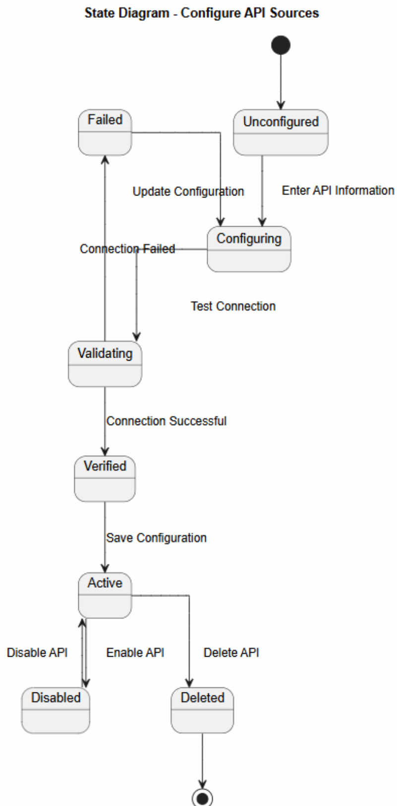
Hình 87: State diagram
