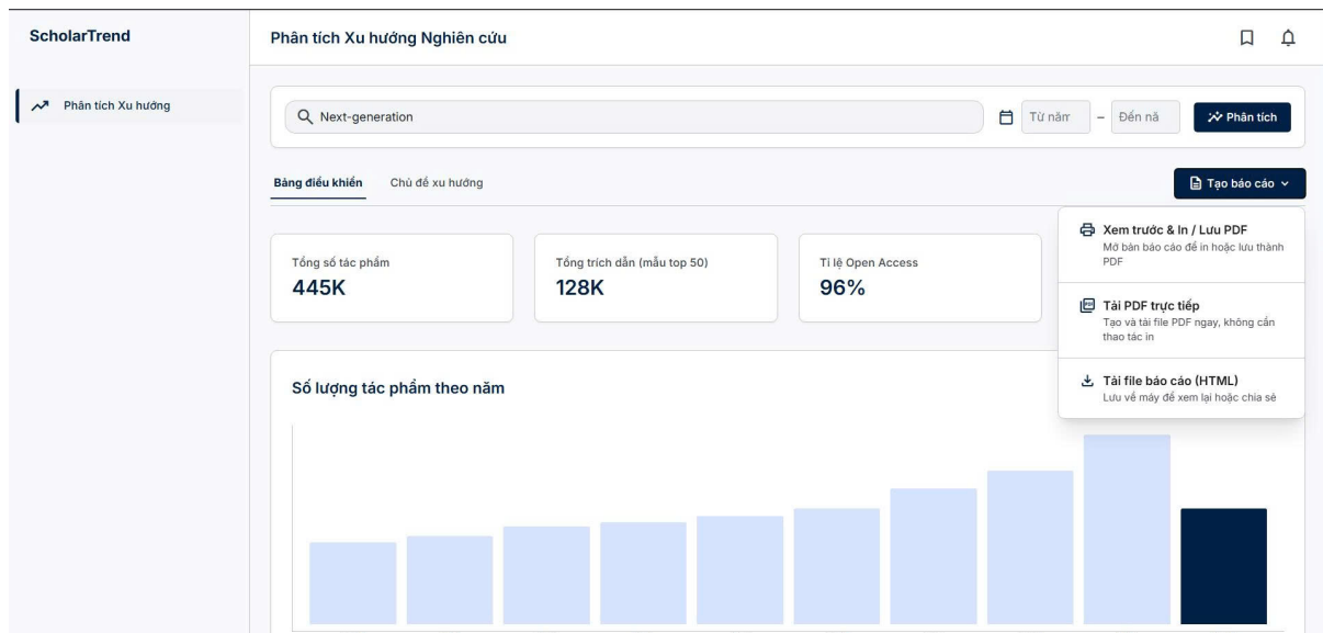
Hình 34: Generate Report
