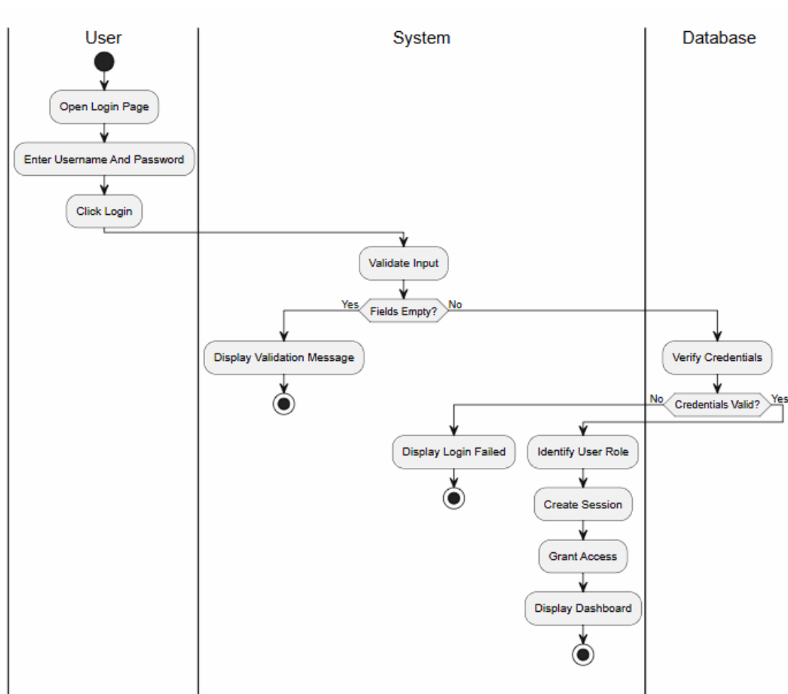
Hình 45: Activity diagram
