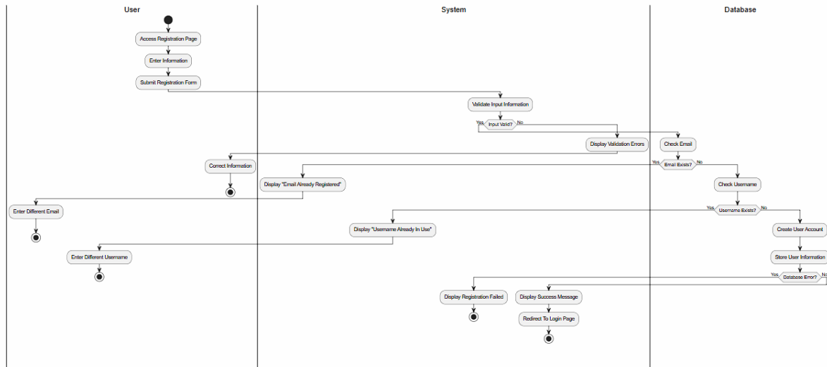
Hình 41: Activity diagram
