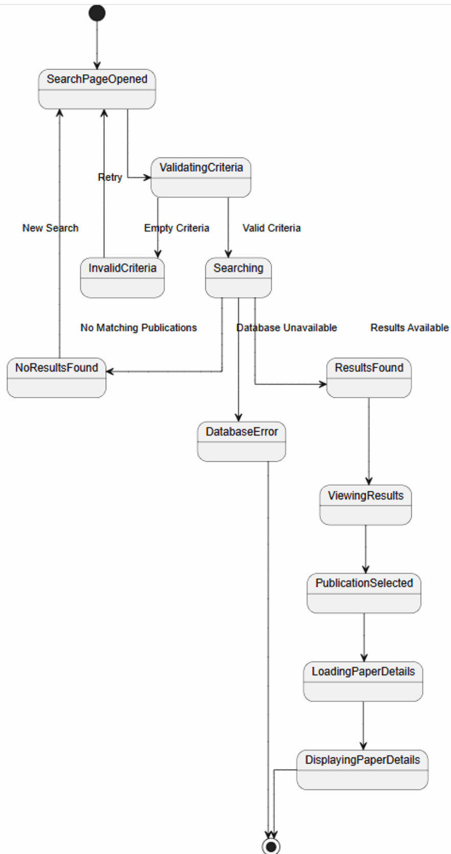
Hình 51: State diagram
