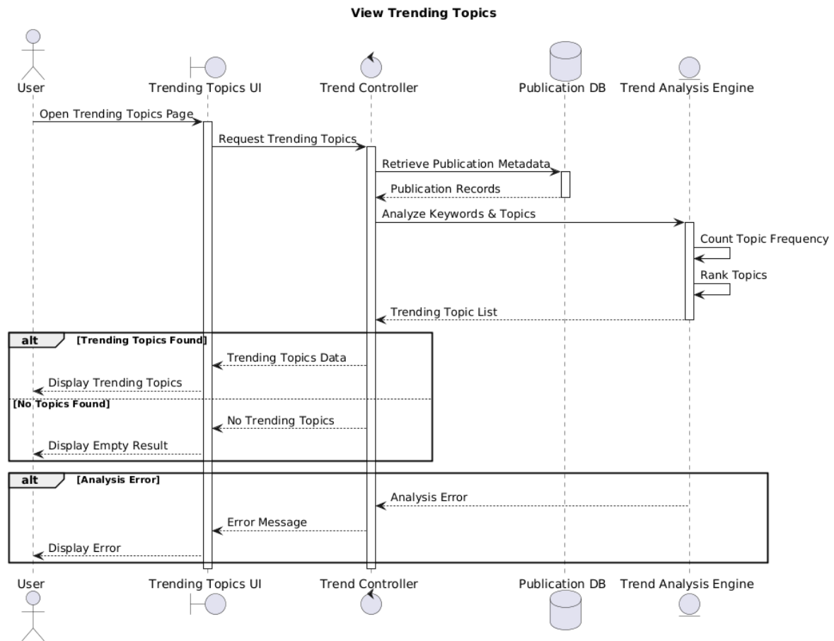
Hình 74: Sequence diagram
