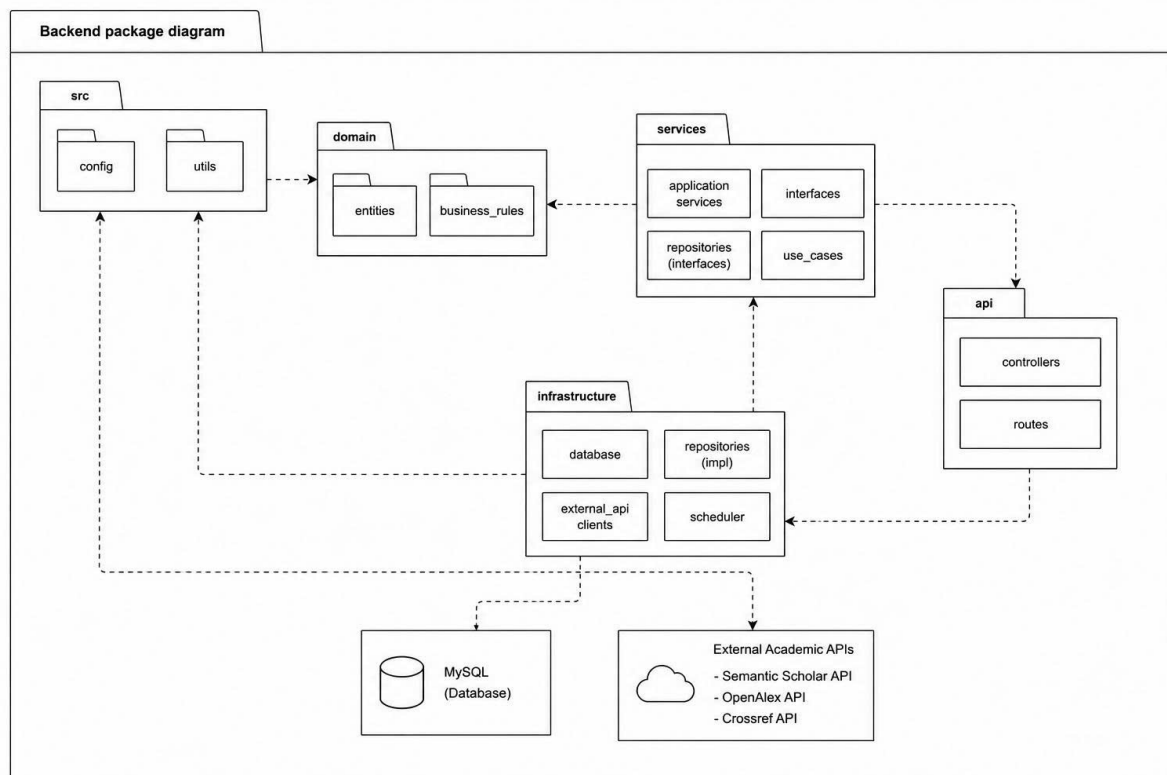
Hình 41: Backend package diagram
