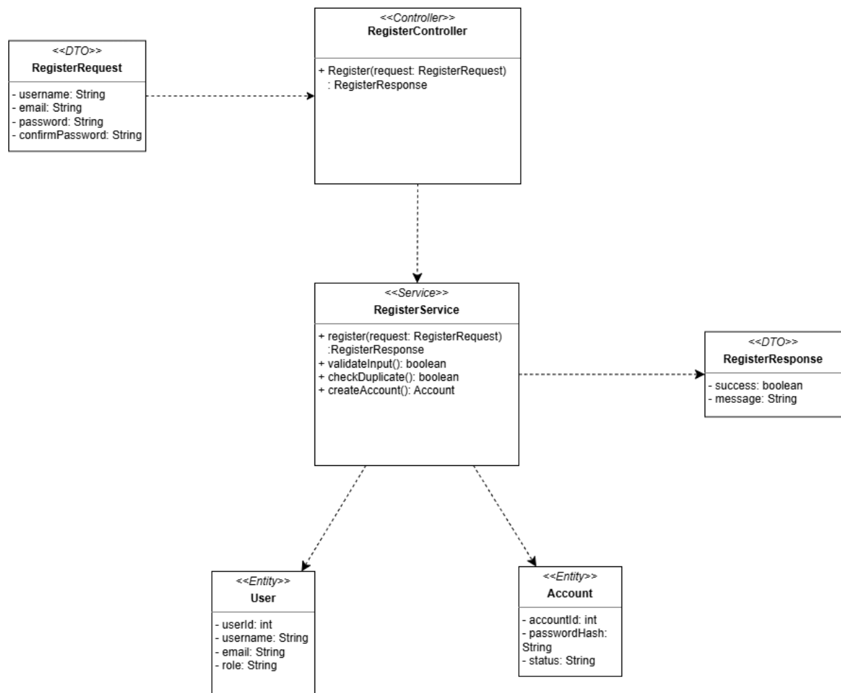
Hình 46: Class Diagram: Register
