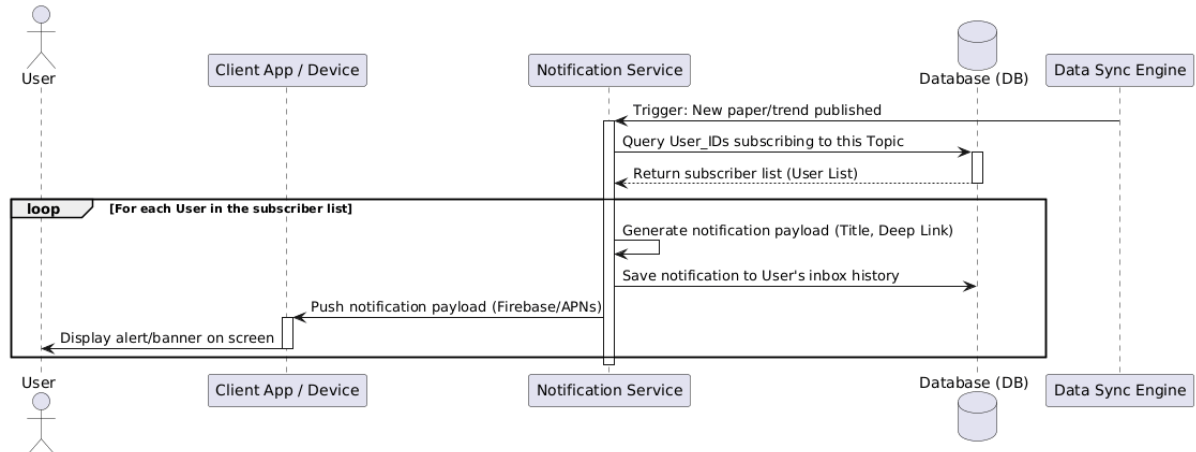
Hình 82: Sequence diagram
