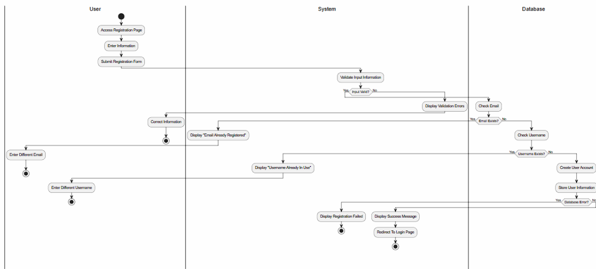
Hình 13: Activity diagram
