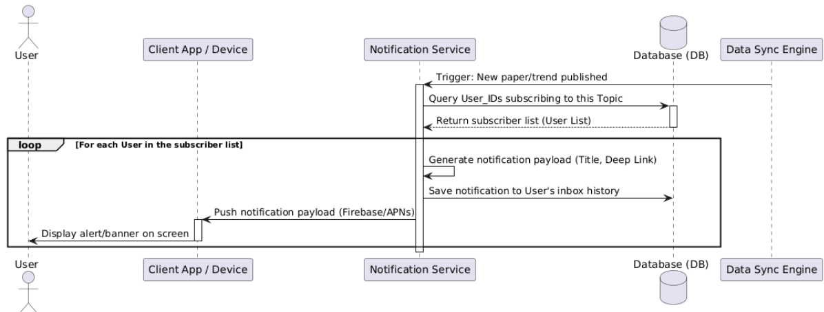
Hình 82: Sequence diagram
