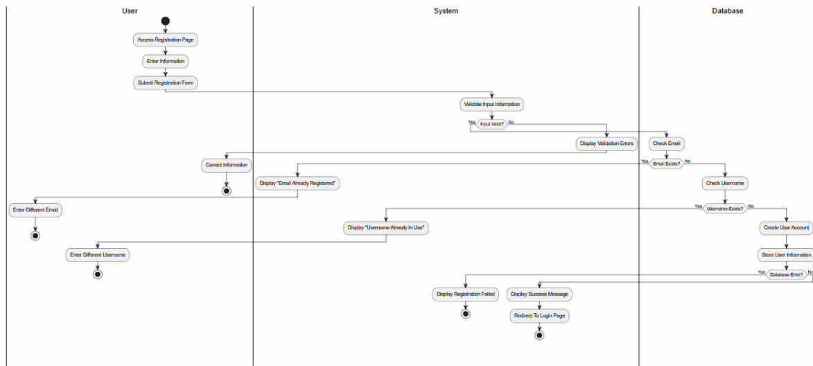
Hình 13: Activity diagram
