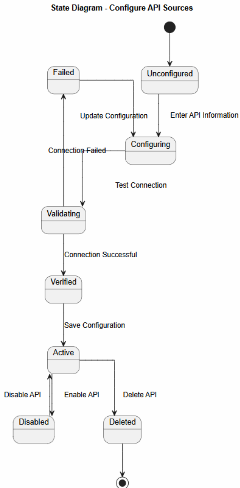
Hình 76: State diagram
