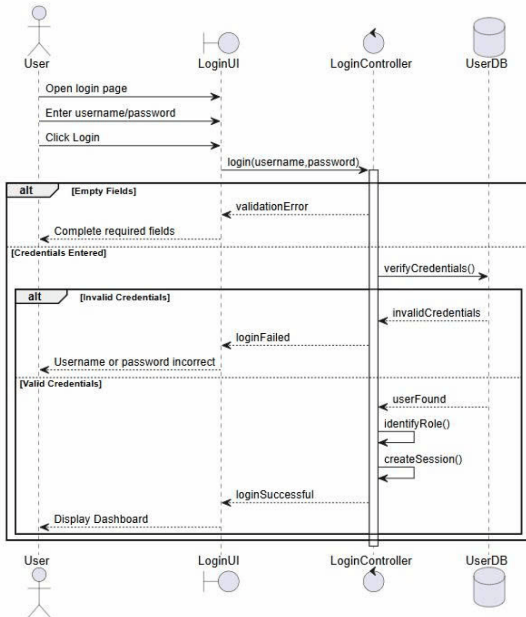
Hình 35: Sequence Diagram
