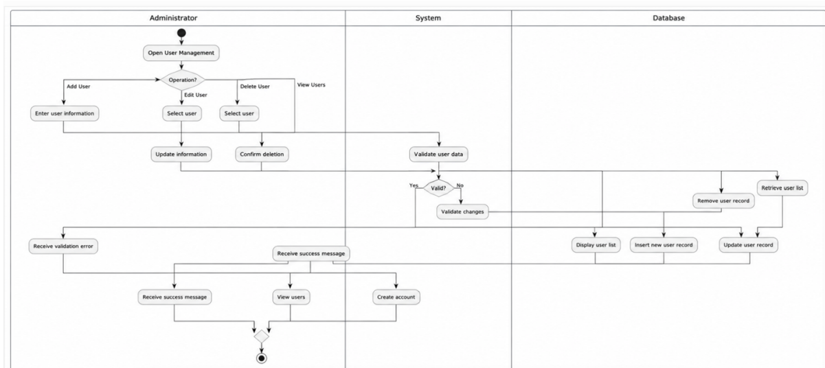
Hình 57: Activity Diagram - Manage Users
