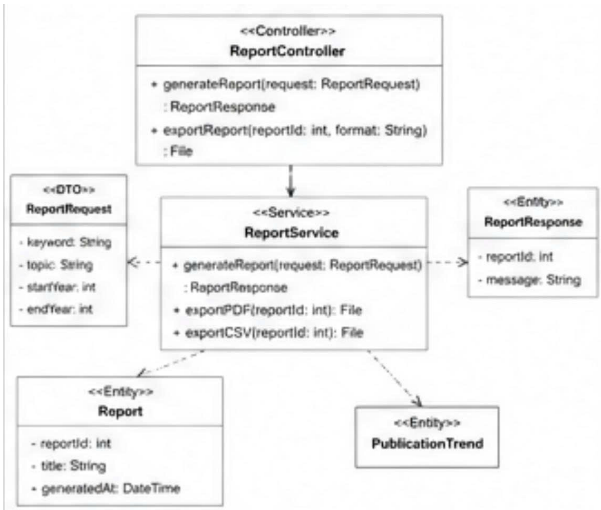
Hình 6: Class Diagram - Generate Reports
