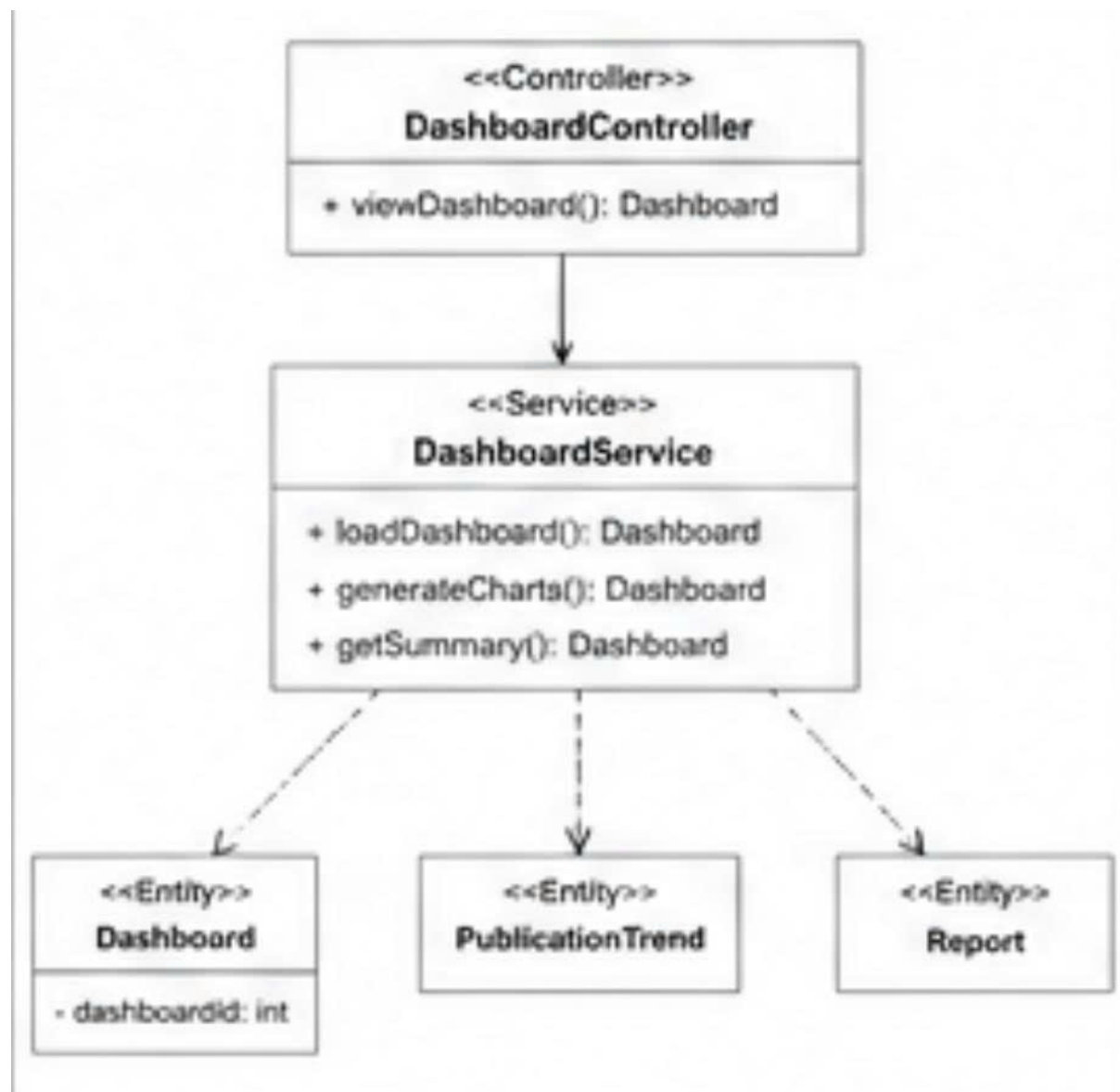
Hình 5: Class Diagram: View Dashboard
