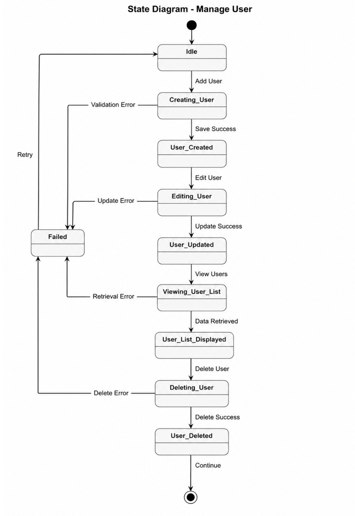
Hình 62: State diagram - Manage Users
