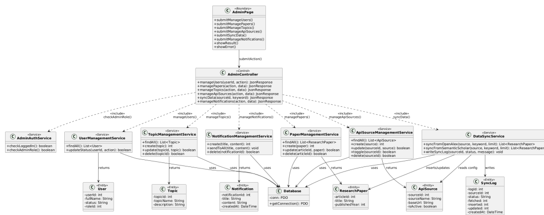
Hình 86: Class Diagram
