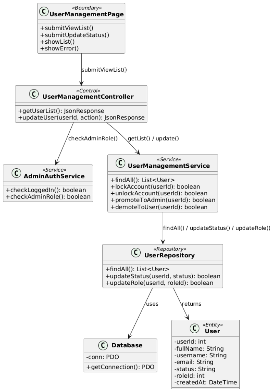
Hình 90: Class Diagram
