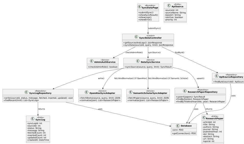
Hình 98: Class Diagram
