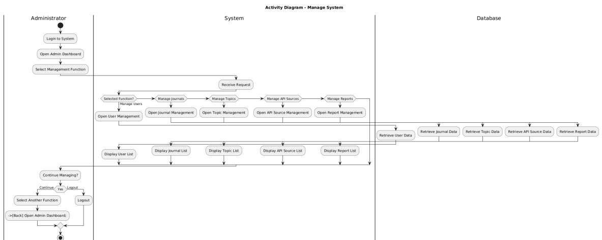
Hình 84: Activity diagram
