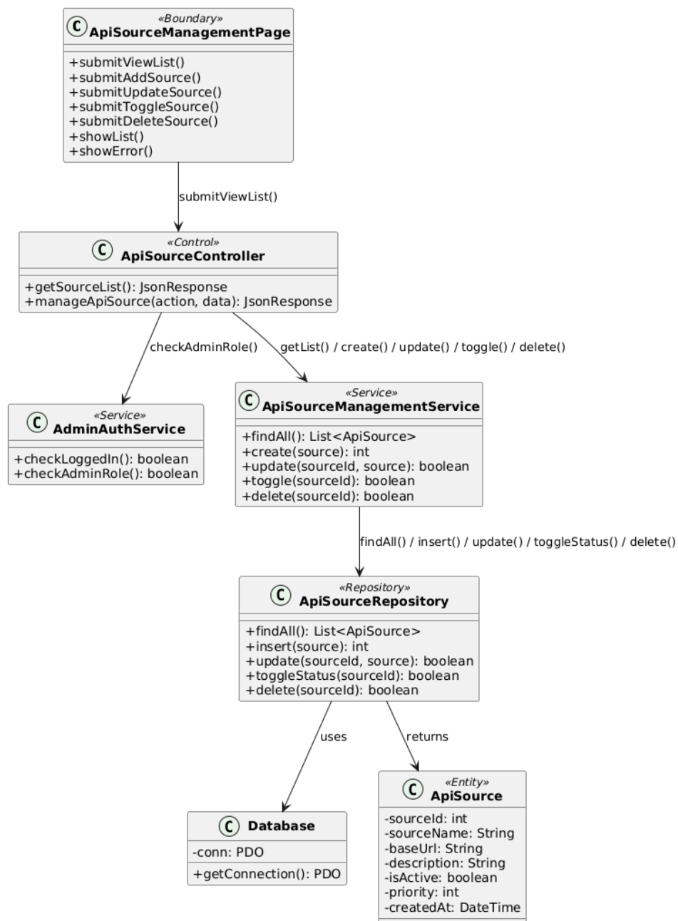
Hình 94: Class Diagram
