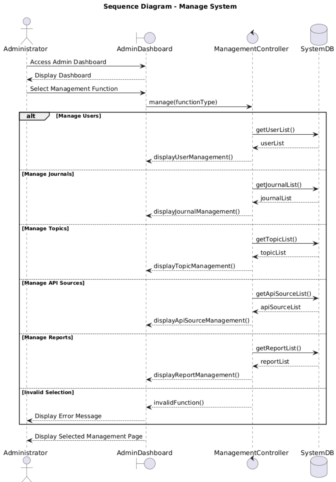
Hình 85: Sequence diagram
