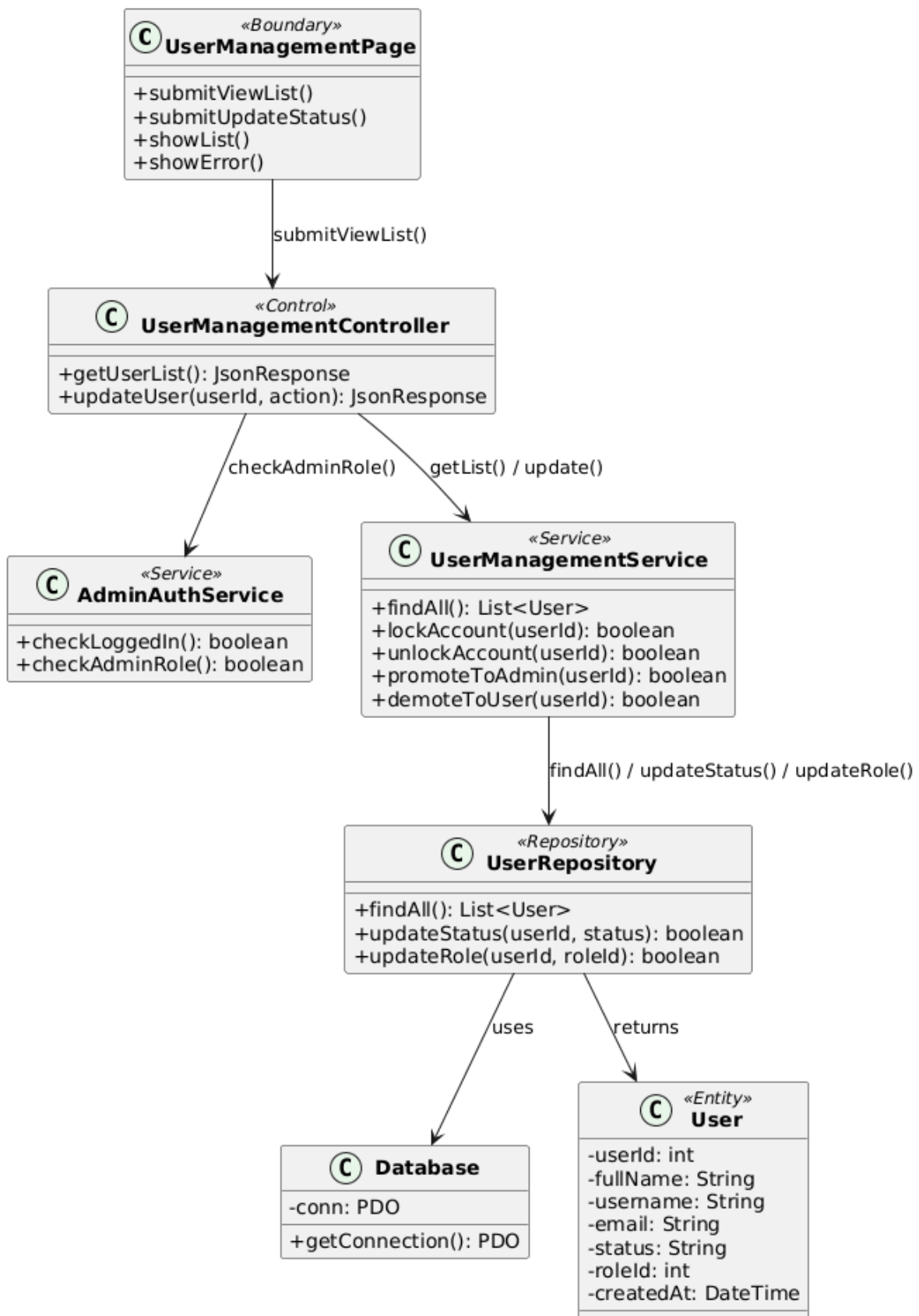
Hình 90: Class Diagram
